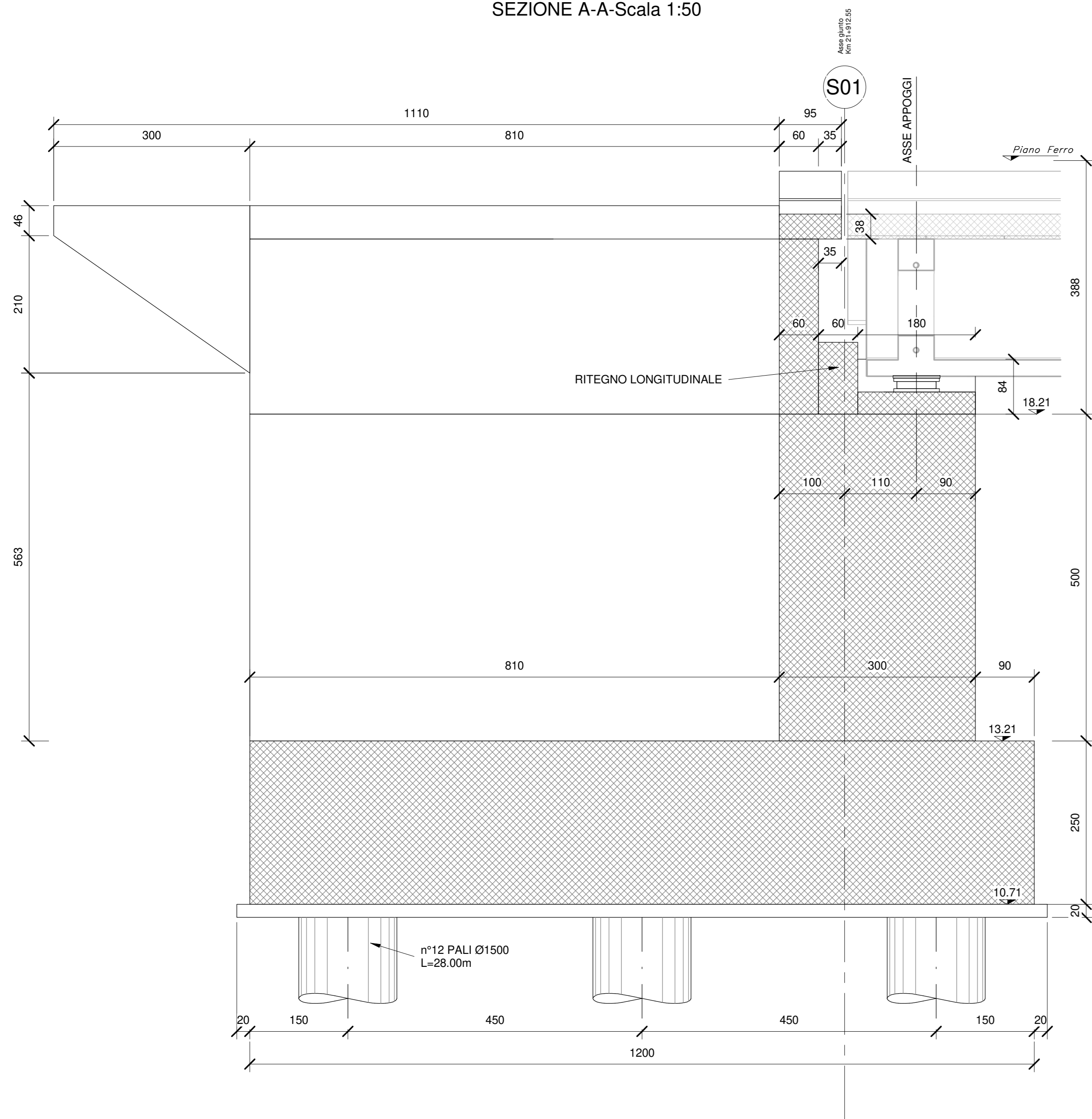
SEZIONE A-A-Scala 1:50
