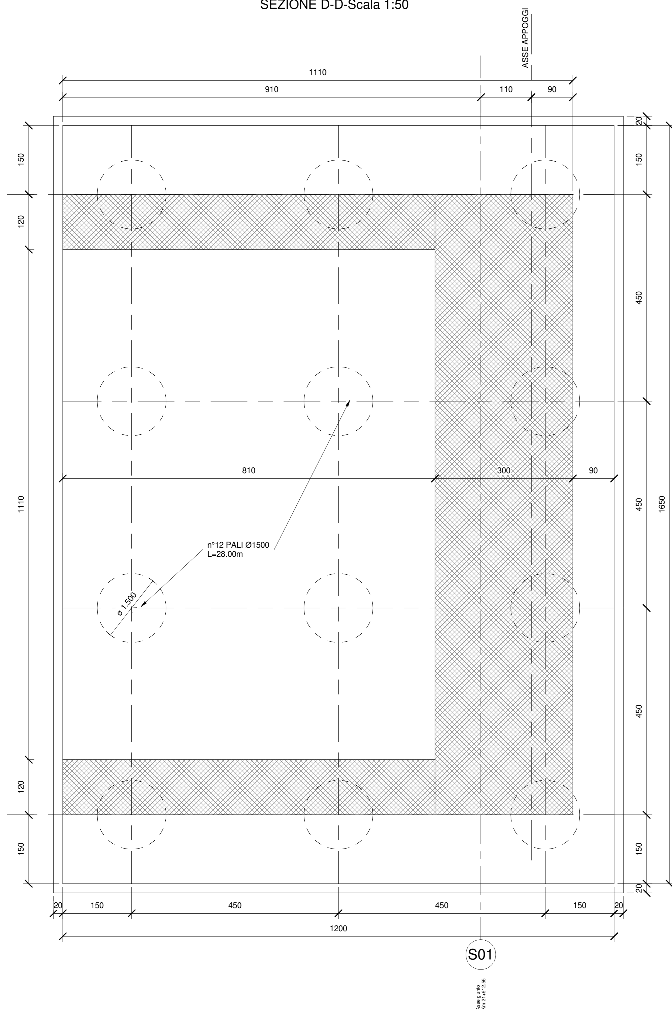
SEZIONE D-D-Scala 1:50
