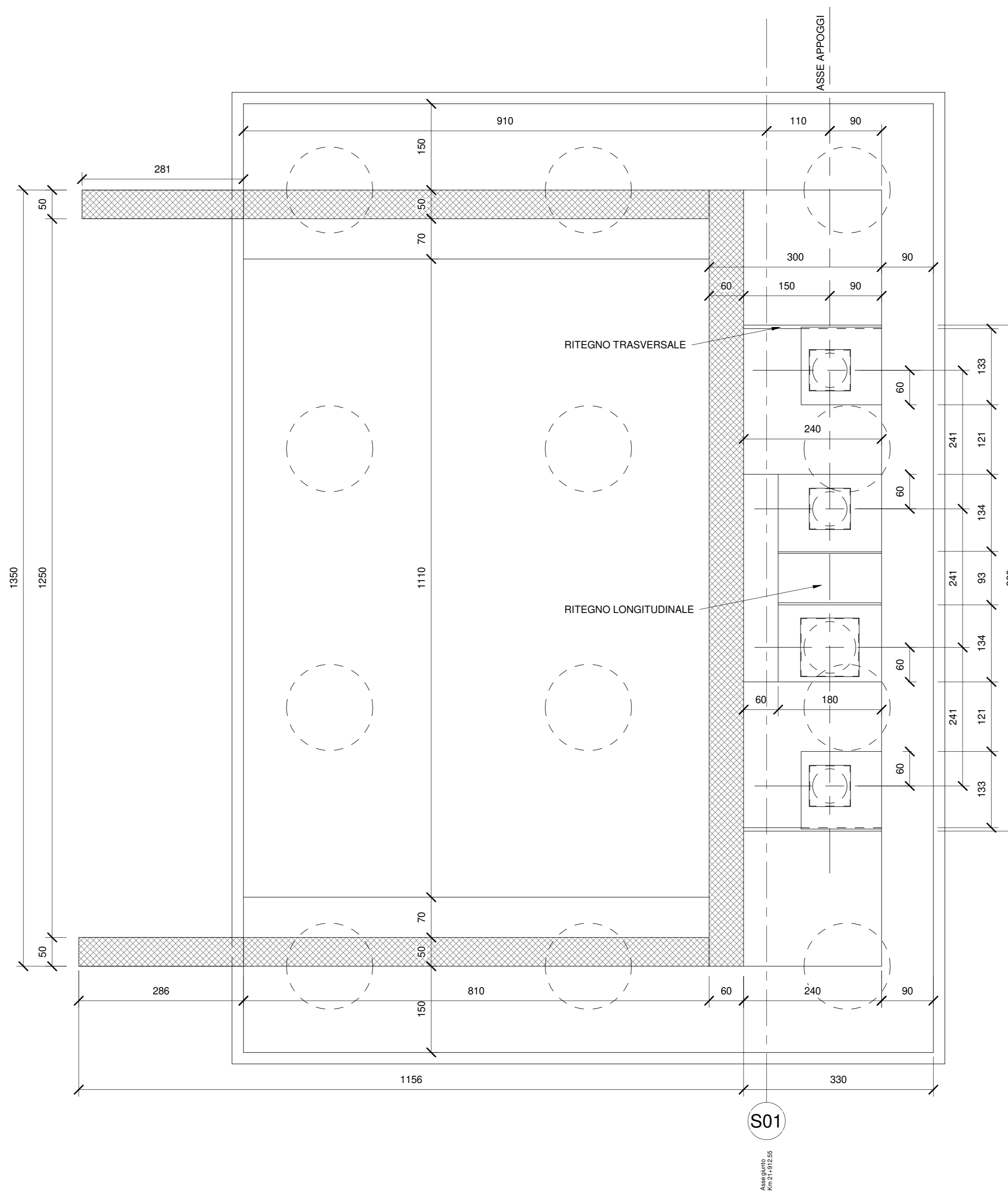
SEZIONE E-E-Scala 1:50
