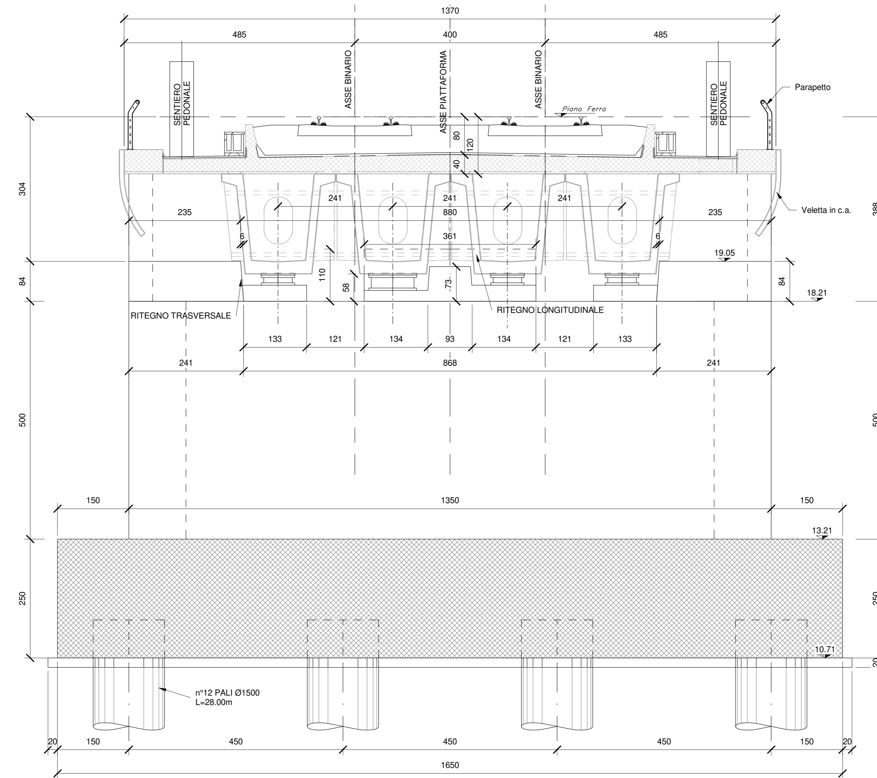
SEZIONE B-B-Scala 1:50
