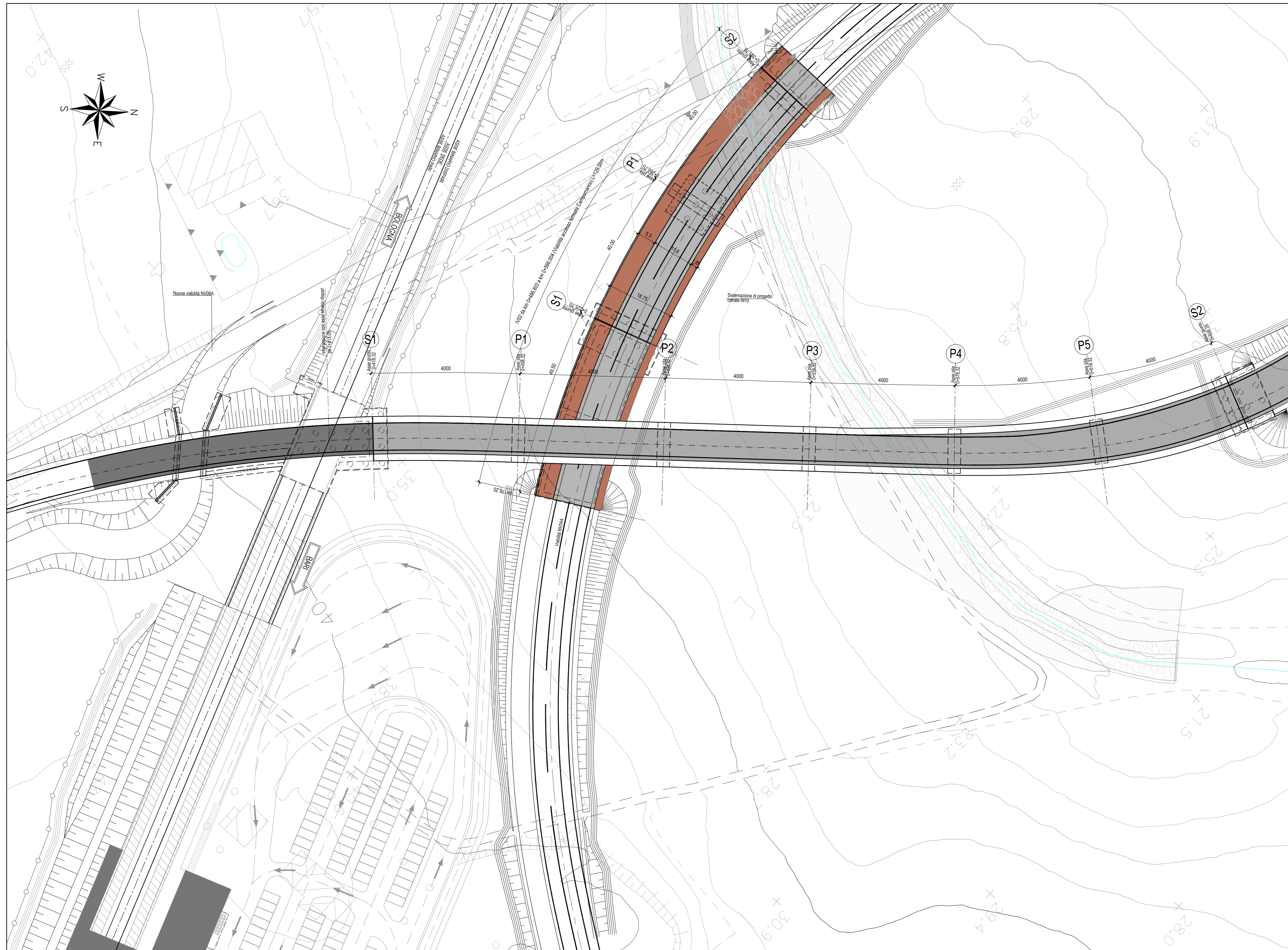
PLANIMETRIA DI PROGETTO - Scala 1:500
