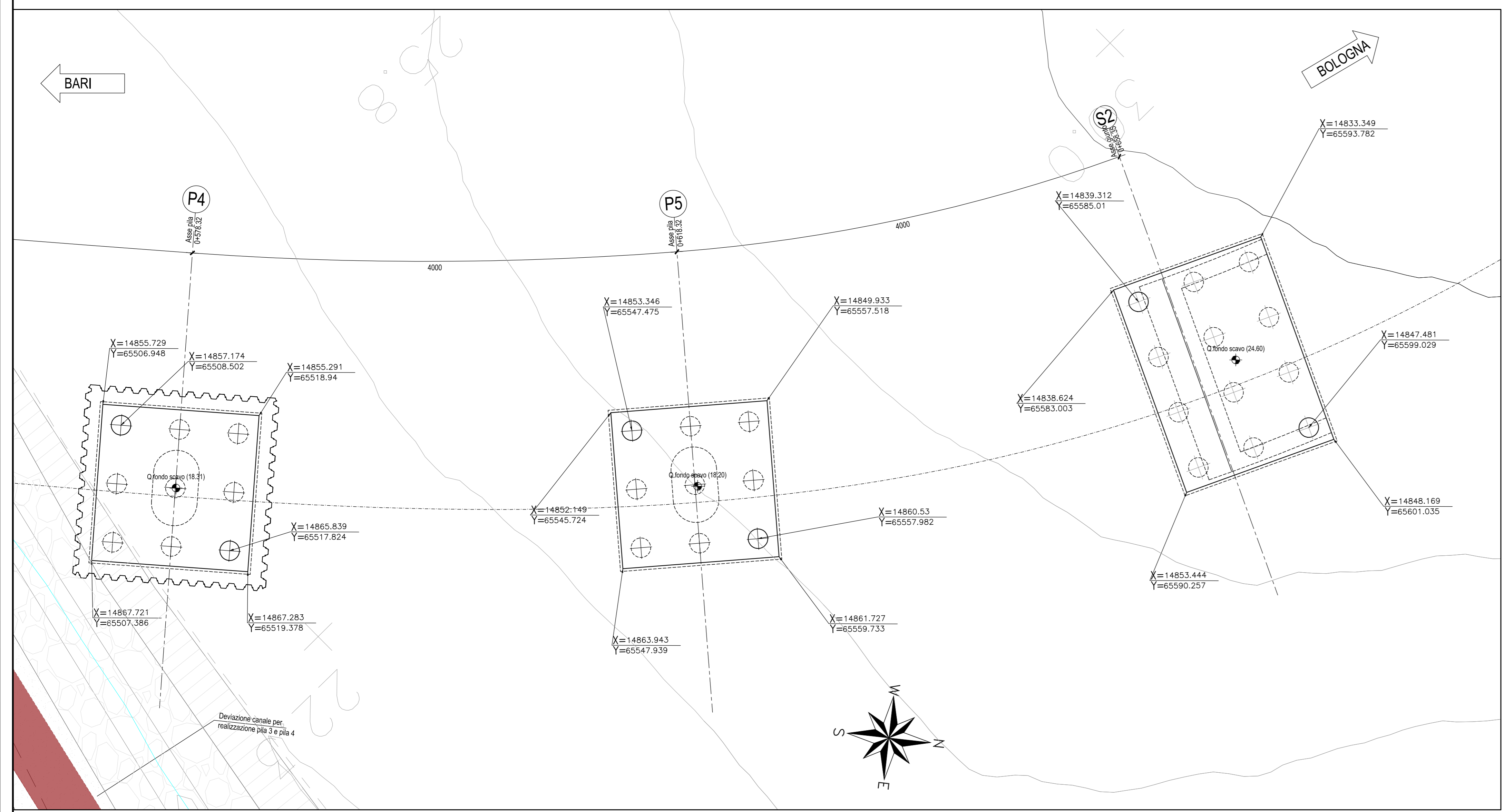
PLANIMETRIA DI TRACCIAMENTO-Scala 1:200
