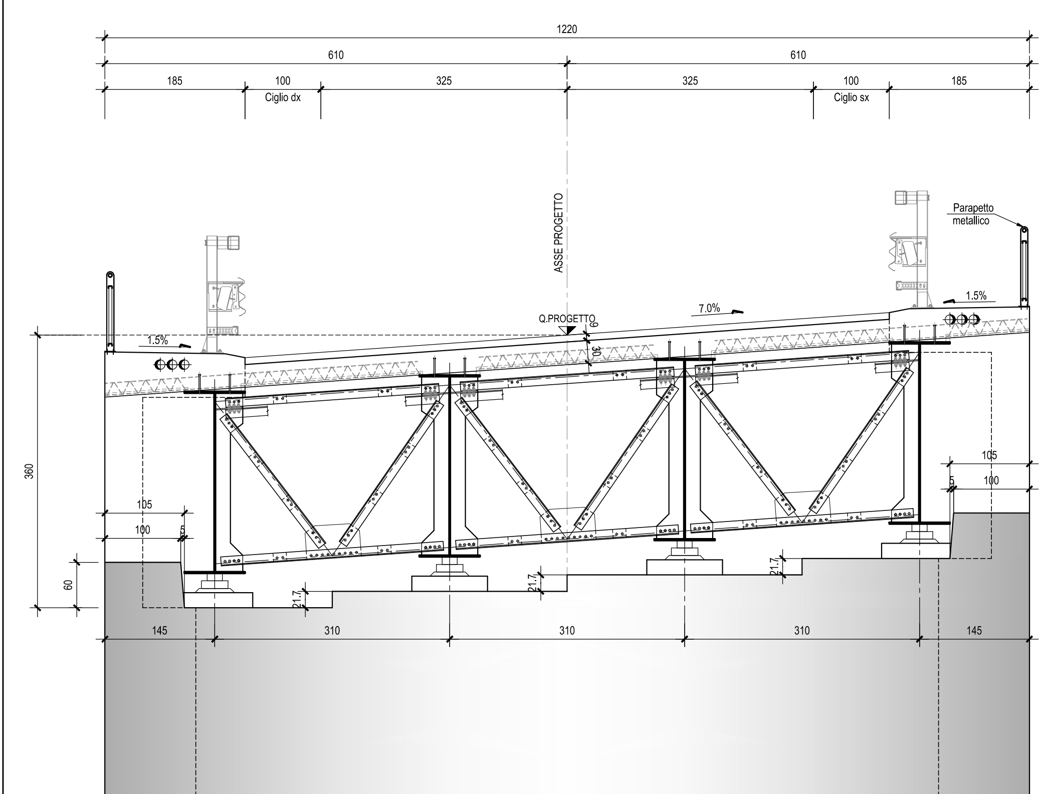
PROSPETTO TIPO APPOGGIO-Scala 1:50 (SPALLA S1)
