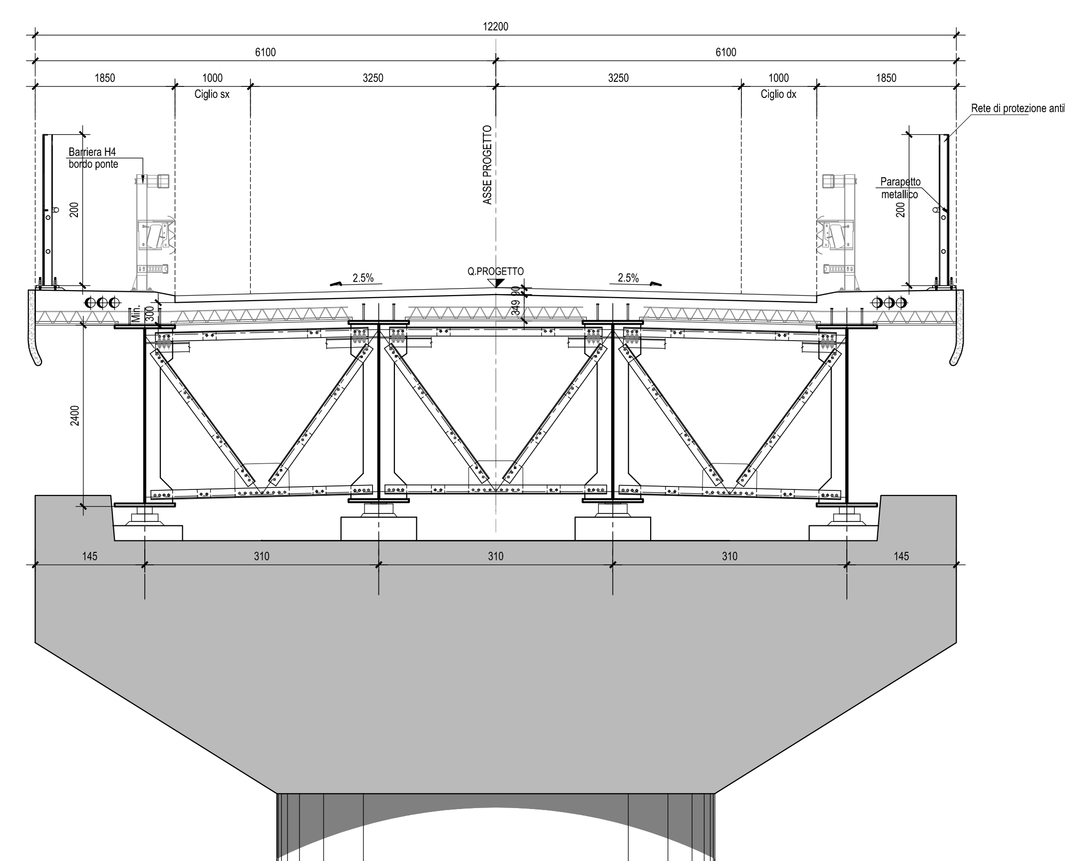
PROSPETTO TIPO APPOGGIO-Scala 1:50 (PILA)
