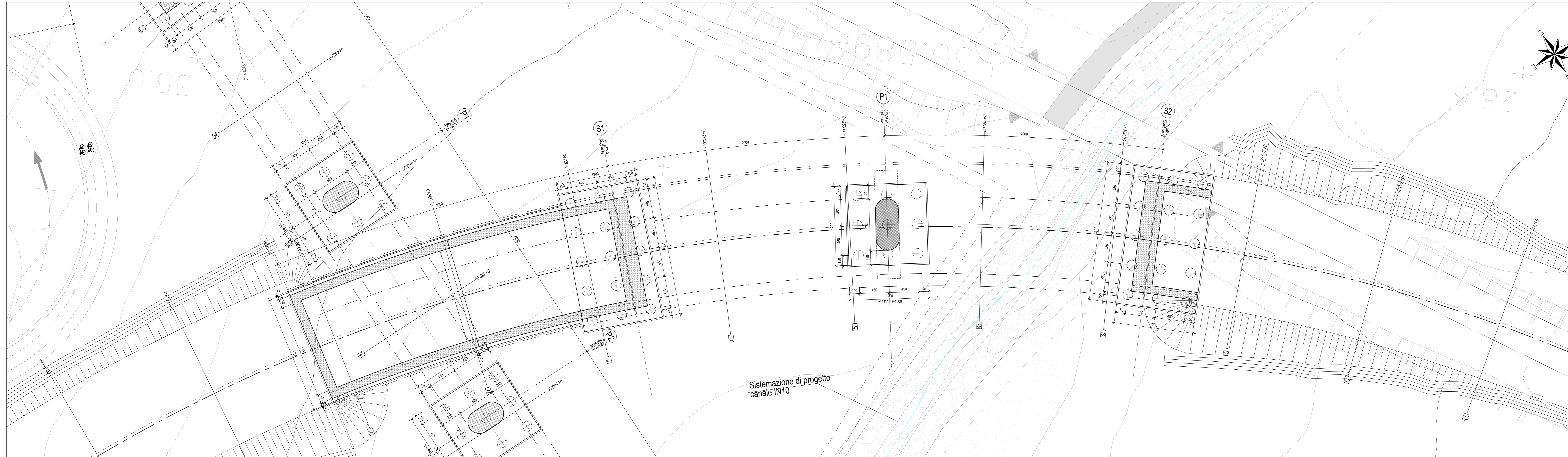
PIANTA FONDAZIONI-Scala 1:200
