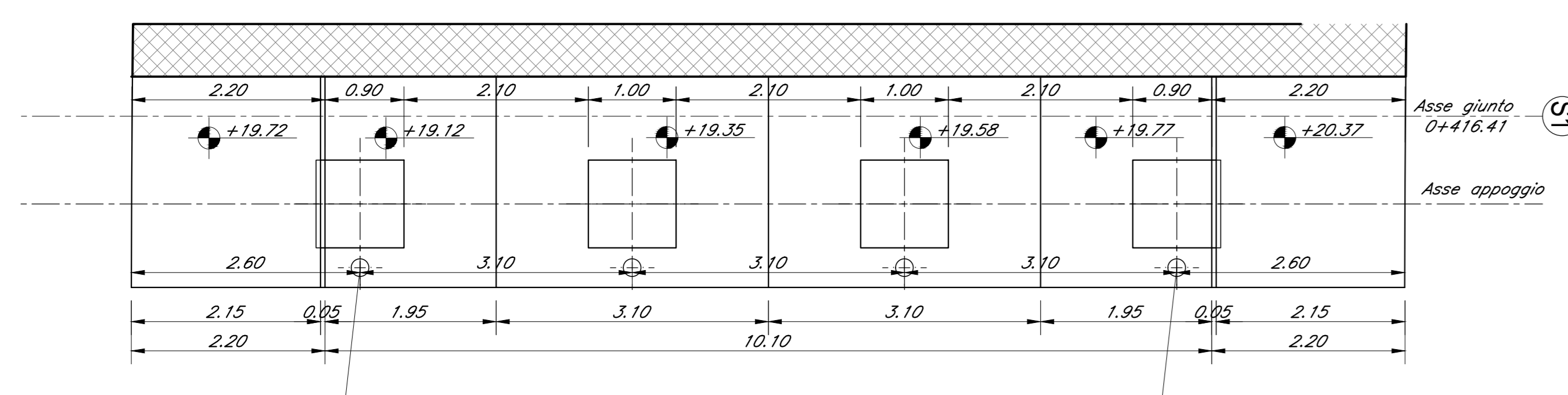
SEZIONE D-D - Scala 1:50
