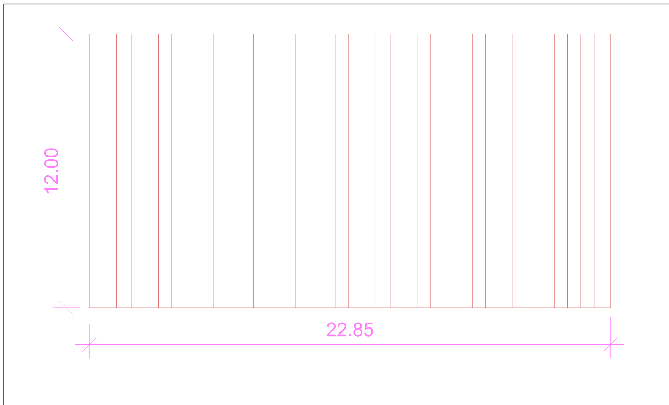
② Carpenteria Palancola tipo 2 1 : 100
