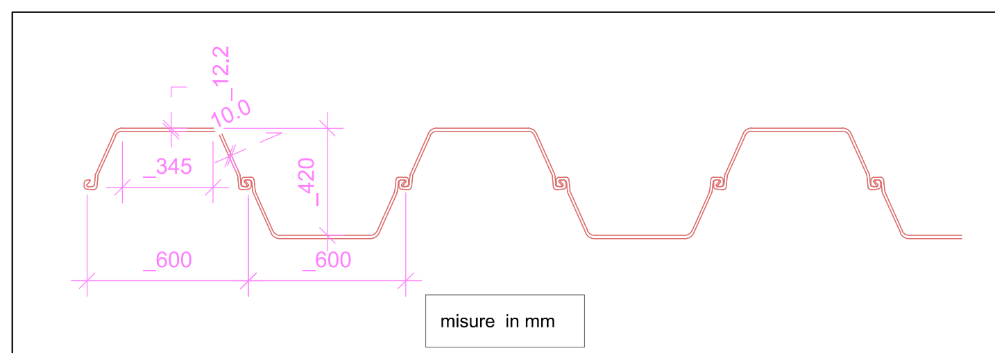
① particolare palancola 1 : 20
