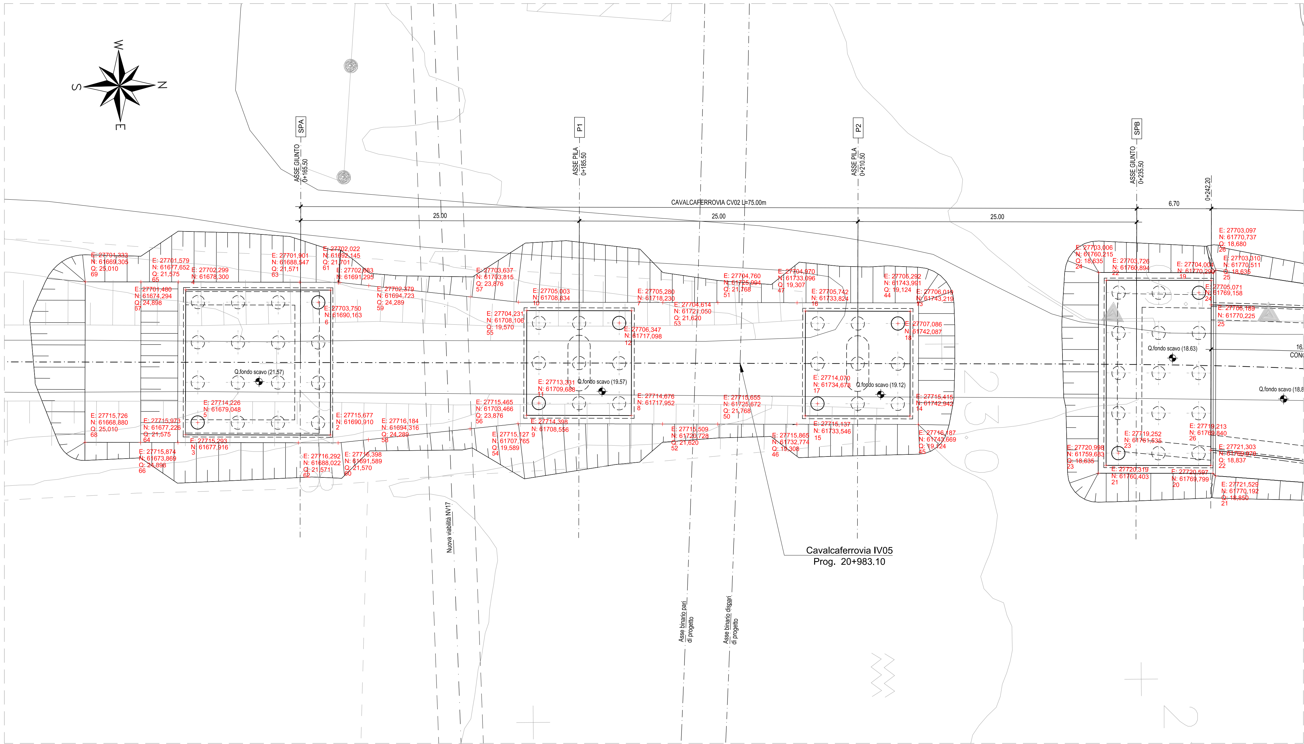
PLANIMETRIA DI TRACCIAMENTO - Scala 1:200
