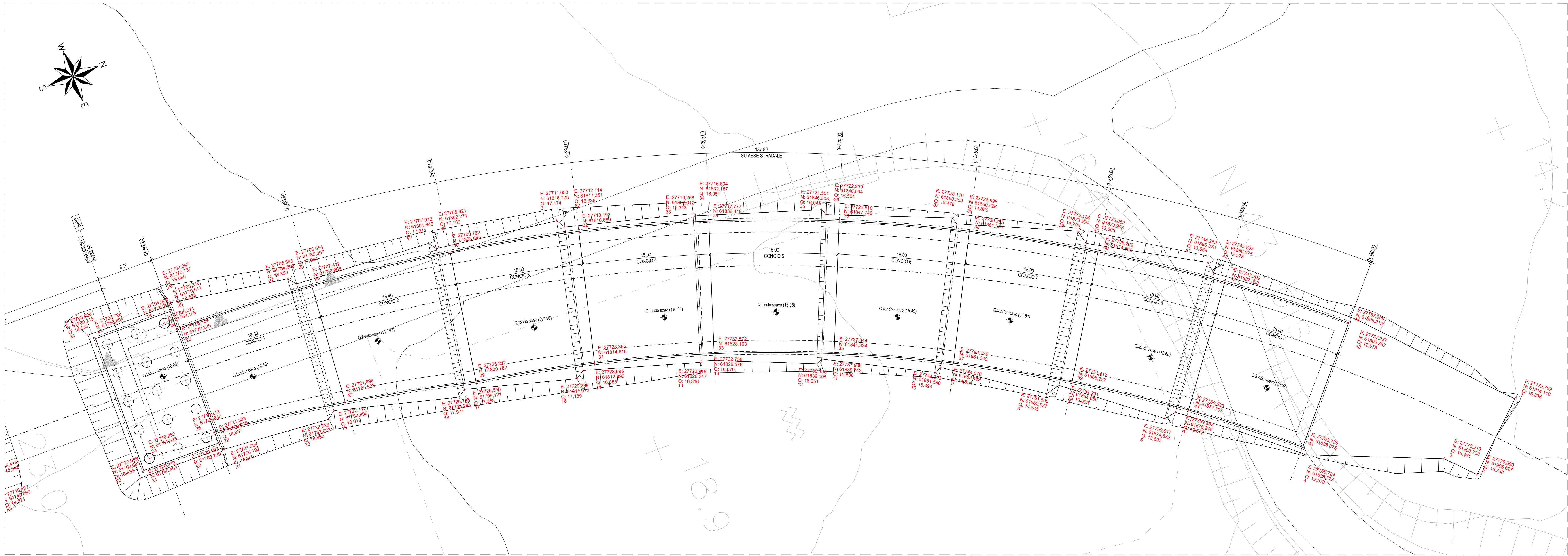
PLANIMETRIA DI TRACCIAMENTO - Scala 1:200
