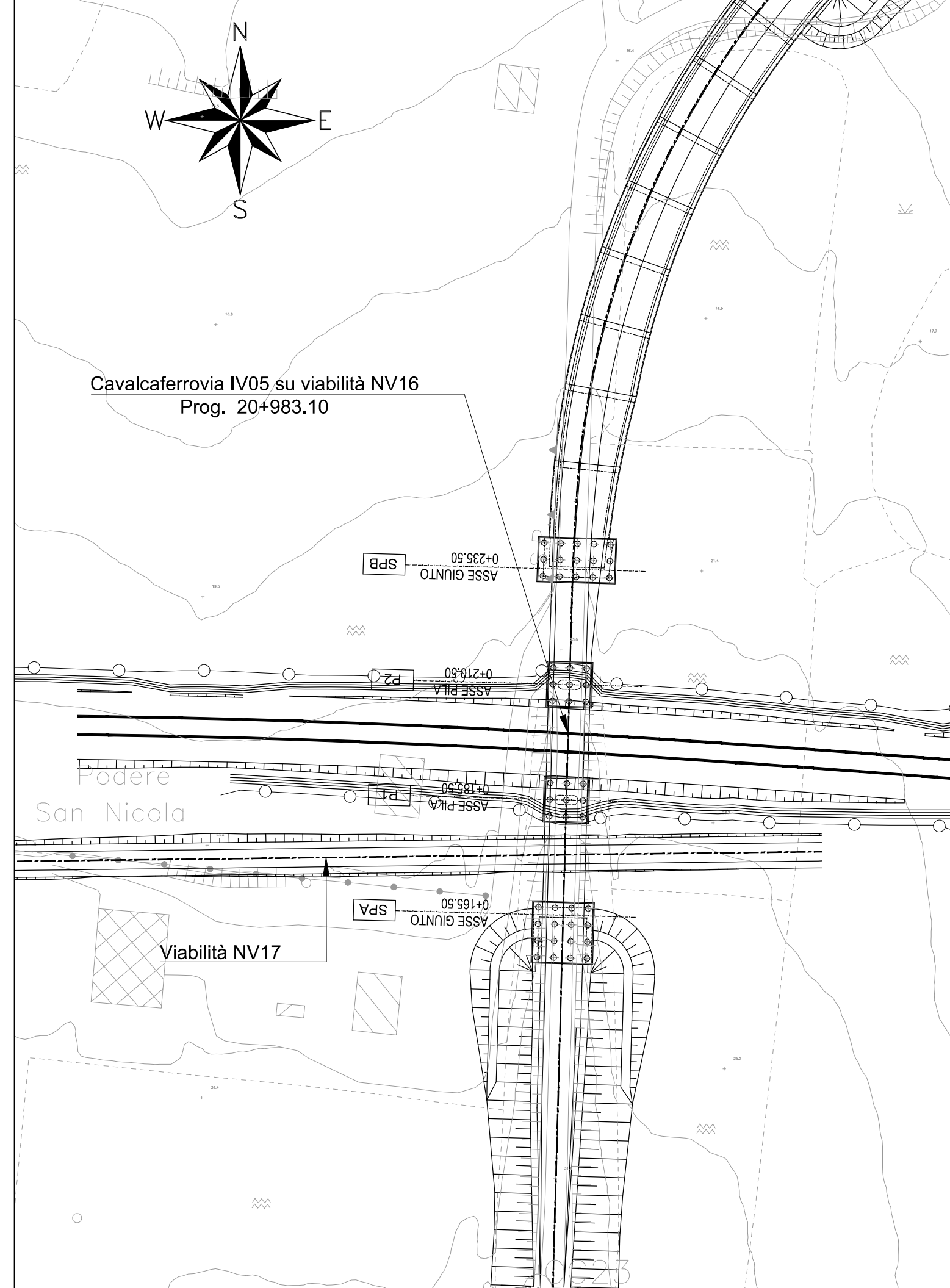
PIANTA CHIAVE SC.1:1000
