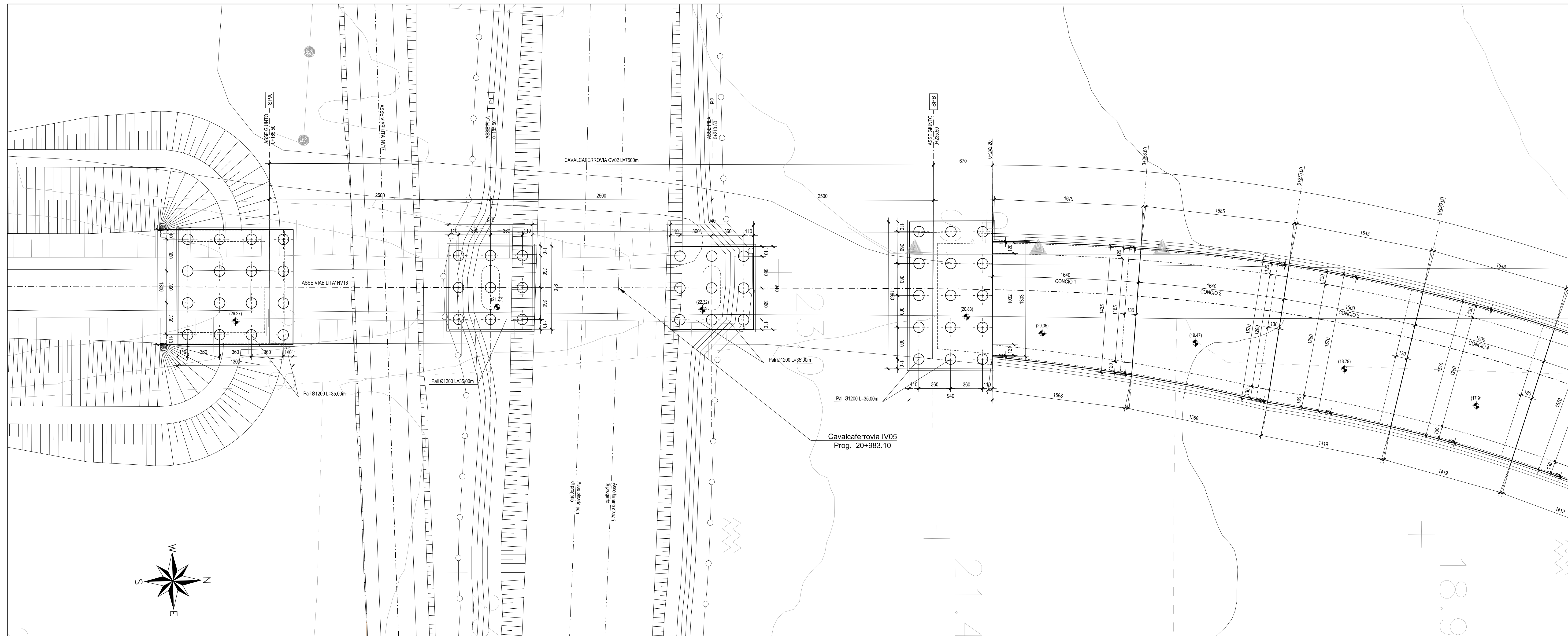
PIANTA FONDAZIONI - Scala 1:200
