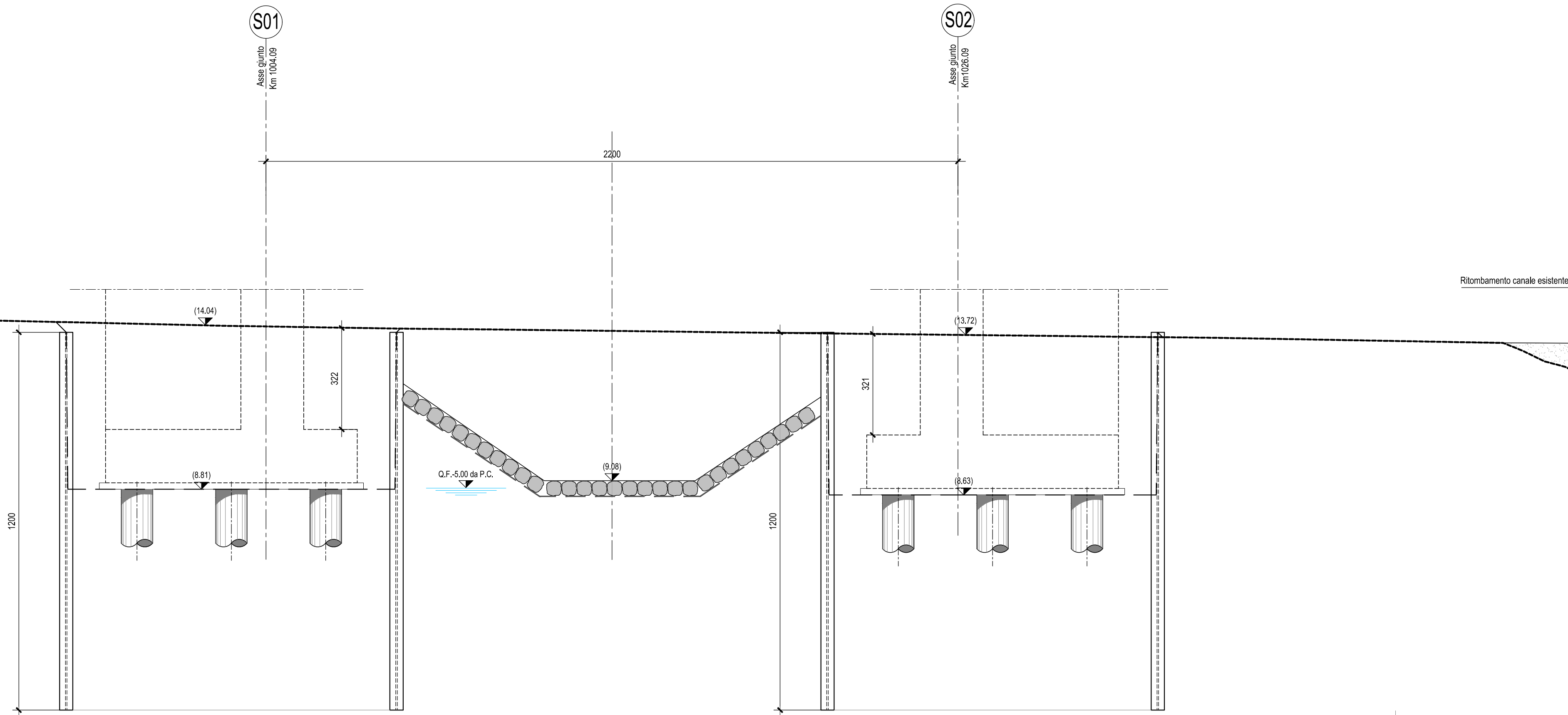
SEZIONE LONITUDINALE-Scala 1:100
