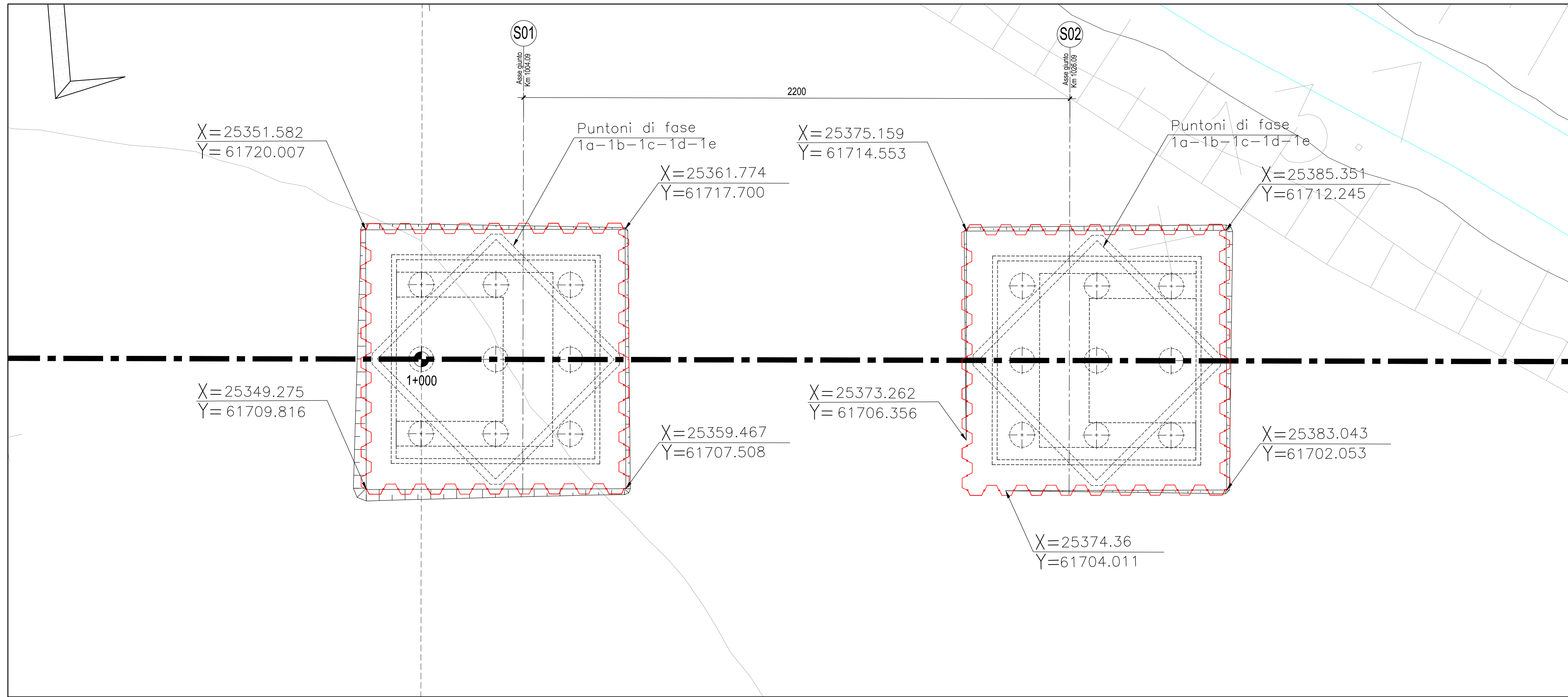
PIANTA FONDAZIONI-Scala 1:100
