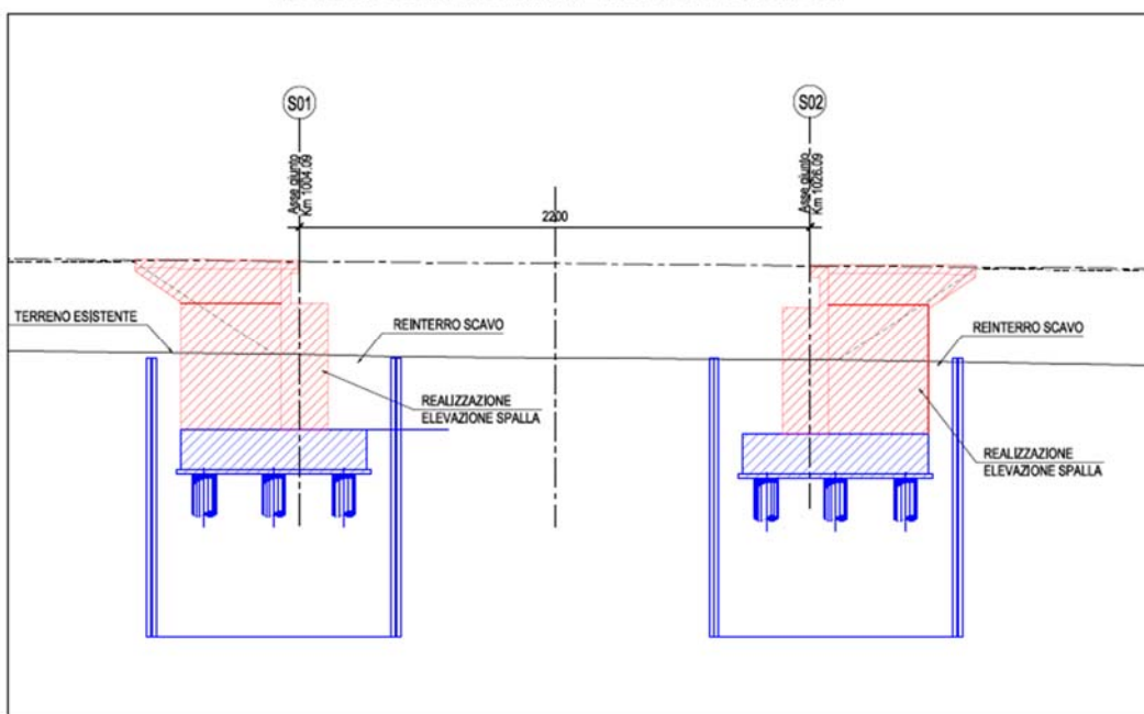
SEZIONE LONGITUDINALE FASE 2-Scala 1:200
