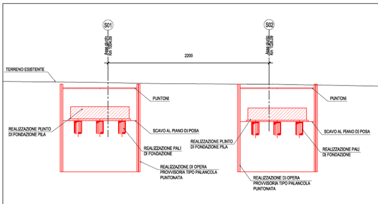
SEZIONE LONGITUDINALE FASE 1 - SOTTOFASI 1a, b, c, d, e - Scala 1:200
