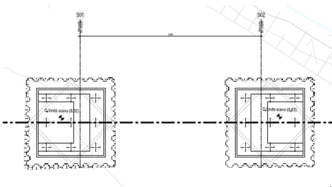
Figura 1.1 : Planimetria a livello fondazioni - IV06
