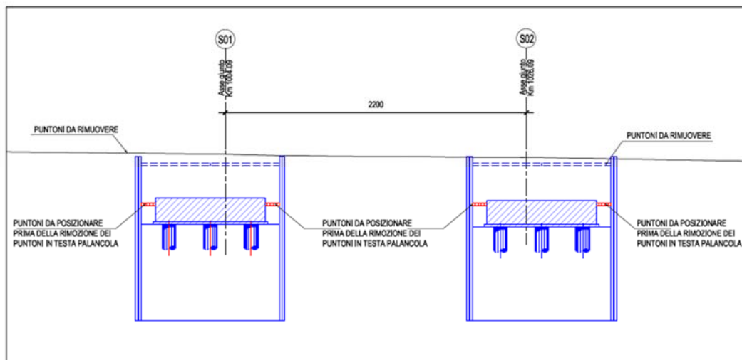
SEZIONE LONGITUDINALE FASE 1 - SOTTOFASI 1f, 1g - Scala 1:200
