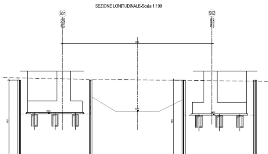
Figura 1.2: Sezione longitudinale – IV06
