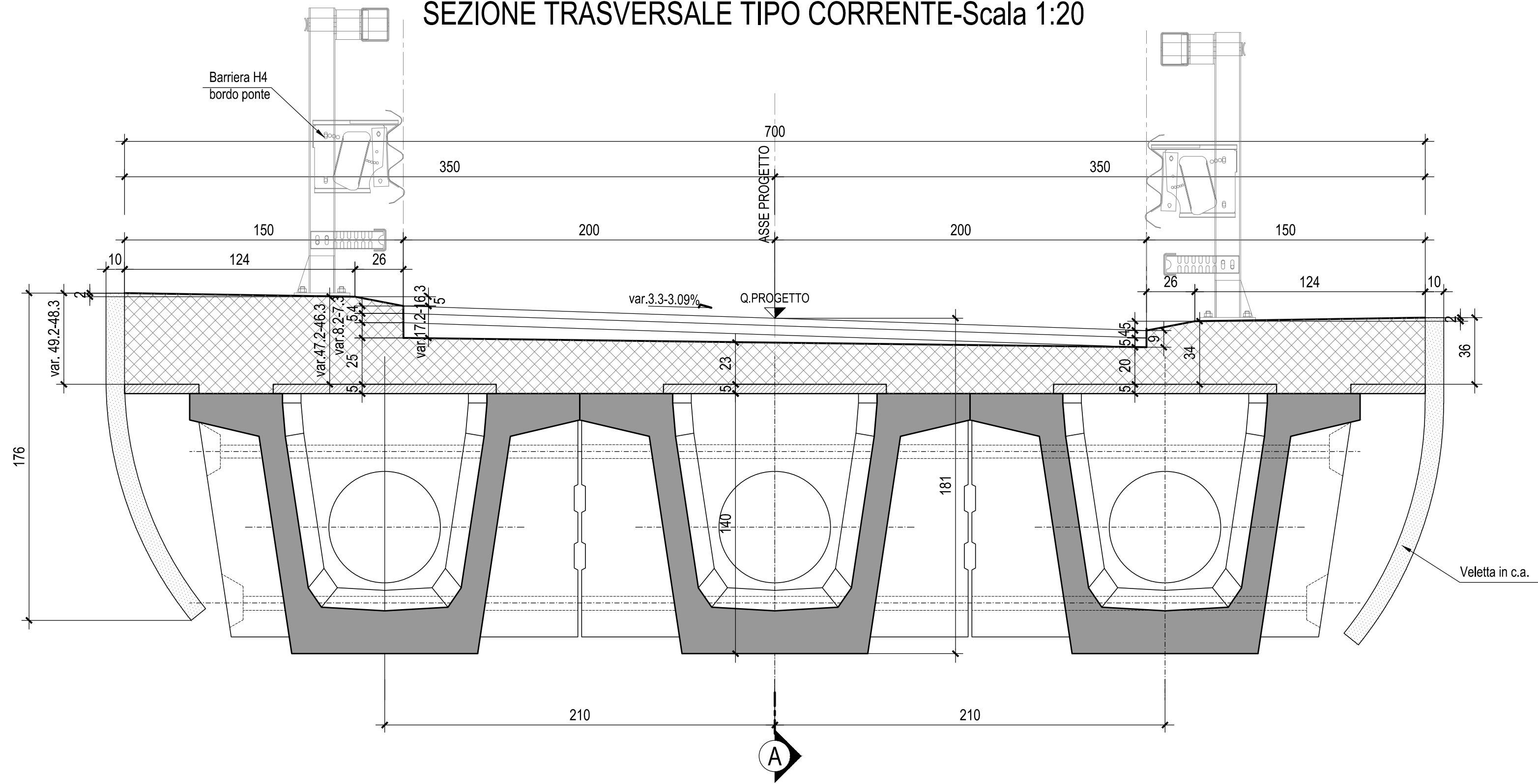
SEZIONE TRASVERSALE TIPO CORRENTE-Scala 1:20
