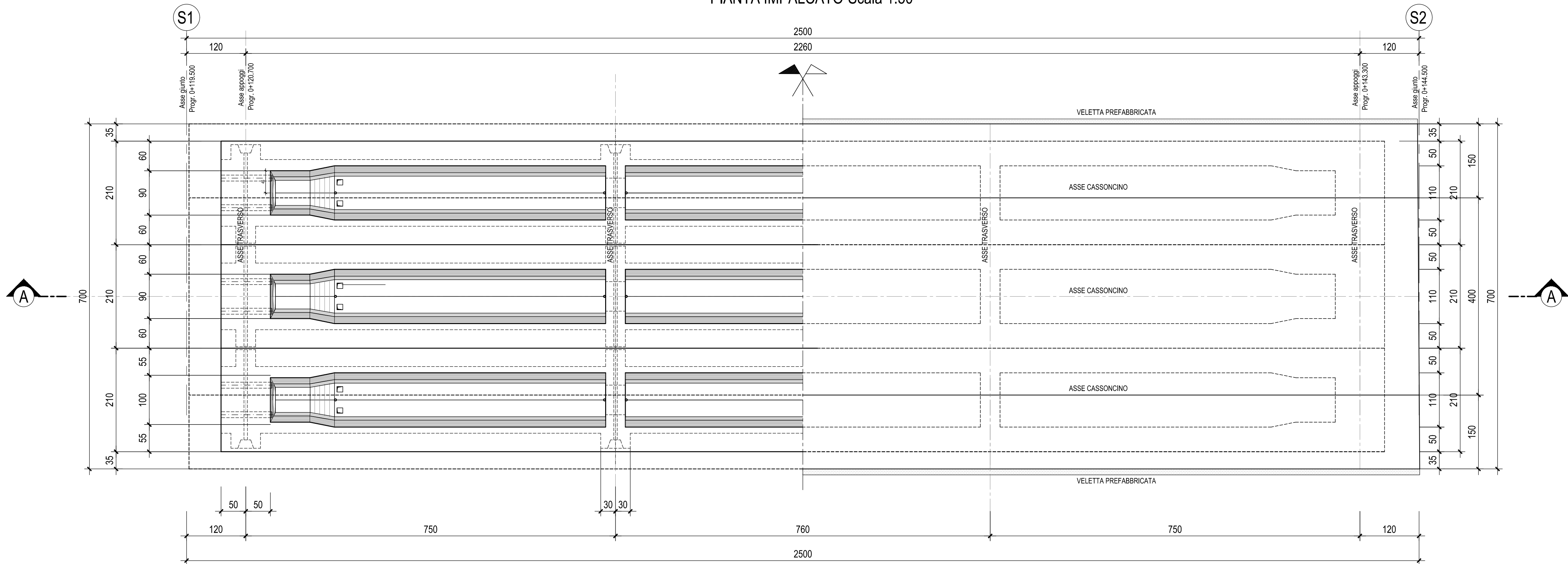
PIANTA IMPALCATO-Scala 1:50
