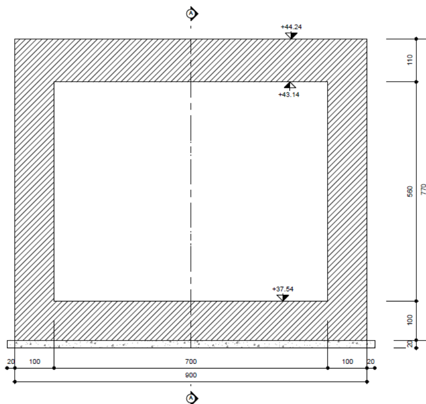
Fig. 5 – Geometria dell'opera
