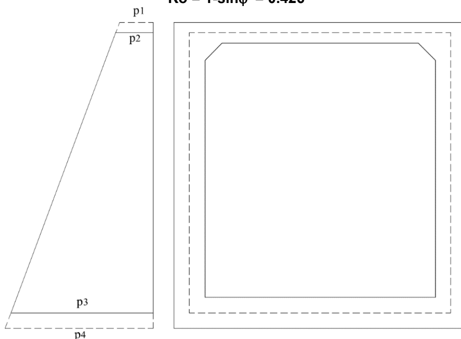
Fig. 11 – Spinta del terreno
