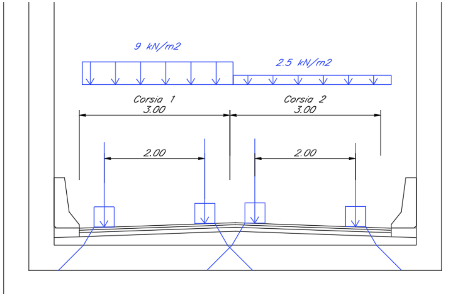
Fig. 19 – Schema di distribuzione del carico mobile considerate sulla soletta inferiore ACC1-VH
