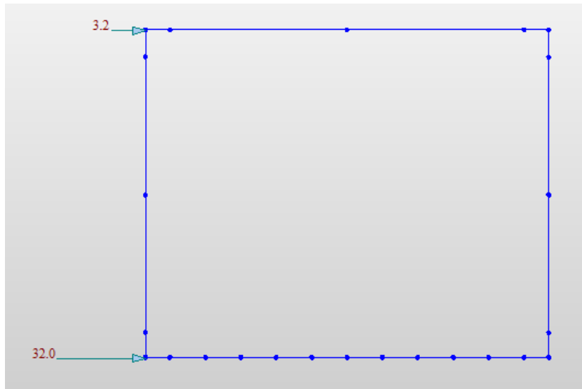
Fig. 13 – Applicazione carico concentrato sul piedritto sinistro (simile per piedritto destro) (STS, STD)
