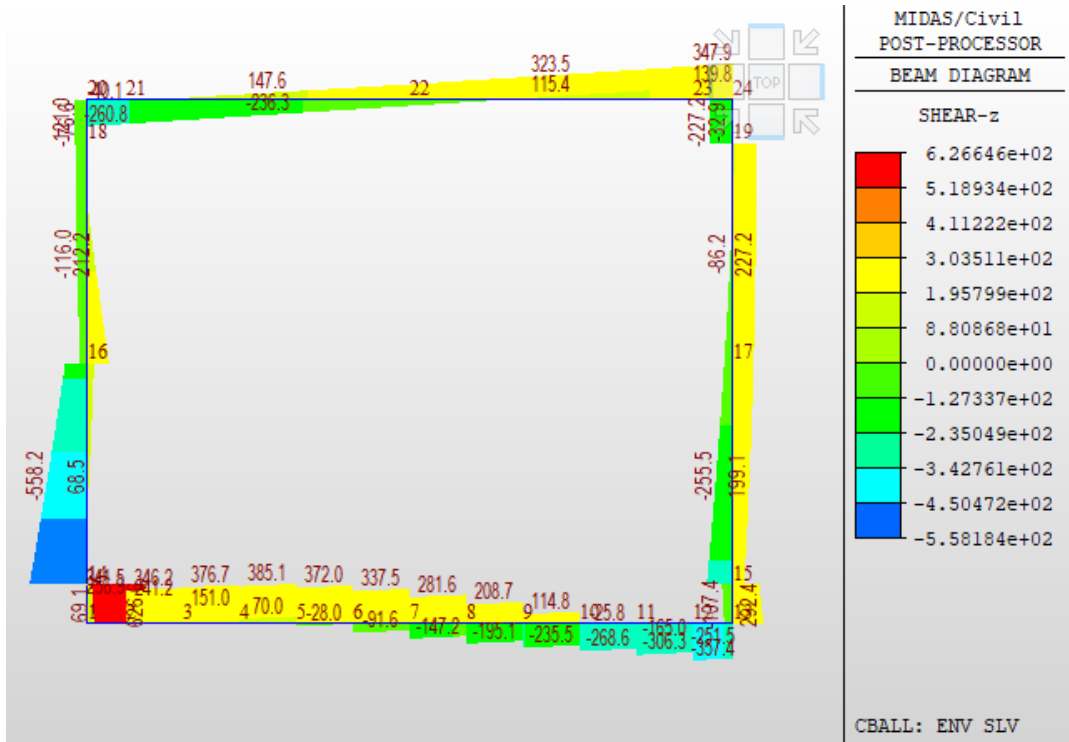
Fig. 34 – Involuppo sforzi taglianti SLV
