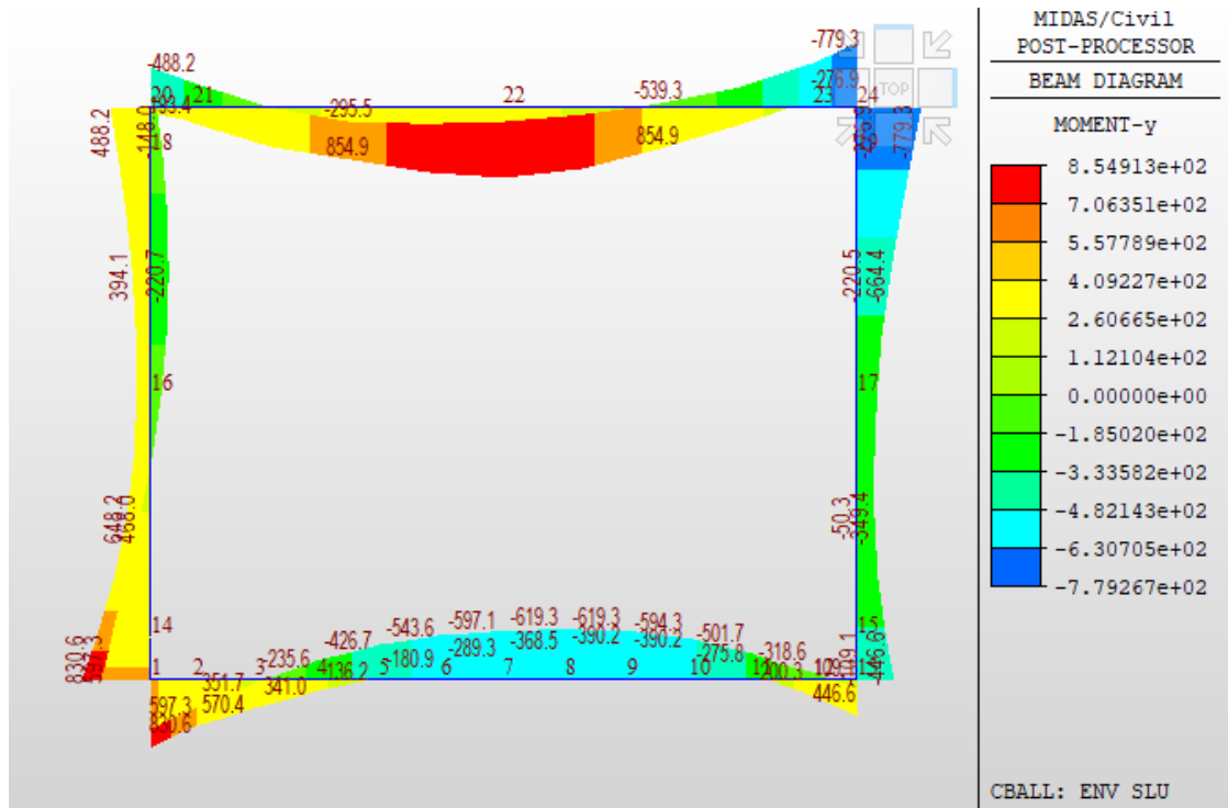
Fig. 30 – Involuppo momenti flettenti SLU
