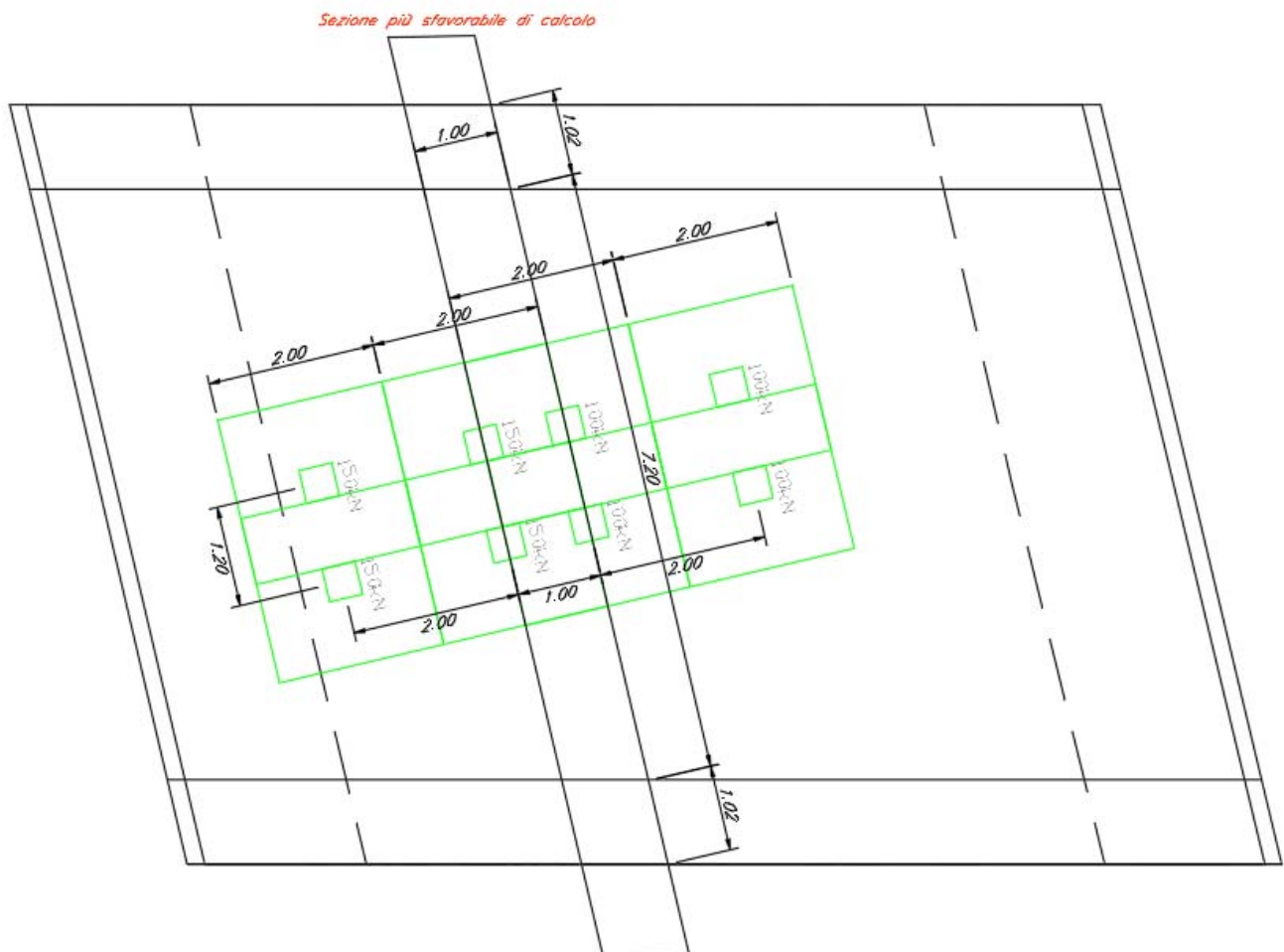
Fig. 6 – Sezione più sfavorevole di calcolo
