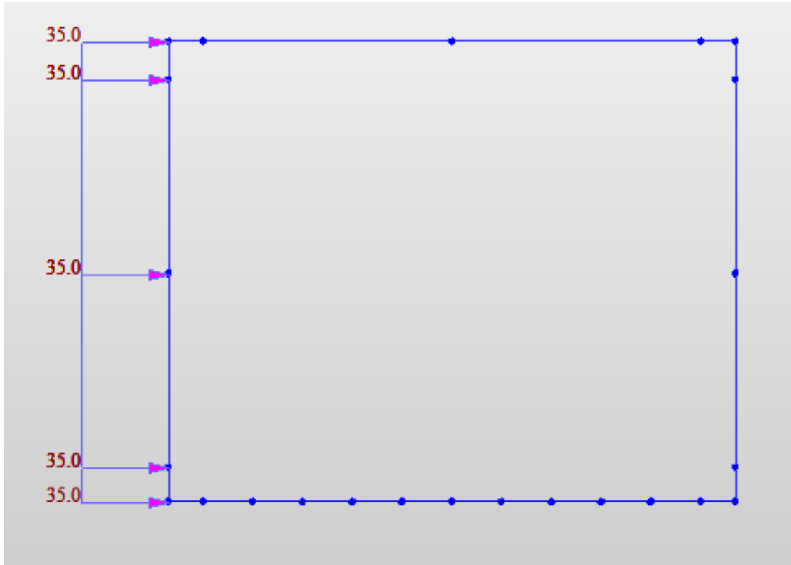
Fig. 26 – Sovraspinta sismica distribuite
