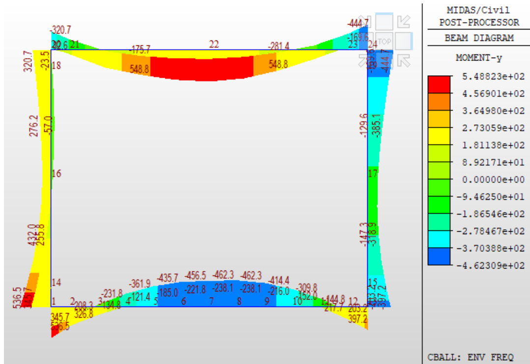
Fig. 37 – Involuppo momenti flettenti FREQ
