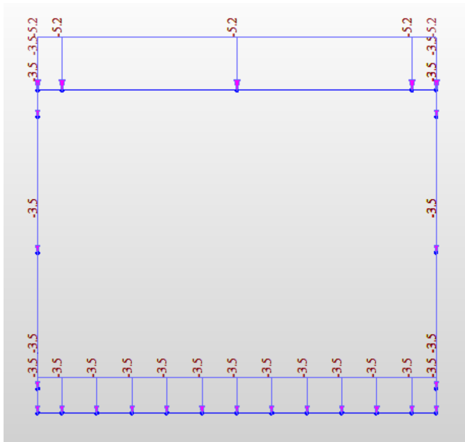
Fig. 29 – SISVER
