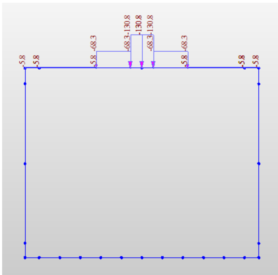
Fig. 16 – Carico mobile considerate ACC1, sul MIDAS
