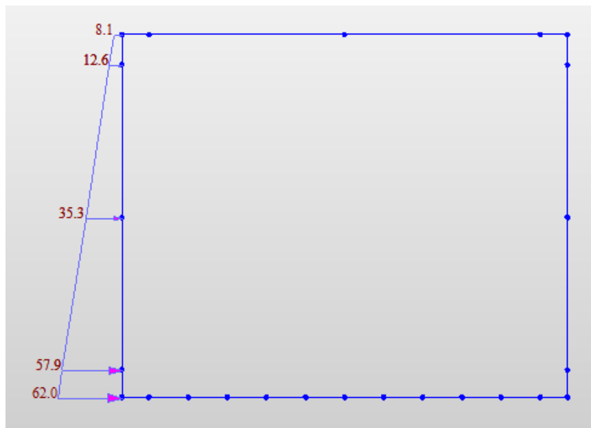
Fig. 12 – Applicazione Spinta terreno (simile per piedritto destro) (STS, STD)
