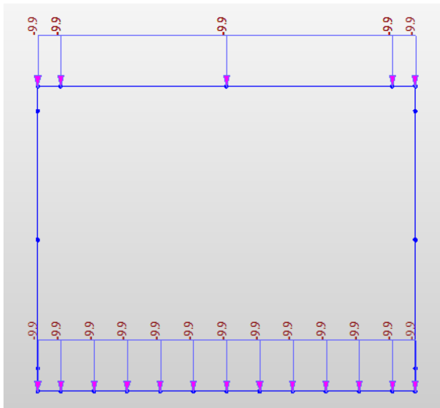
Fig. 9 – Carichi distribuiti verticali permanenti (PERM)
