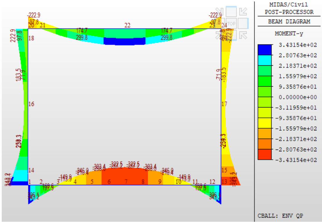
Fig. 38 – Involuppo momenti flettenti QP
