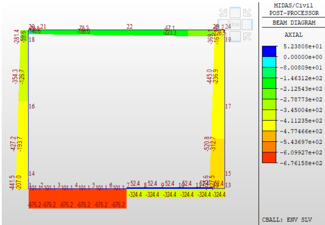
Fig. 35 – Involuppo azioni assiali SLV
