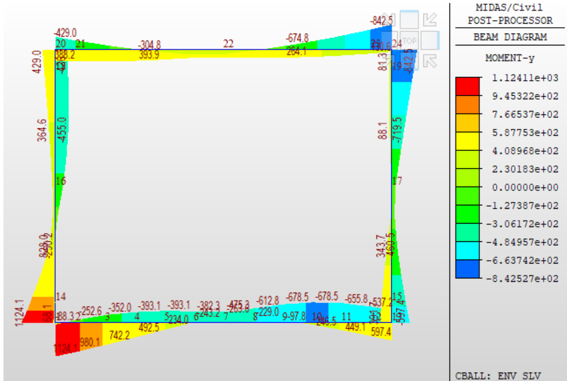
Fig. 33 – Involuppo momenti flettenti SLV
