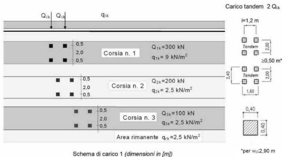
Fig. 14 – NTC08-schema di carico 1
