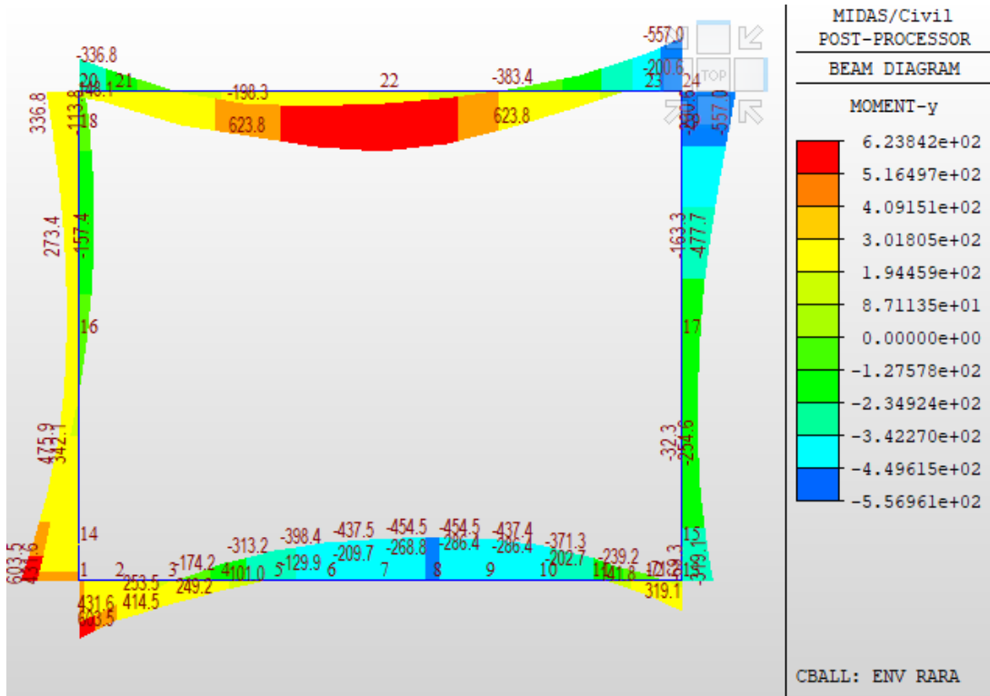
Fig. 36 – Involuppo momenti flettenti RARA
