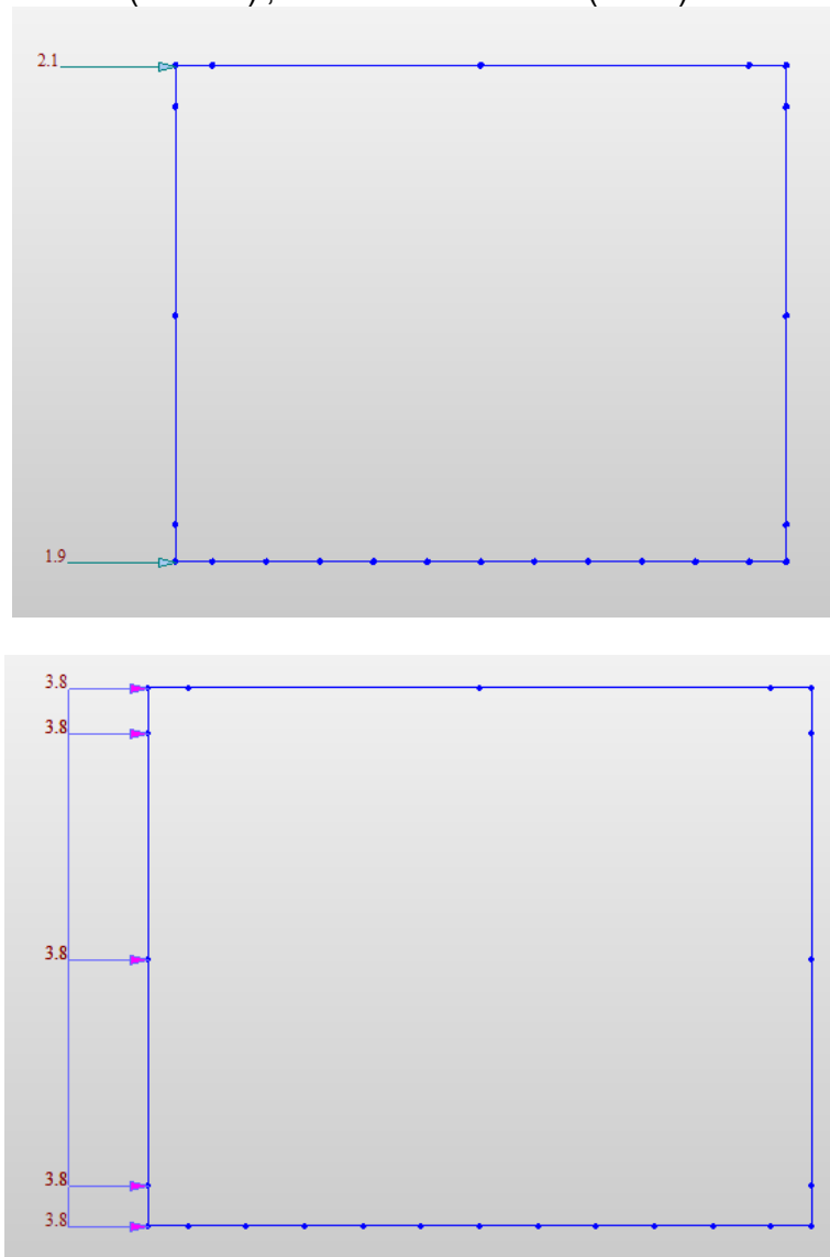
Fig. 21 – Spinta dei carichi ripartiti SAS
