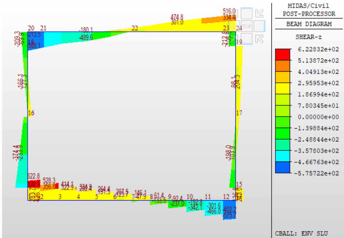
Fig. 31 – Involuppo sforzi taglienti SLU
