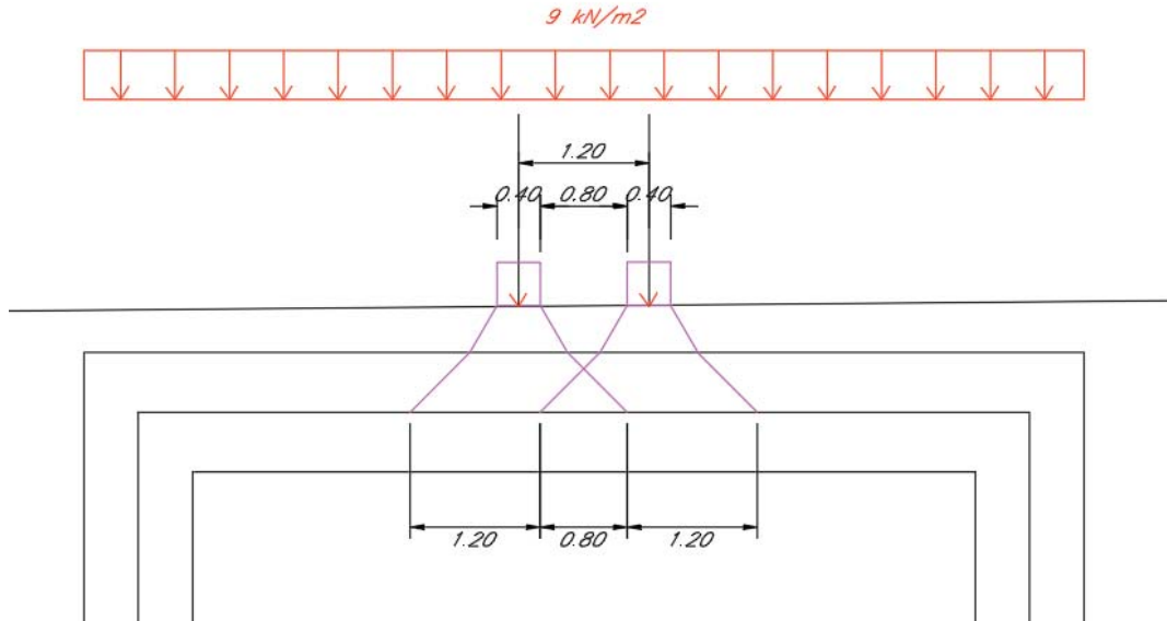
Fig. 15 – Schema di distribuzione del carico mobile considerate ACC1
