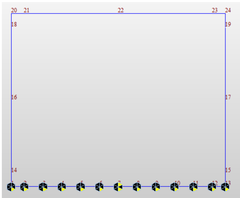
Fig. 4 – Modellazione molle elastiche in MIDAS
