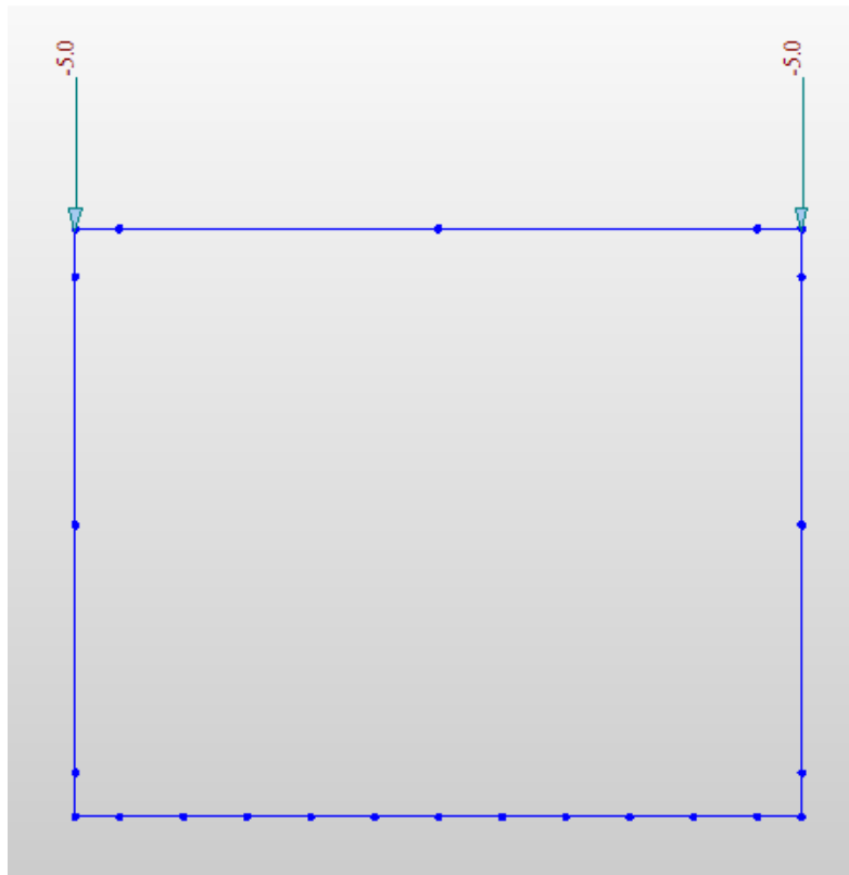
Fig. 10 – Carichi puntuali verticali permanenti (PERM)
