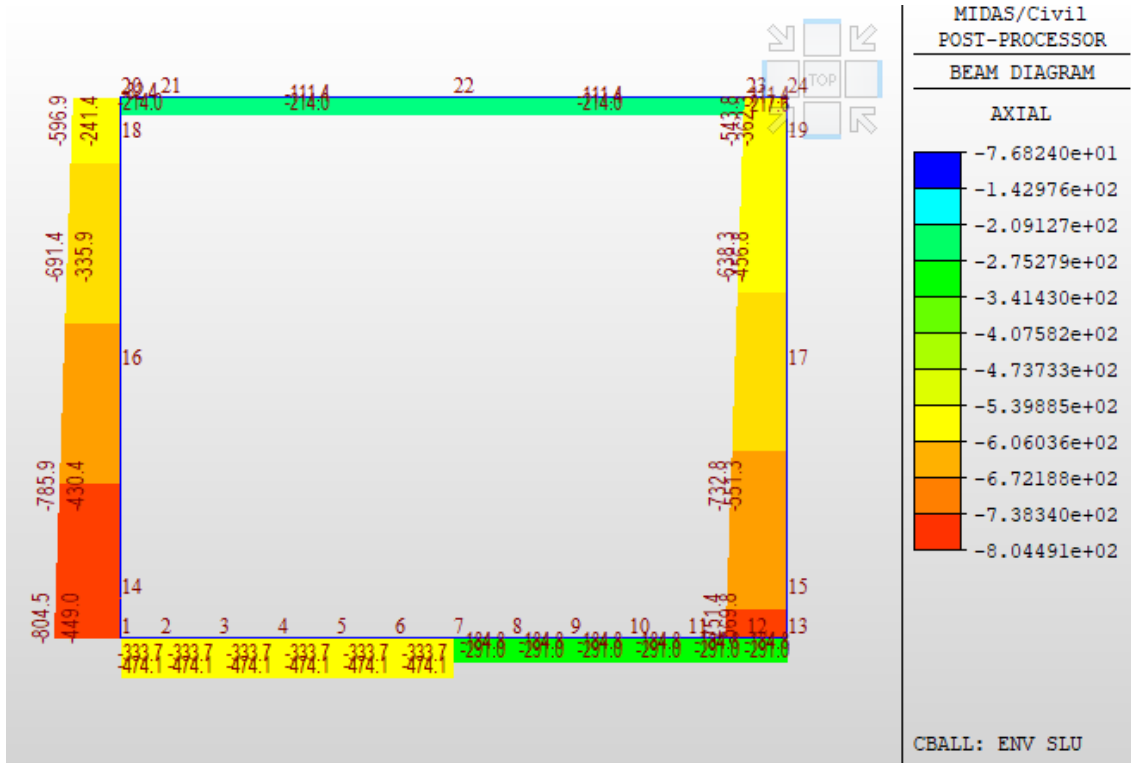
Fig. 32 – Involuppo azioni assiali SLU
