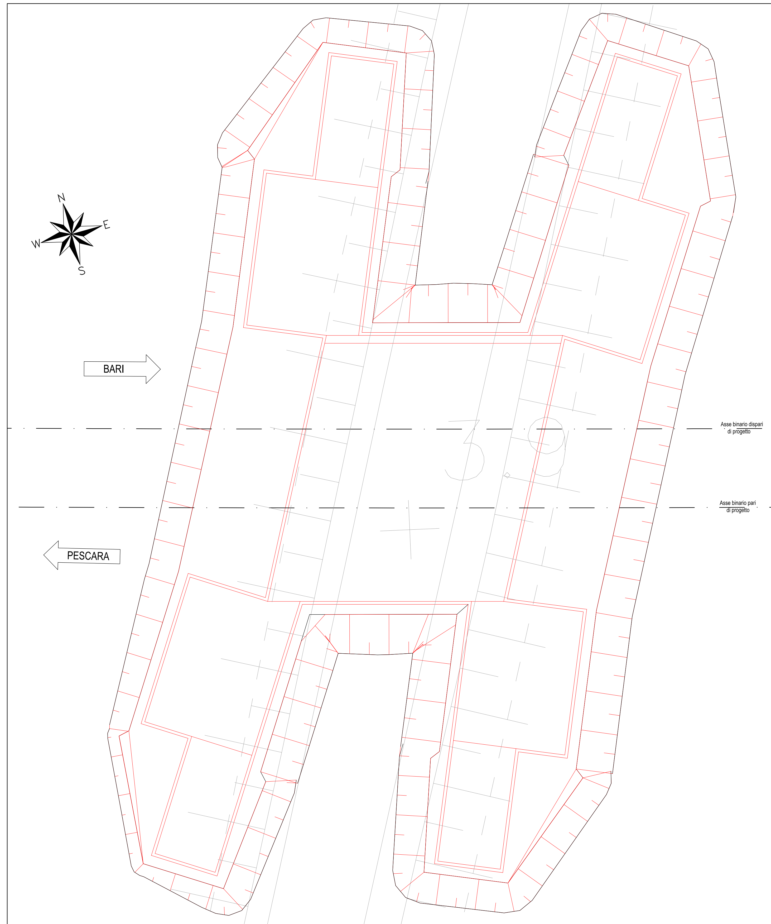
PLANIMETRIA FASE 1-Scala 1:100
