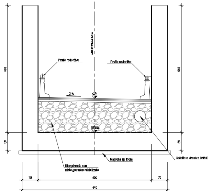
Figura 1 - Sezione trasversale dell'opera
