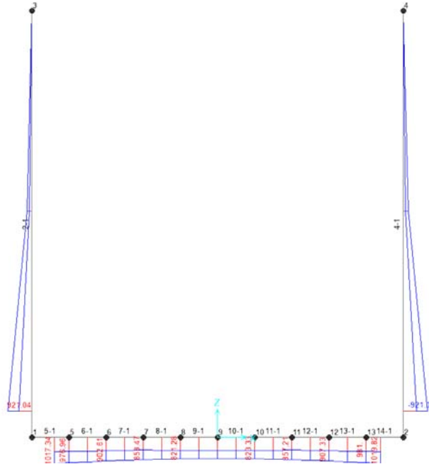
Figura 4 -Involuppo momenti flettenti SLU
