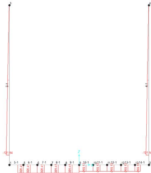
Figura 11– Involuppo azioni assiali SLE rara
