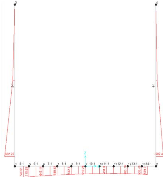
Figura 10– Involuppo momenti flettenti SLE rara
