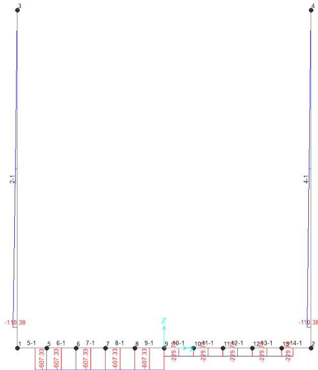
Figura 9– Involuppo azioni assiali SLV
