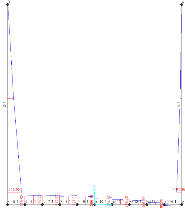
Figura 8– Involuppo sforzi taglianti SLV
