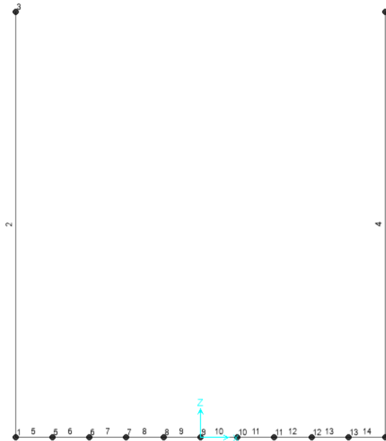
Figura 3 – Numerazione aste e nodi
