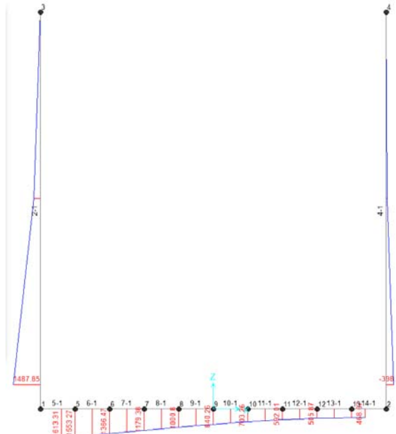
Figura 7–Inviluppo momenti flettenti SLV
