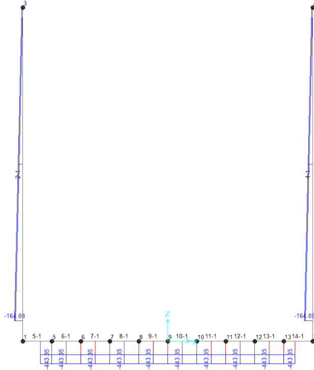
Figura 6– Inviluppo azioni assiali SLU
