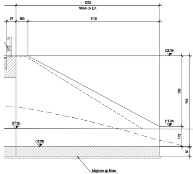
Figura 2 - Sezione longitudinale
