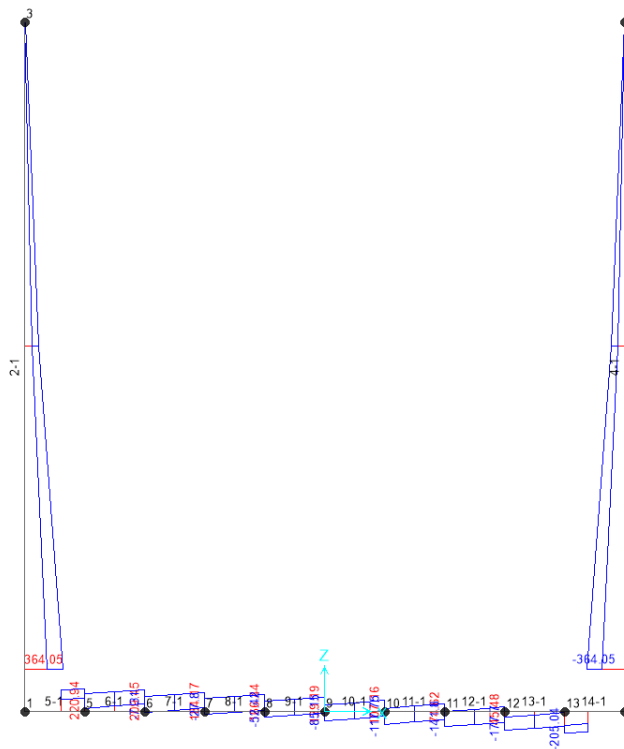
Figura 5 -Involuppo sforzi taglienti SLU
