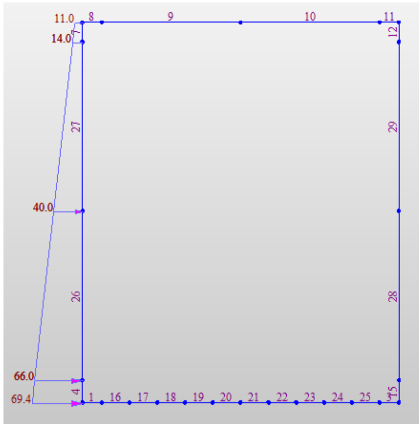
Fig. 10 –Applicazione Spinta terreno (simile per piedritto destro) (STS, STD)
