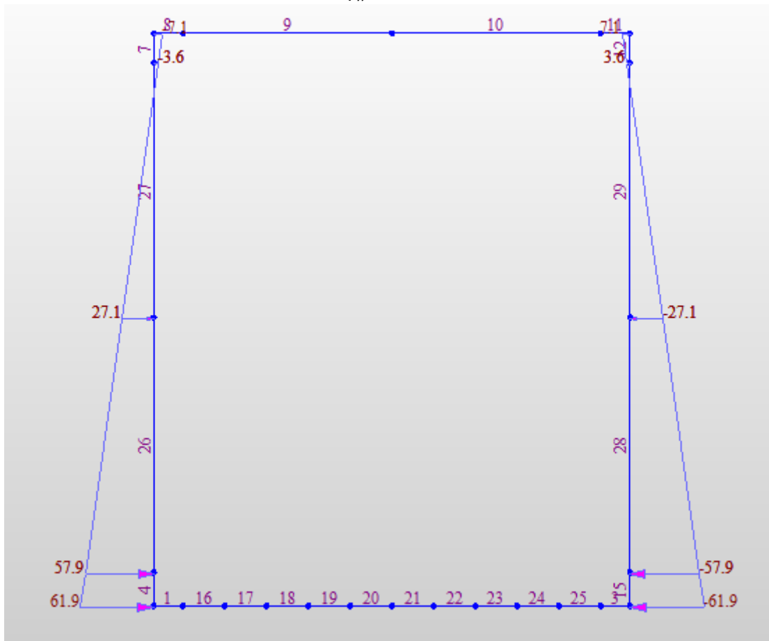
Fig. 12 –Diagramma delle pressioni di falda.
