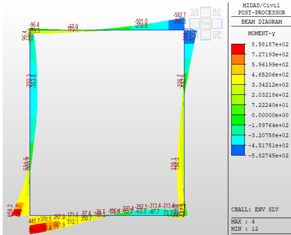
Fig. 34 – Involuppo momenti flettenti SLV
