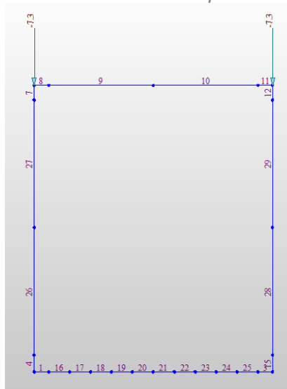
Fig. 8 – Carichi puntuali verticali permanenti (PERM)
