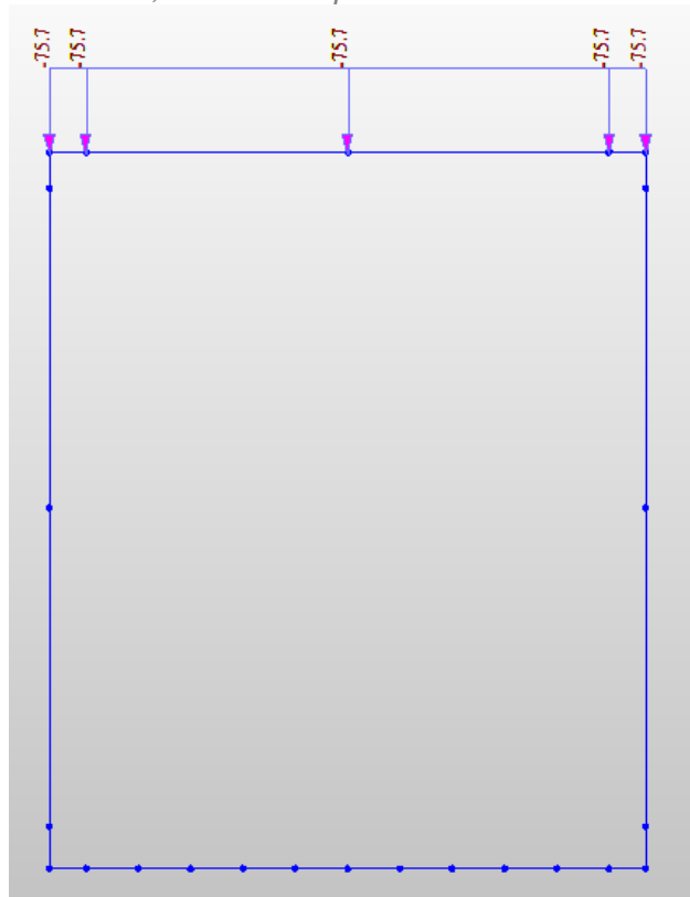
Fig. 16 – Carico LM71; condizione per massimizzare il taglio
