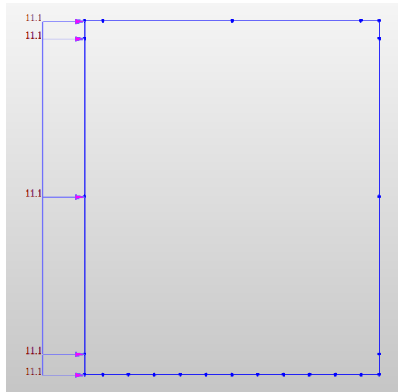
Fig. 17 – Spinta carico accidentale distribuito nel piedritto sinistro (simile per il piedritto destro) (SAS, SAD)
