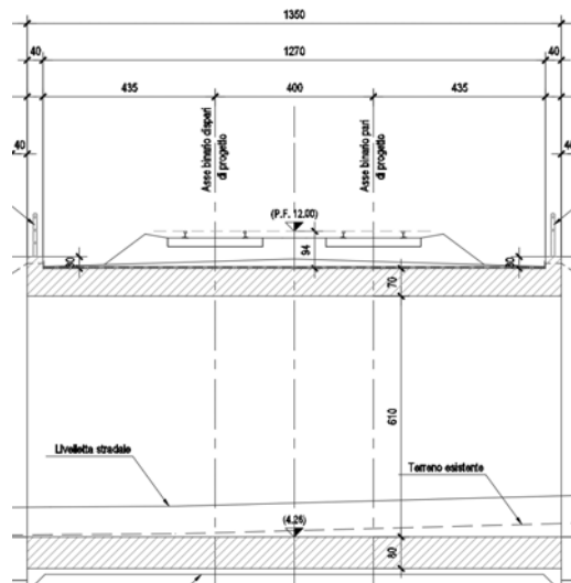
Fig. 2 – Sezione longitudinale
