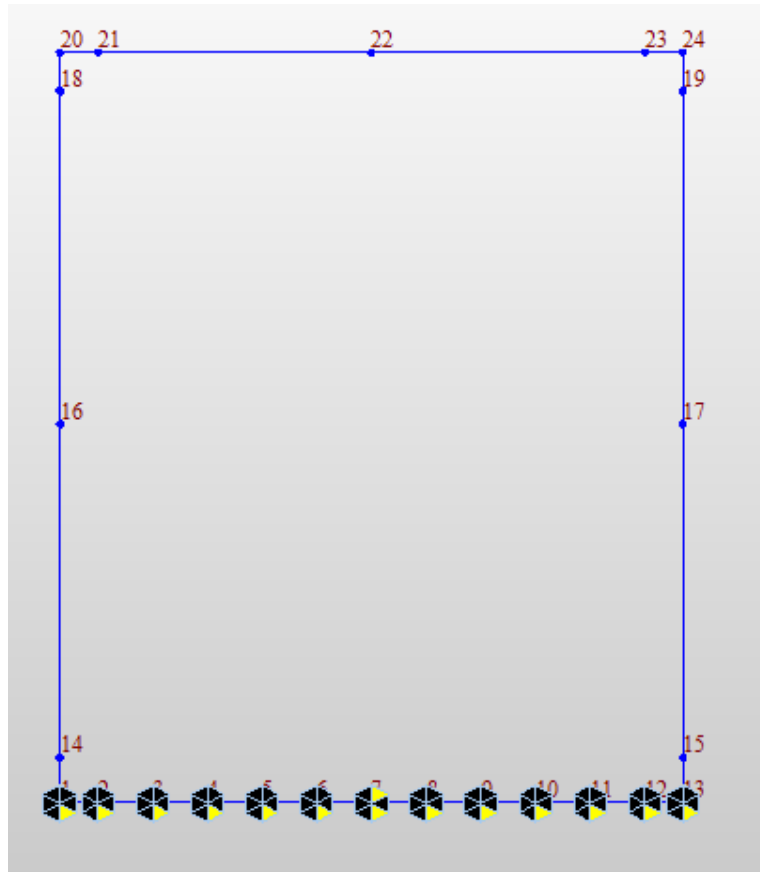
Fig. 3 – Modellazione molle elastiche in MIDAS
