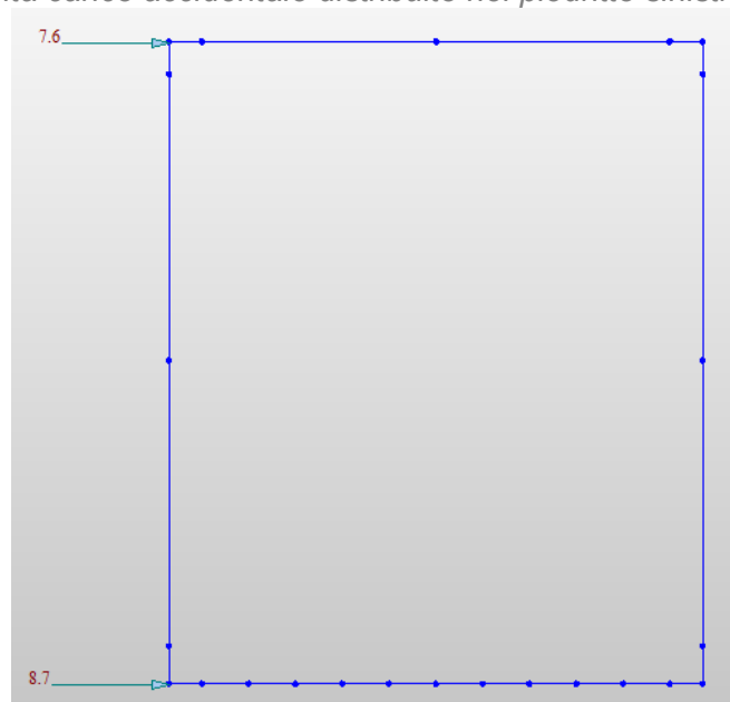
Fig. 20 – Spinta carico accidentale puntuale nel piedritto sinistro (SASXLM71)
