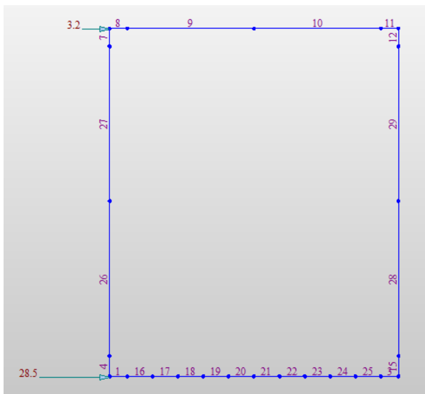
Fig. 11 –Applicazione carico concentrato sul piedritto sinistro (simile per piedritto destro) (STS, STD)
