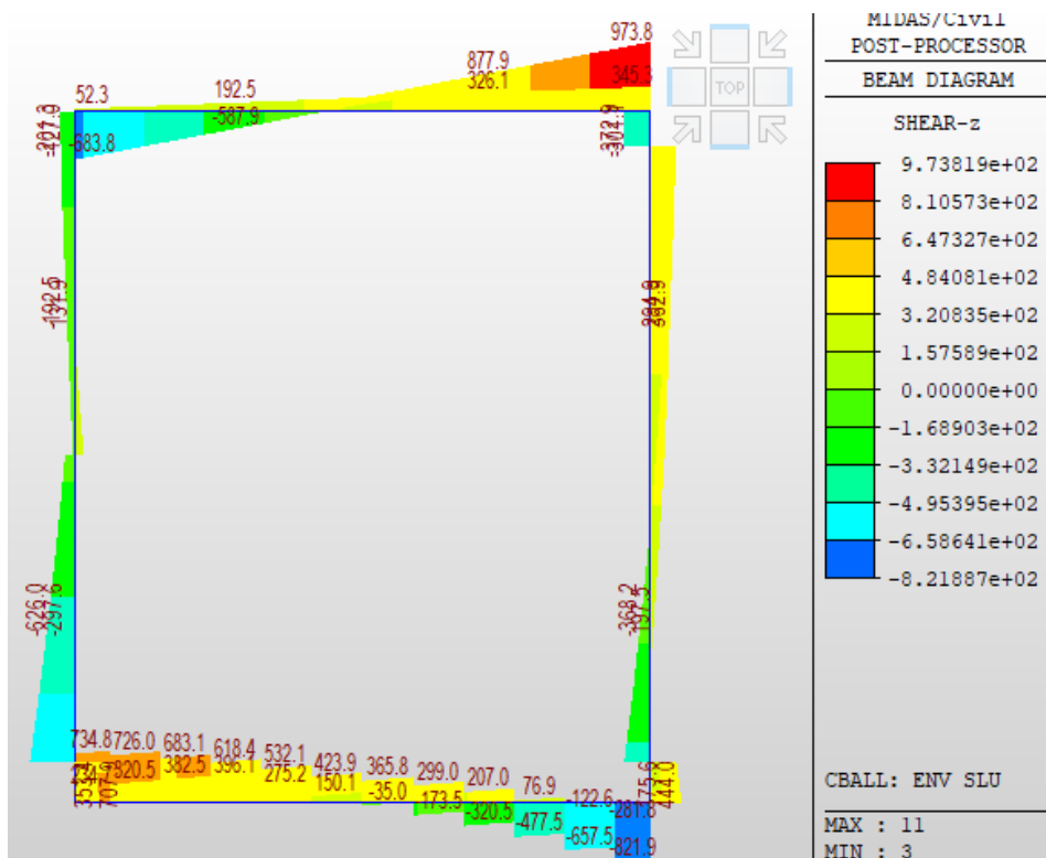
Fig. 32 – Involuppo sforzi taglienti SLU
