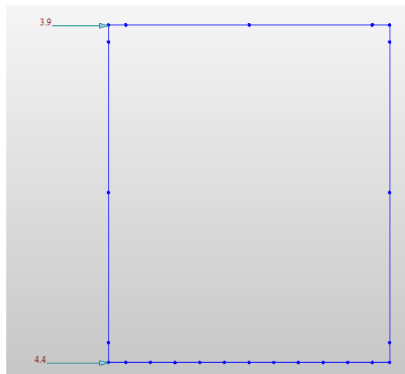
Fig. 18 – Spinta carico accidentale puntuale nel piedritto sinistro (simile per piedritto destro) (SAS, SAD)
