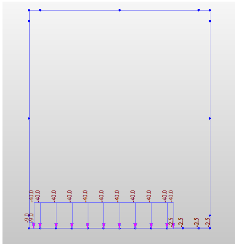
Fig. 24 – Carichi variabili sulla soletta di fondazione in MIDAS (TRAF)
