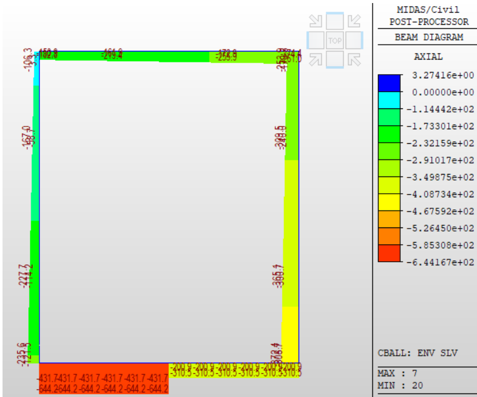
Fig. 36 – Involuppo azioni assiali SLV
