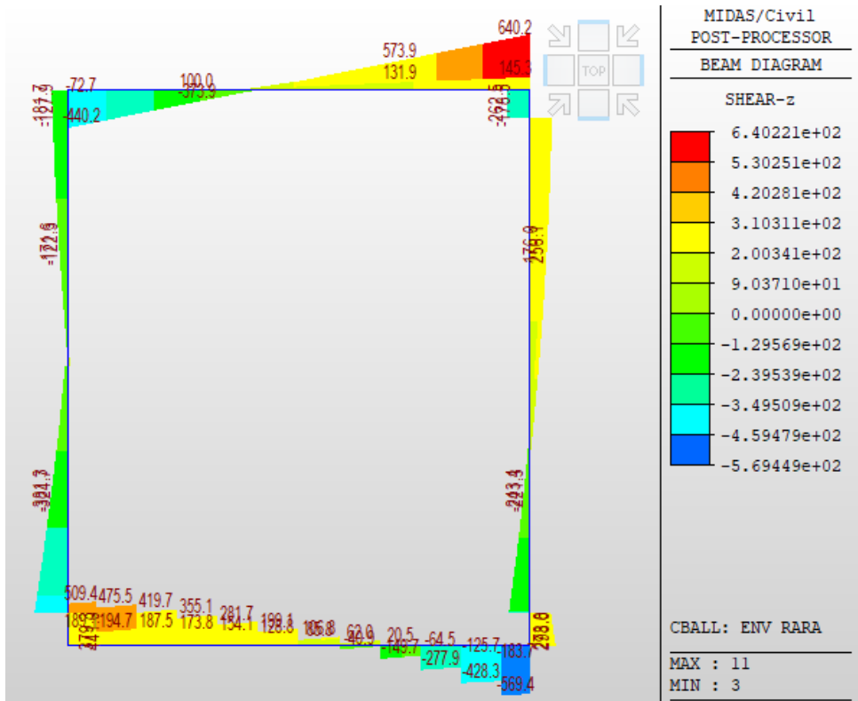
Fig. 38 – Involuppo sforzi taglianti RARA
