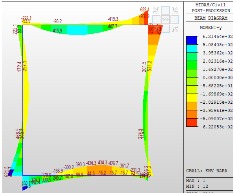
Fig. 37 – Involuppo momenti flettenti RARA
