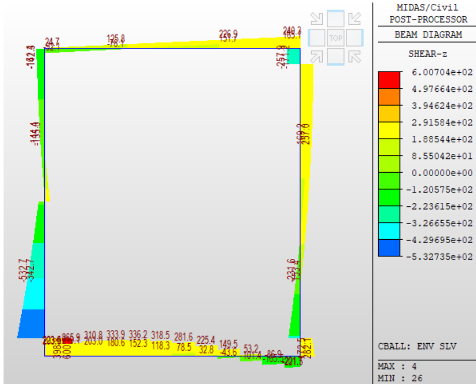
Fig. 35 – Involuppo sforzi taglianti SLV
