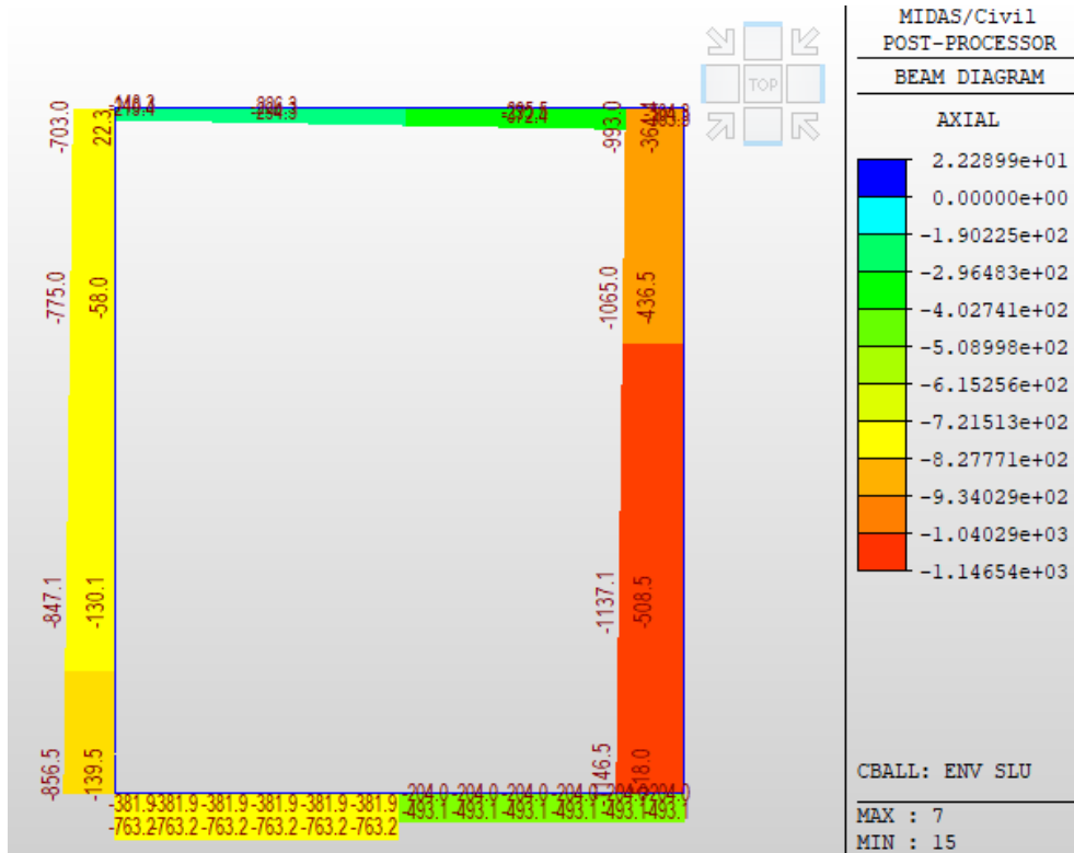
Fig. 33 – Involuppo azioni assiali SLU
