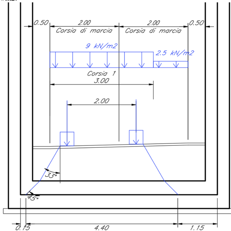
Fig. 23 – Schema di distribuzione del carico mobile considerate
