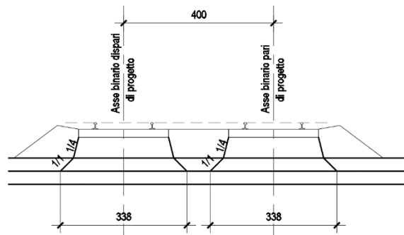
Fig. 14 – Diffusione del carico in senso trasversale
