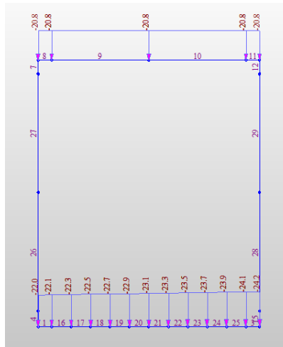
Fig. 7 – Carichi distribuiti verticali permanenti (PERM)
