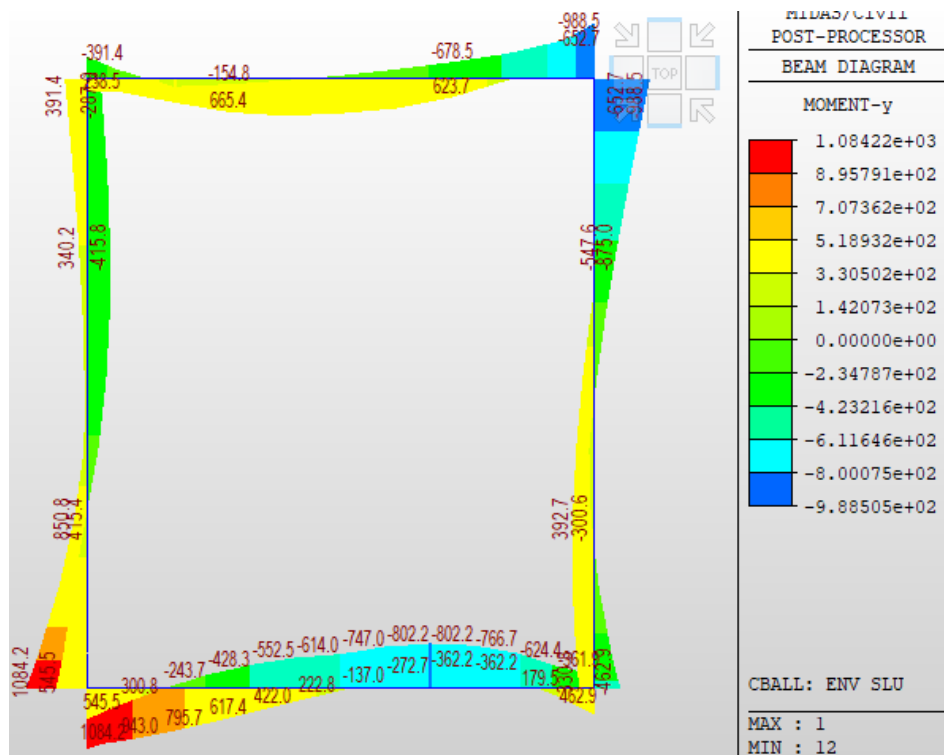
Fig. 31 – Involuppo momenti flettenti SLU
