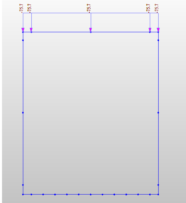
Fig. 15 – Carico LM71; condizione per massimizzare il momento flettente
