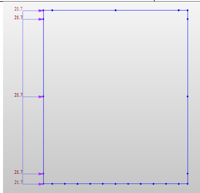
Fig. 19 – Spinta carico accidentale distribuito nel piedritto sinistro (SASXLM71)
