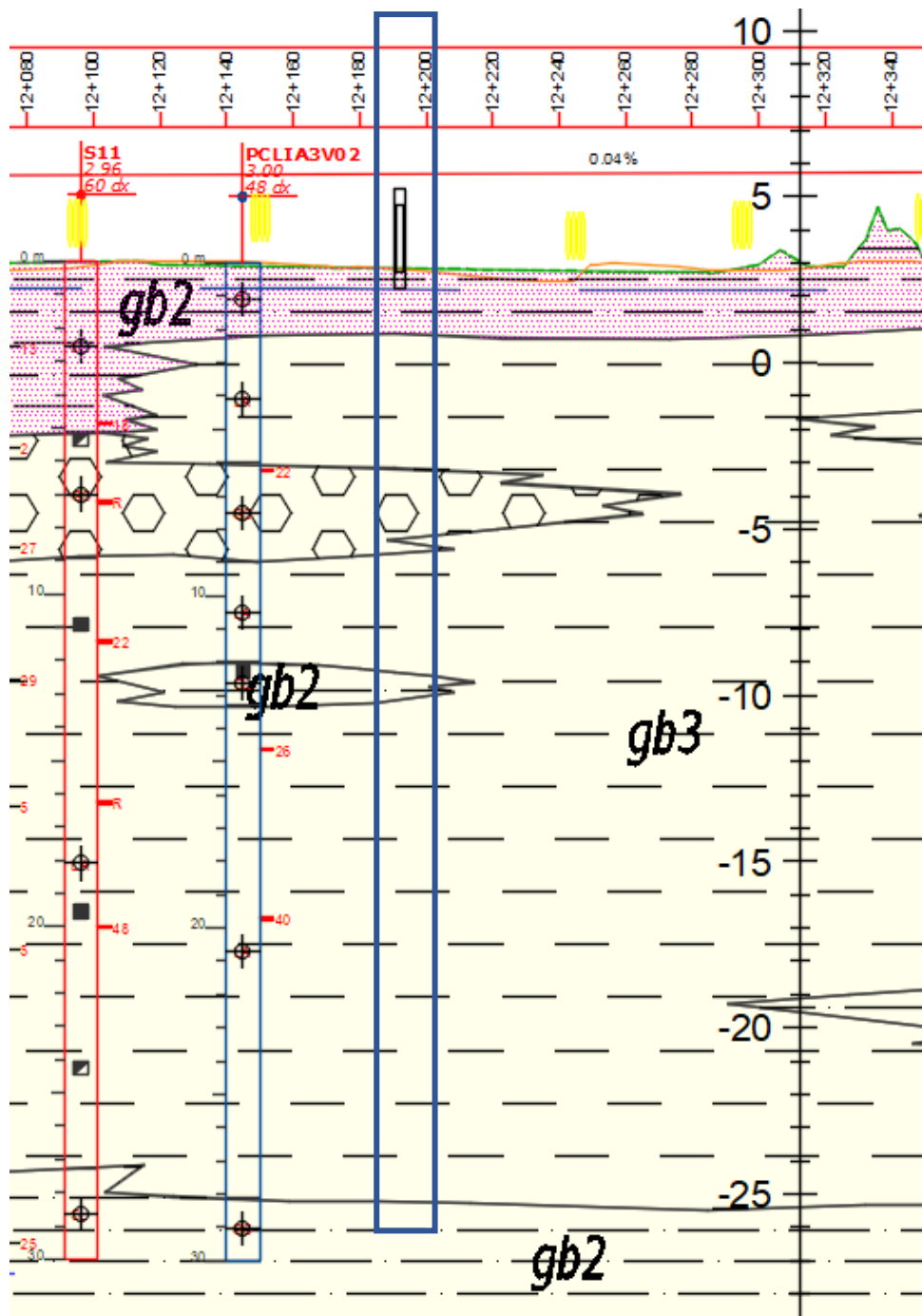
Fig. 4 – Stralcio del profilo geotecnico
