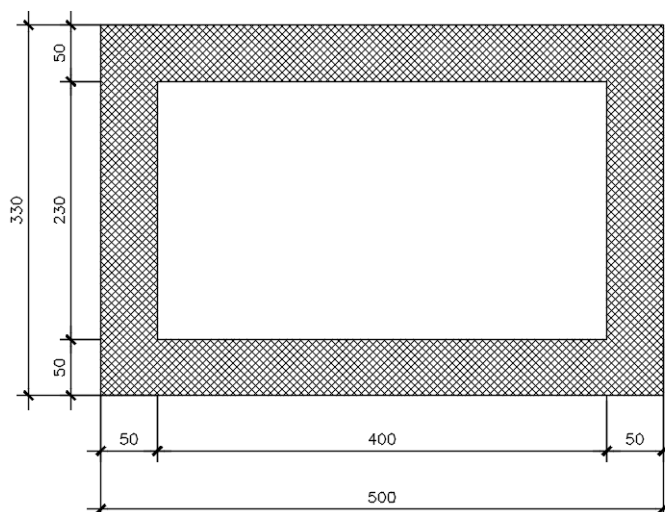
Fig. 6 – Stralcio Modello geometrico
