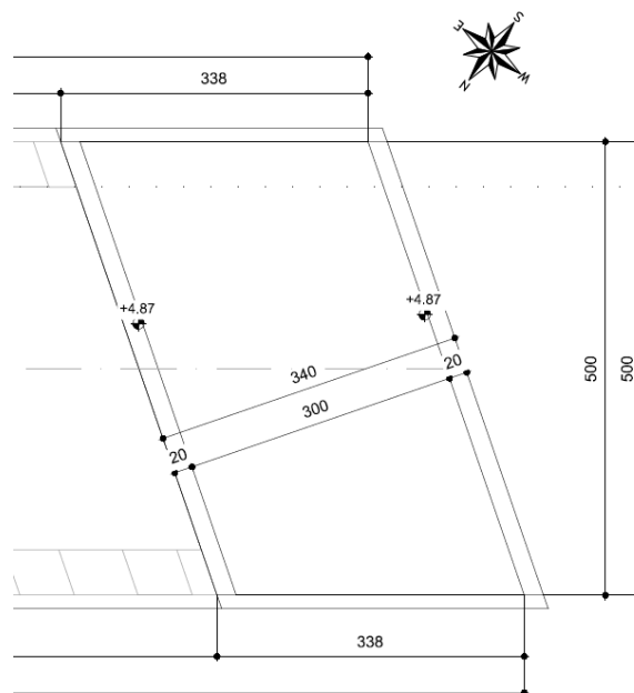
Fig. 2 – Sezione trasversale dell'opera
