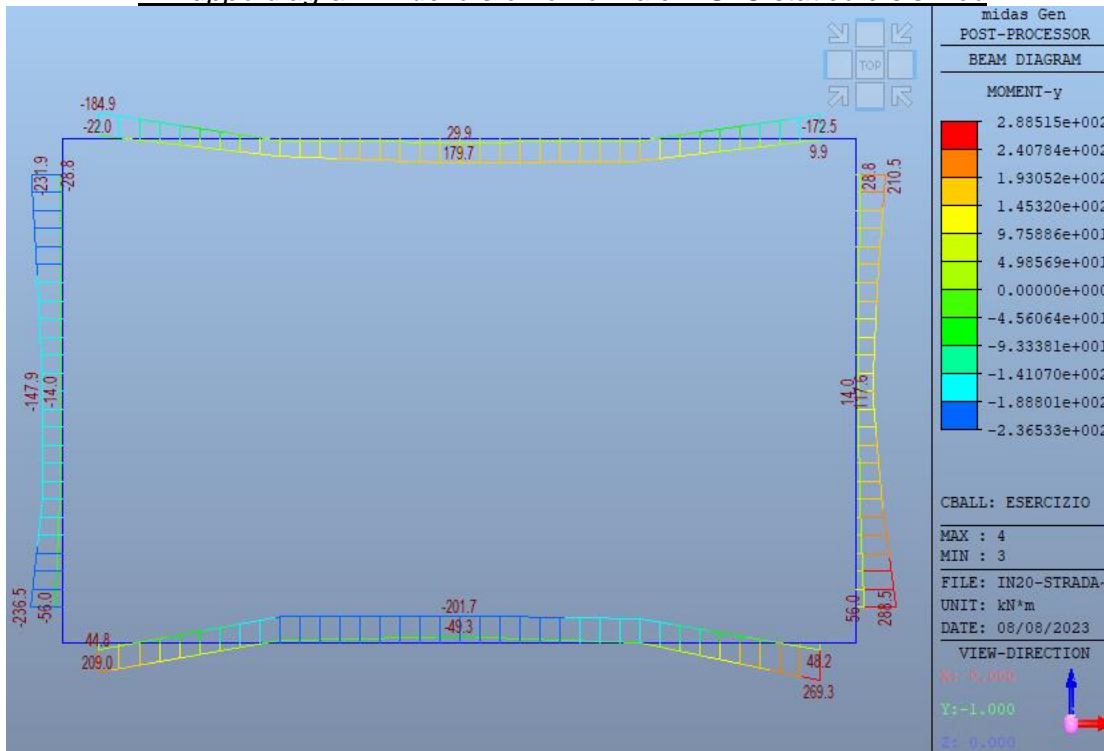
Inviluppo diagrammi del momento flettente – SLE
