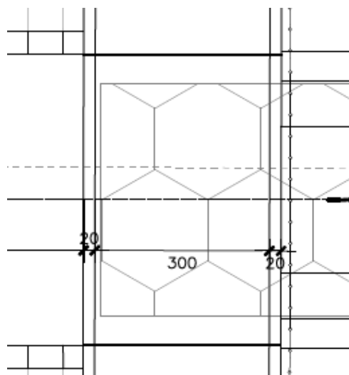
Fig. 2 – Pianta scatolare stradello
