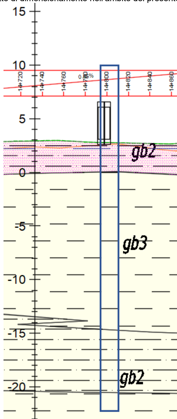
Fig. 4 – Stralcio del profilo geotecnico
