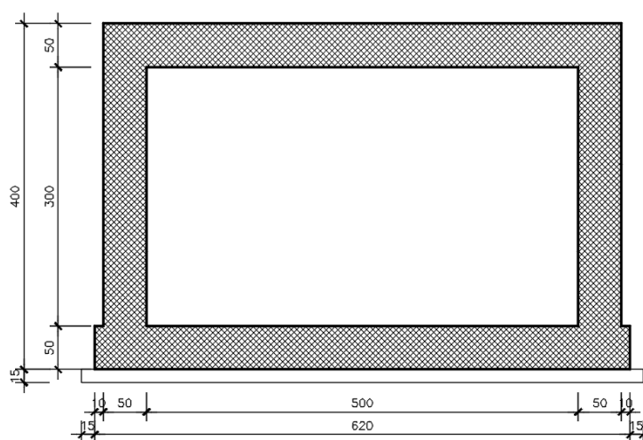
Fig. 6 – Stralcio Modello geometrico
