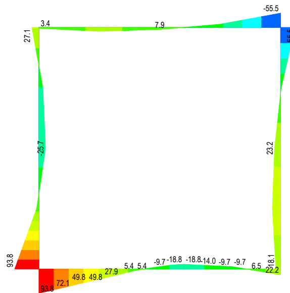
Fig. 10 – Inviluppo momenti flettenti SLV
