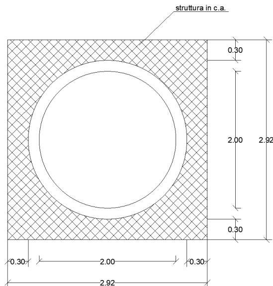
Figura 1: Sezione trasversale dell'opera
