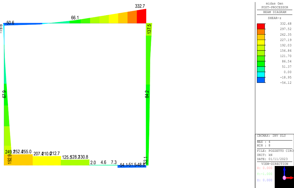
Fig. 8 – Involuppo sforzi taglianti SLU
