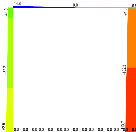
Fig. 11 – Inviluppo sforzi taglianti SLV
