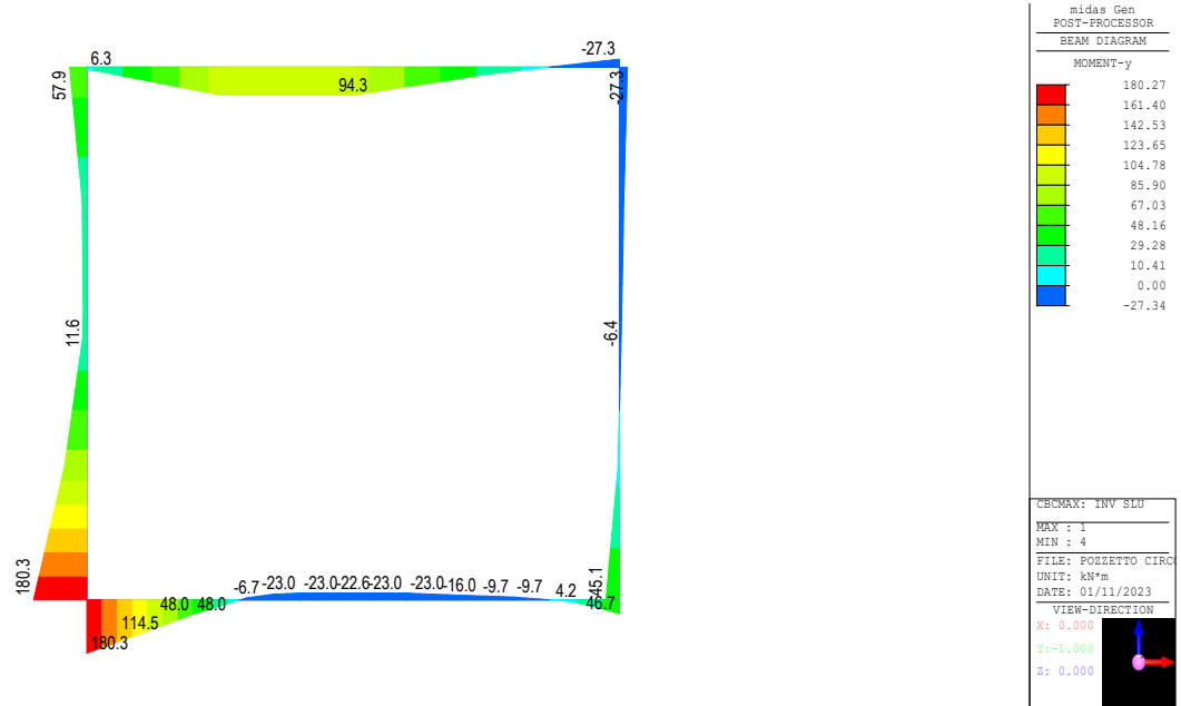
Fig. 7 – Involuppo momenti flettenti SLU
