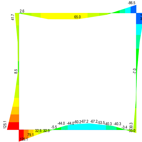
Fig. 13 – Involuppo momenti flettenti SLE rara
