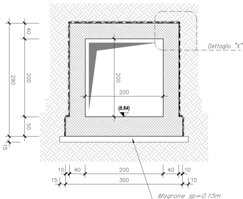
Fig. 2 – Sezione trasversale tipo
