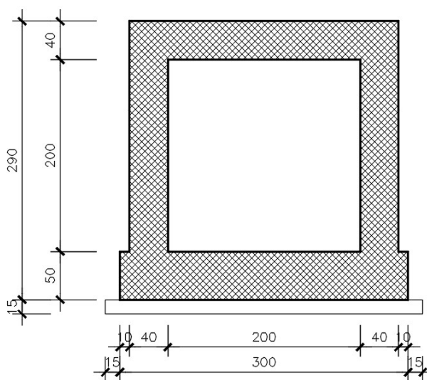
Fig. 6 – Stralcio Modello geometrico
