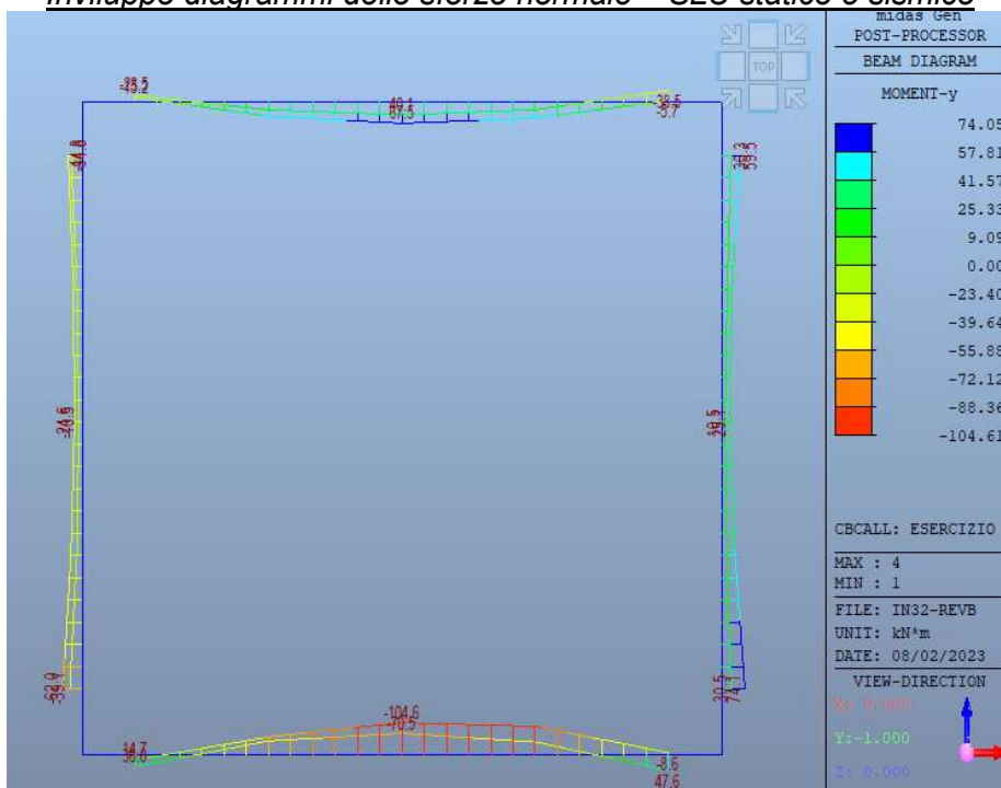
Involuppo diagrammi del momento flettente – SLE
