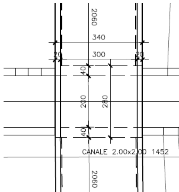
Fig. 2 – Pianta Scatolare stradale
