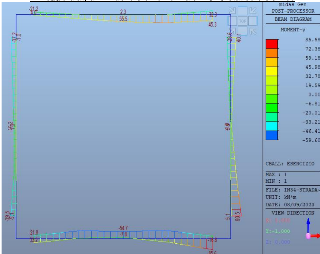
Involuppo diagrammi del momento flettente – SLE
