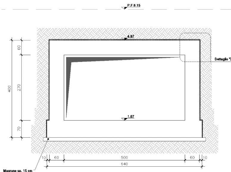
Fig. 2 – Sezione trasversale tipo
