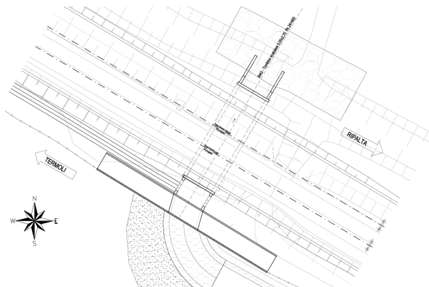
Fig. 1 – Inquadramento planimetrico
