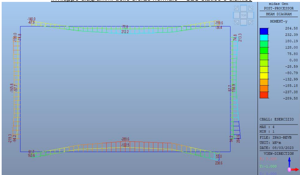
Inviluppo diagrammi del momento flettente – SLE
