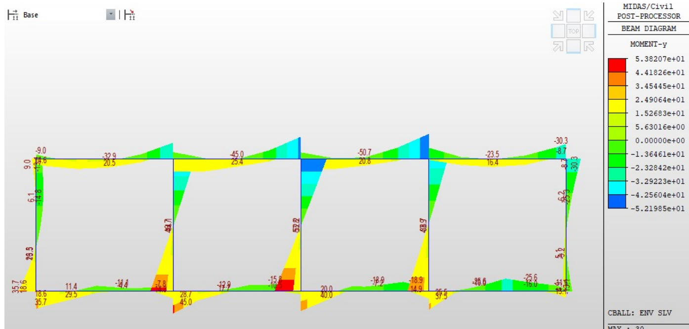
Fig. 30 – Involuppo momenti flettenti SLV
