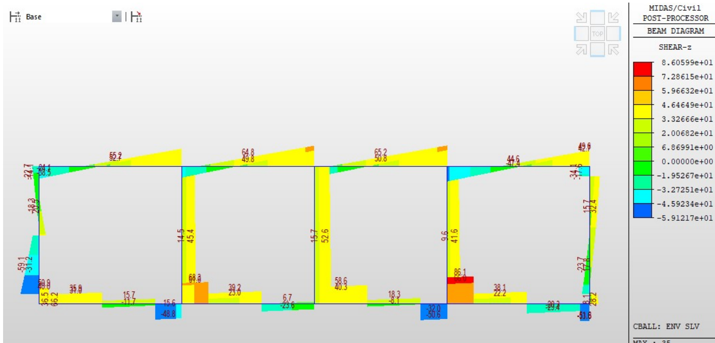
Fig. 31 – Involuppo sforzi taglienti SLV
