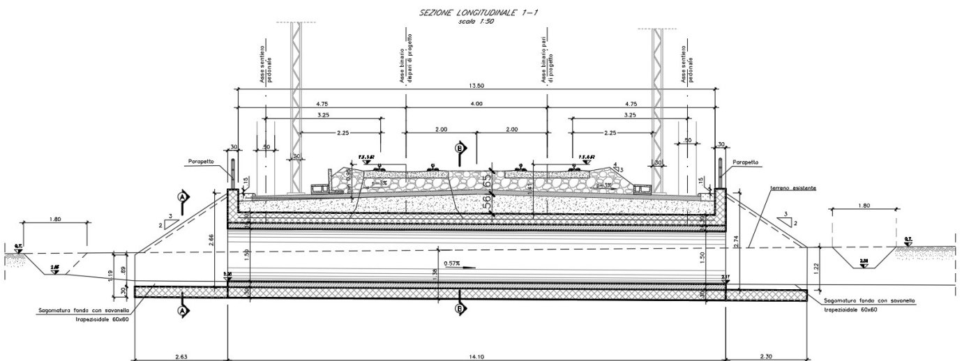
Fig. 2 – Sezione longitudinale
