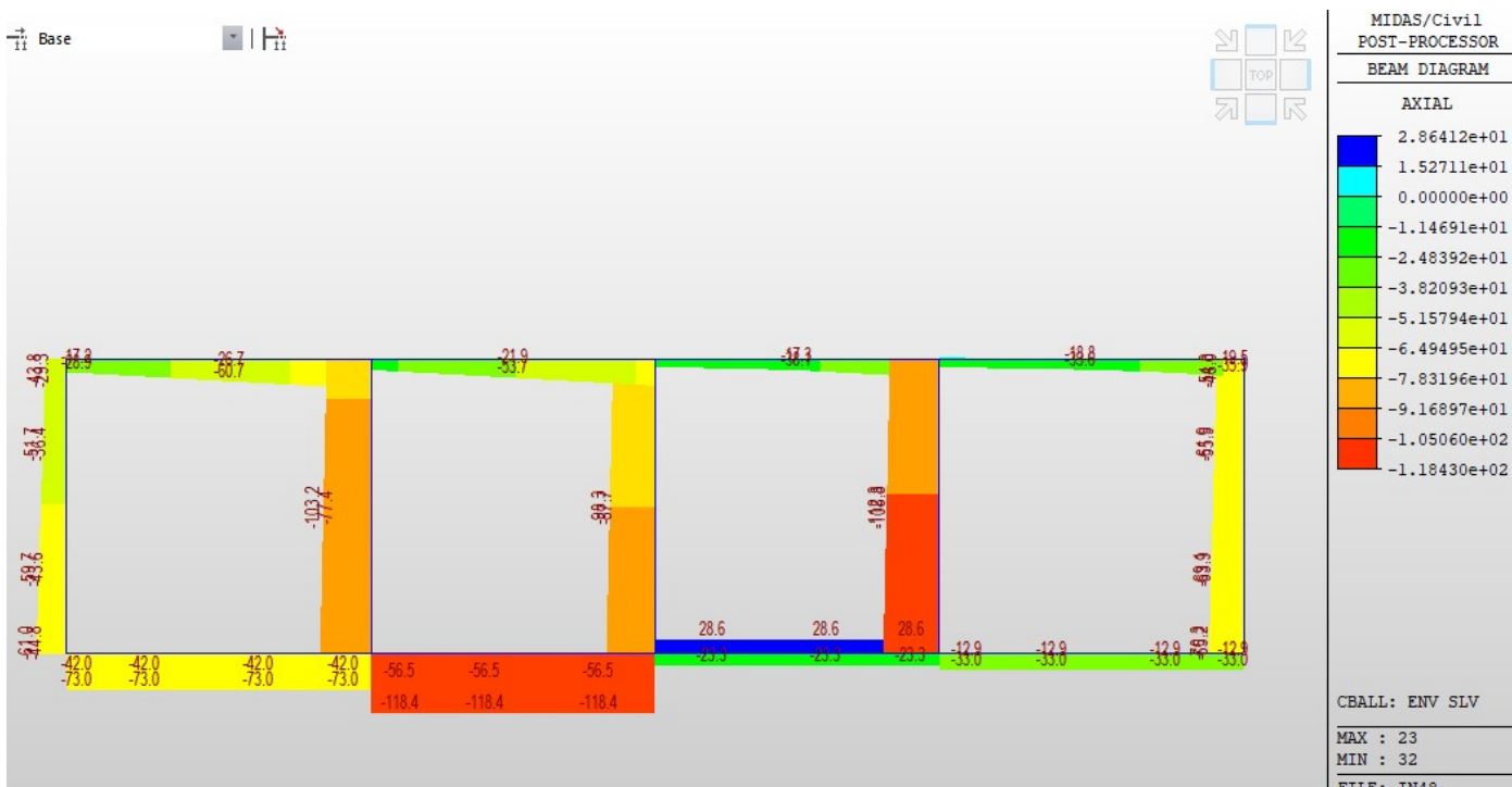
Fig. 32 – Involuppo azioni assiali SLV
