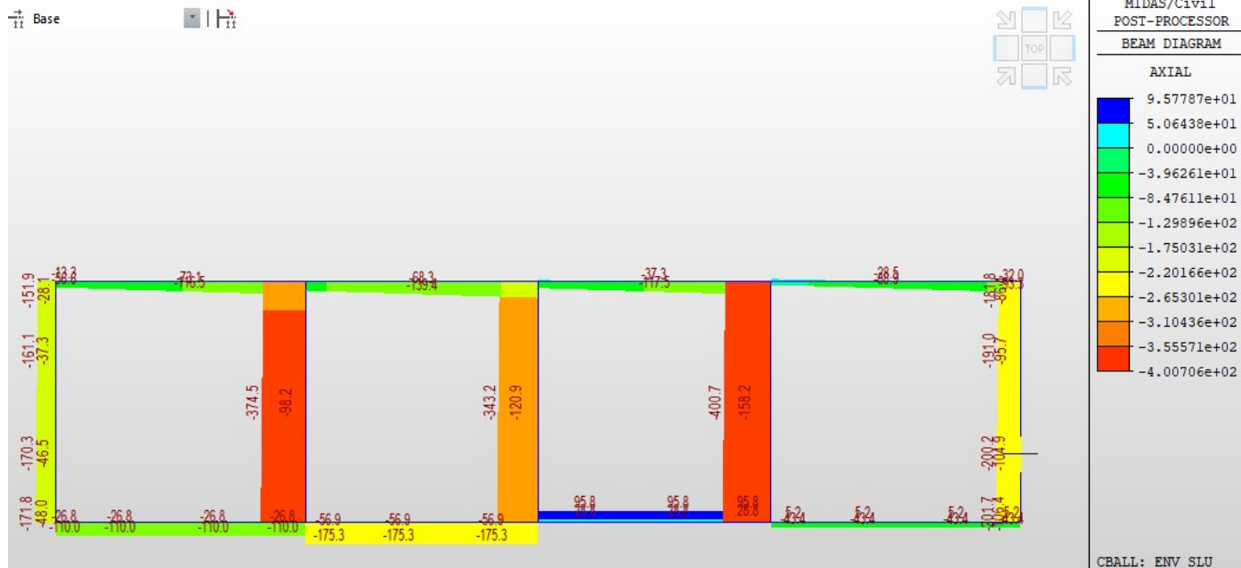
Fig. 29 – Involuppo azioni assiali SLU
