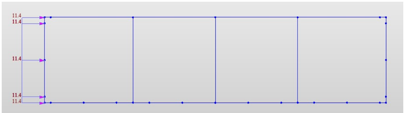
Fig. 16 – Spinta carico accidentale distribuito nel piedritto sinistro (simile per il piedritto destro) (SAS, SAD)
