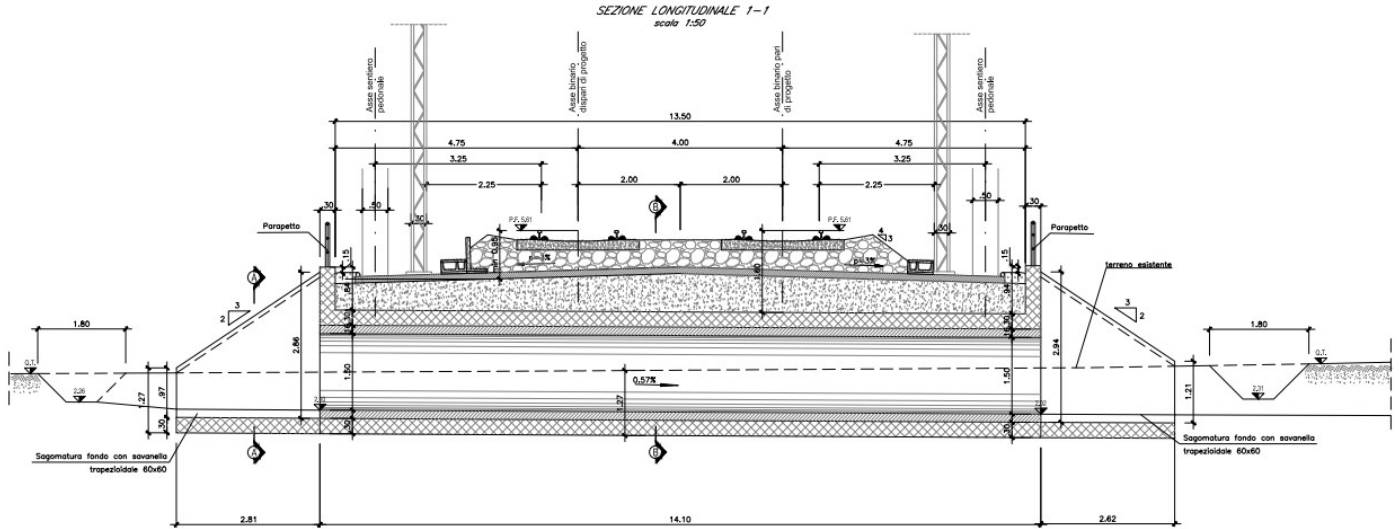
Fig. 2 – Sezione longitudinale
