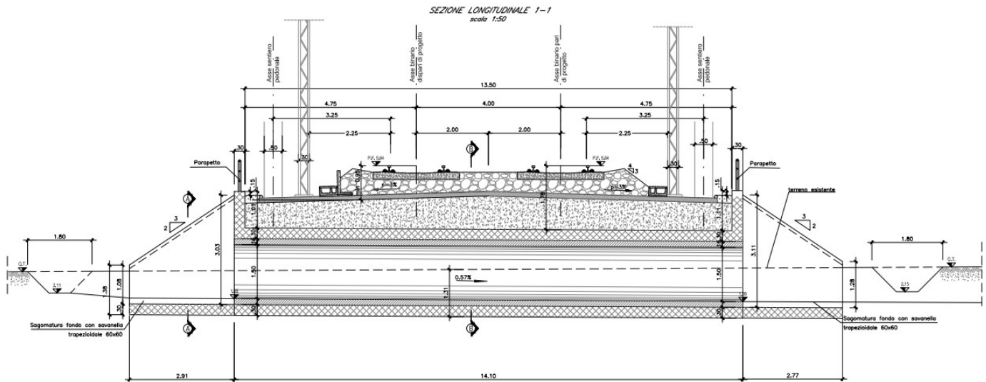
Fig. 2 – Sezione longitudinale
