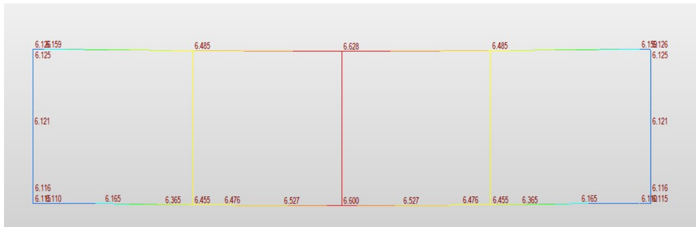
Fig. 35 – Deformazione
