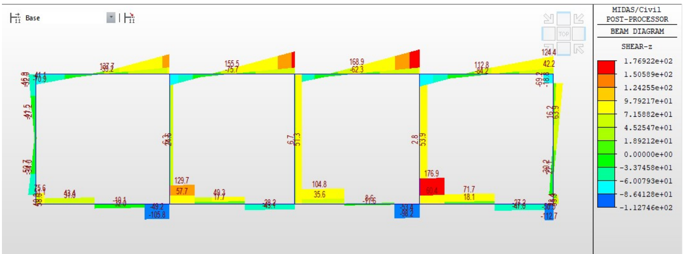
Fig. 34 – Involuppo sforzi taglianti RARA
