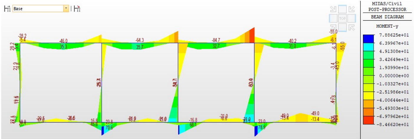
Fig. 33 – Involuppo momenti flettenti RARA
