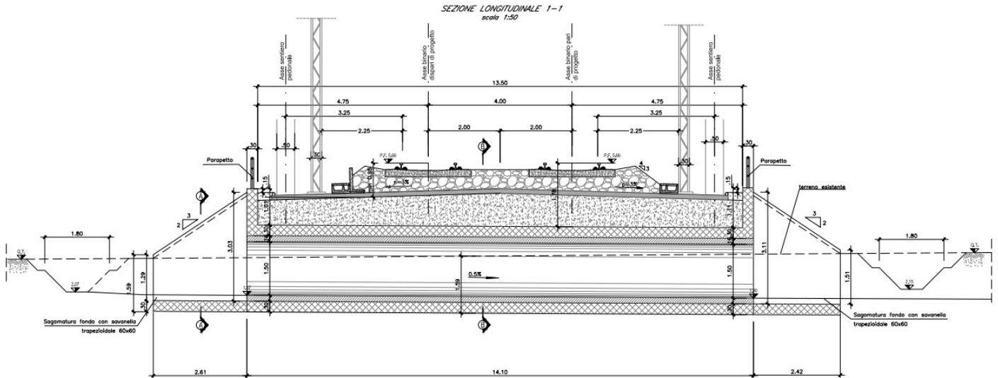
Fig. 2 – Sezione longitudinale
