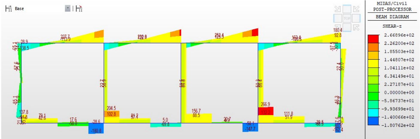
Fig. 28 – Involuppo sforzi taglienti SLU
