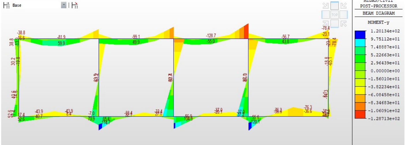
Fig. 27 – Involuppo momenti flettenti SLU
