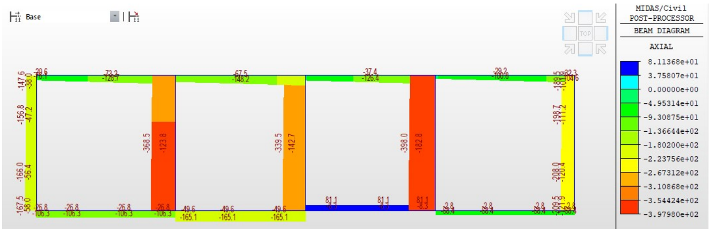
Fig. 29 – Involuppo azioni assiali SLU
