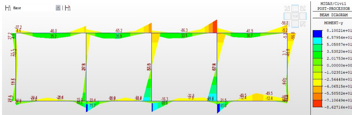
Fig. 33 – Involuppo momenti flettenti RARA
