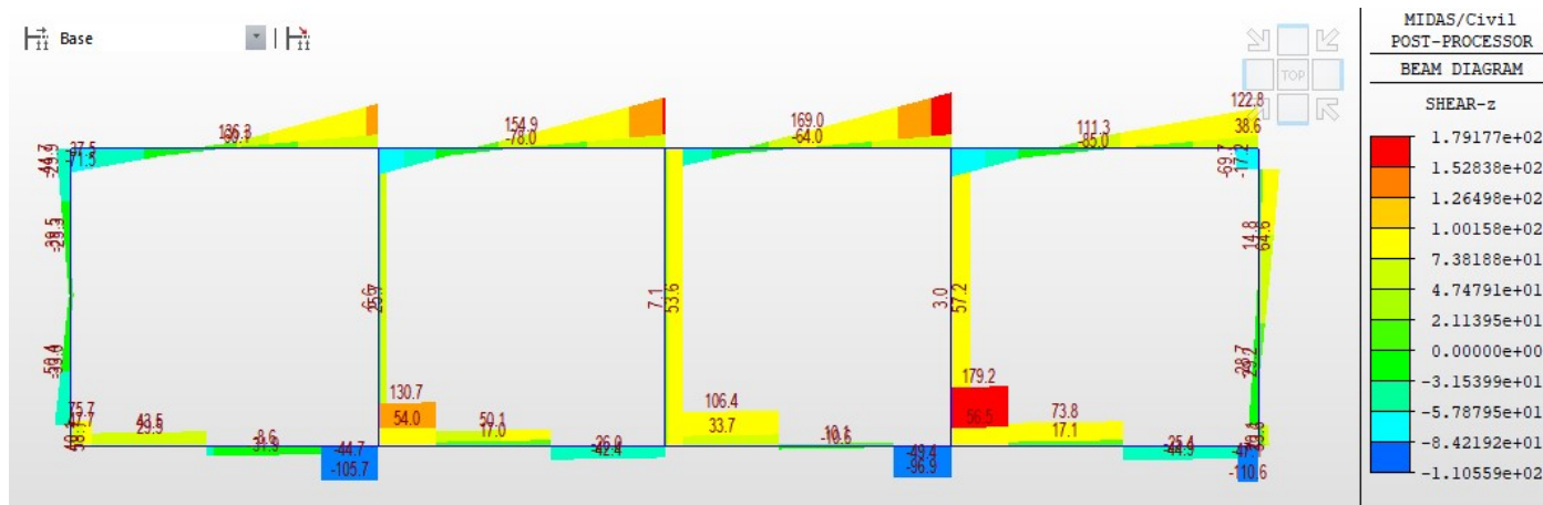
Fig. 34 – Involuppo sforzi taglianti RARA
