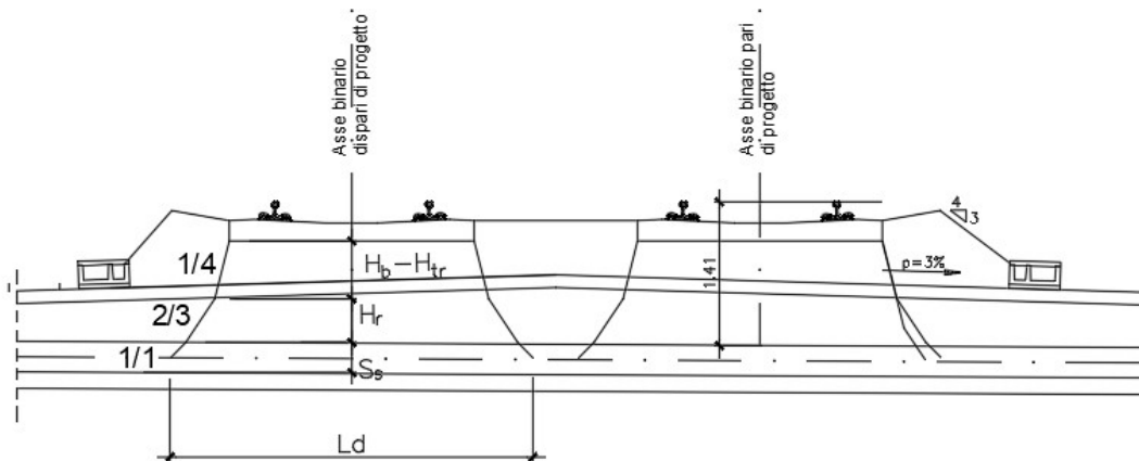
Fig. 13 – Diffusione del carico in senso trasversale
