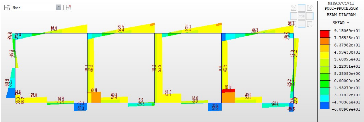
Fig. 31 – Involuppo sforzi taglienti SLV
