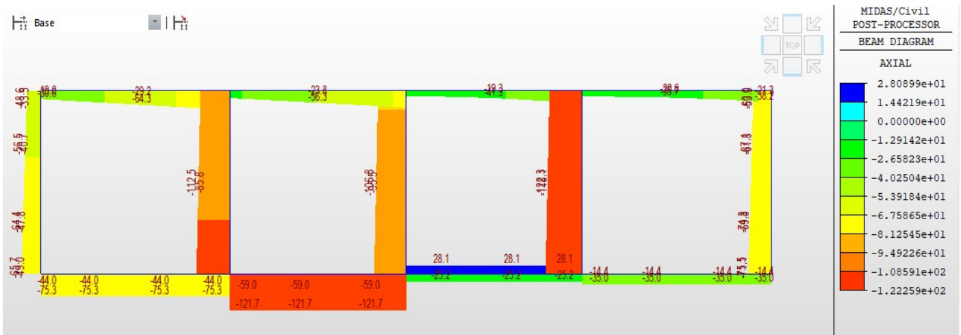
Fig. 32 – Involuppo azioni assiali SLV
