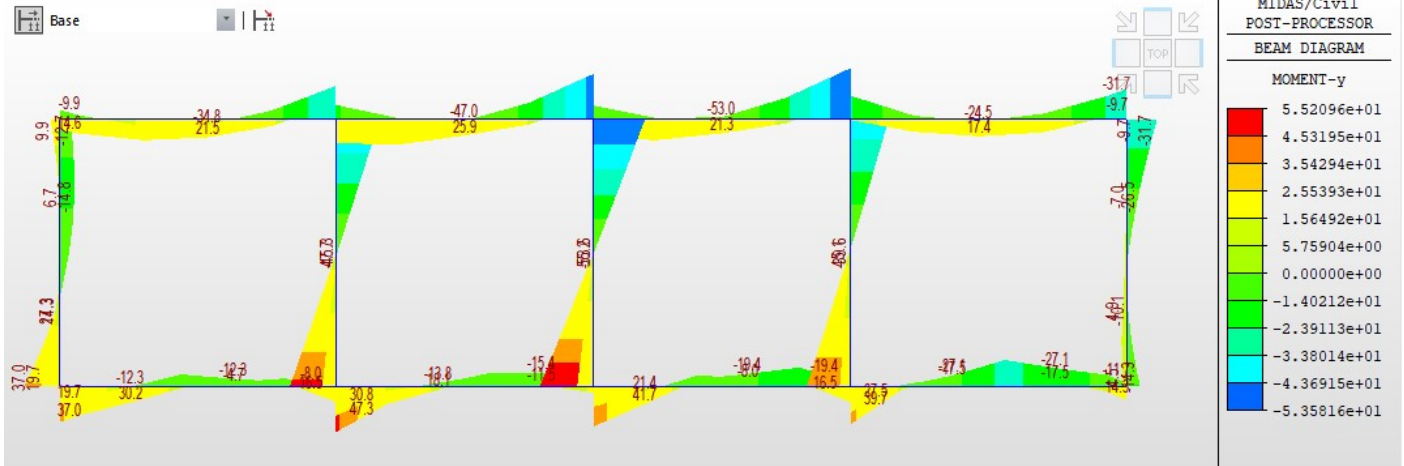
Fig. 30 – Involuppo momenti flettenti SLV
