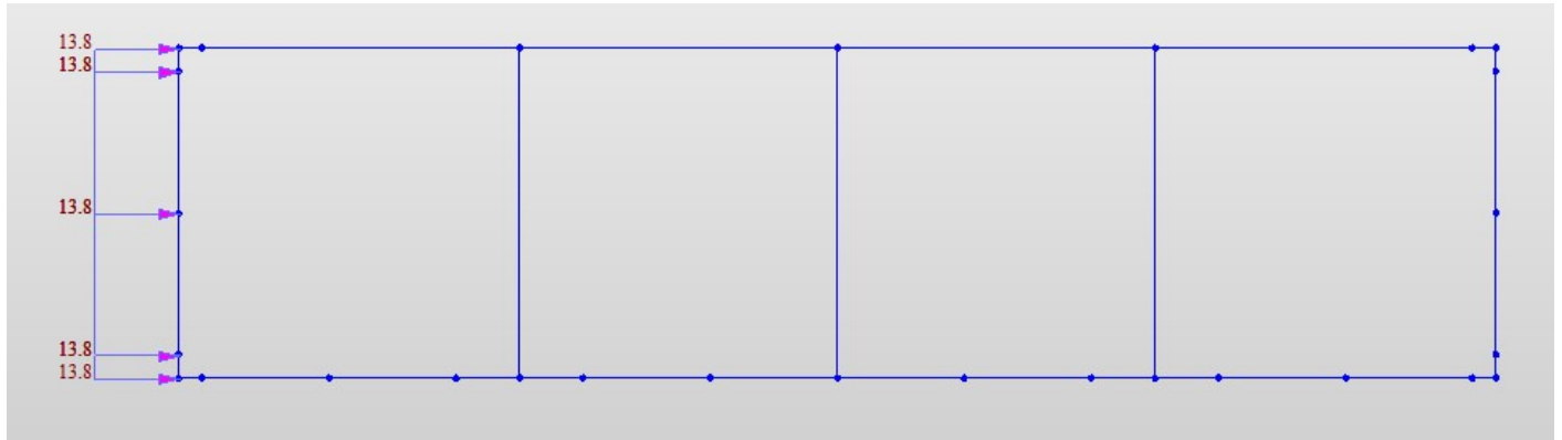
Fig. 23 – Sovraspinta sismica distribuite SISSX
