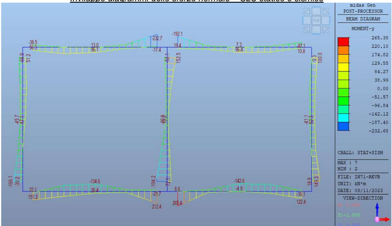
Inviluppo diagrammi del momento flettente – SLE
