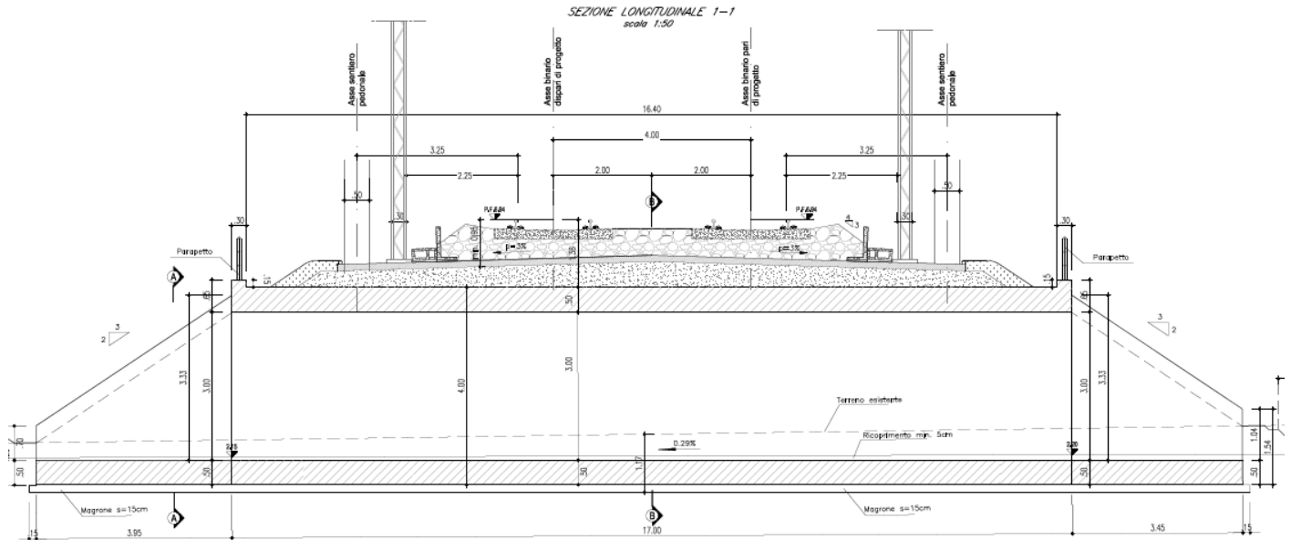
Fig. 3 – Sezione longitudinale
