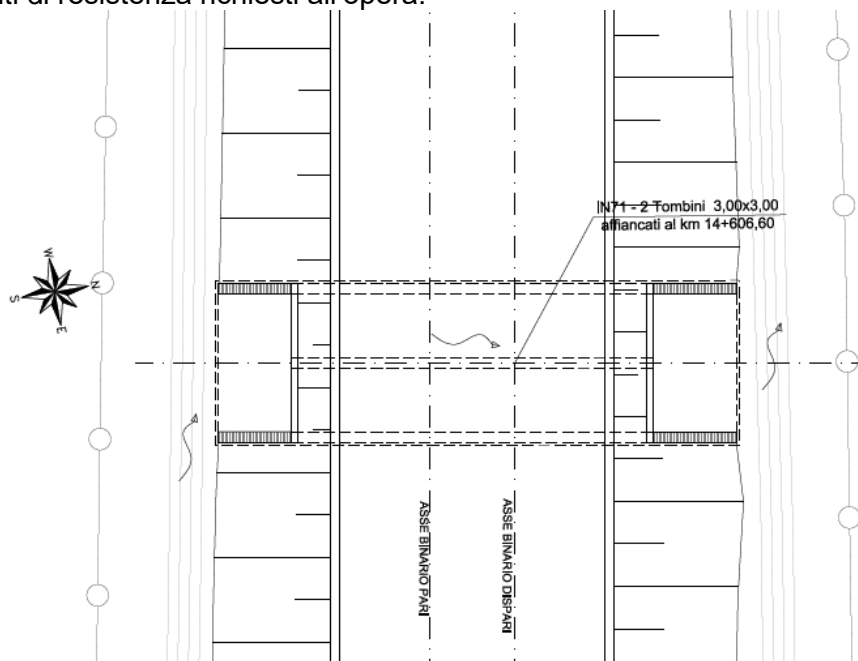
Fig. 1 – Inquadramento planimetrico
