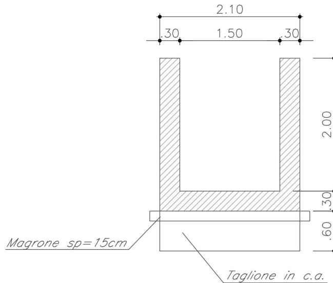
Figura 1 – Sezione trasversale
