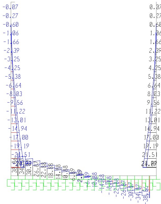
Fig. 2 – Involuppo sforzi taglianti SLU
