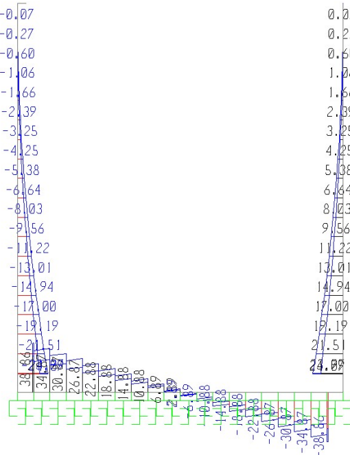
Fig. 2 – Involuppo sforzi taglienti SLU
