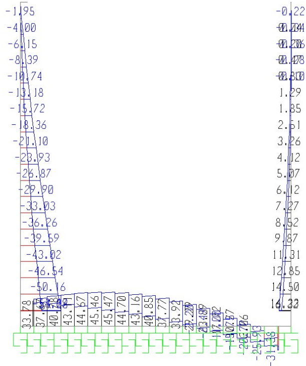
Fig. 5 – Involuppo sforzi taglianti SLV
