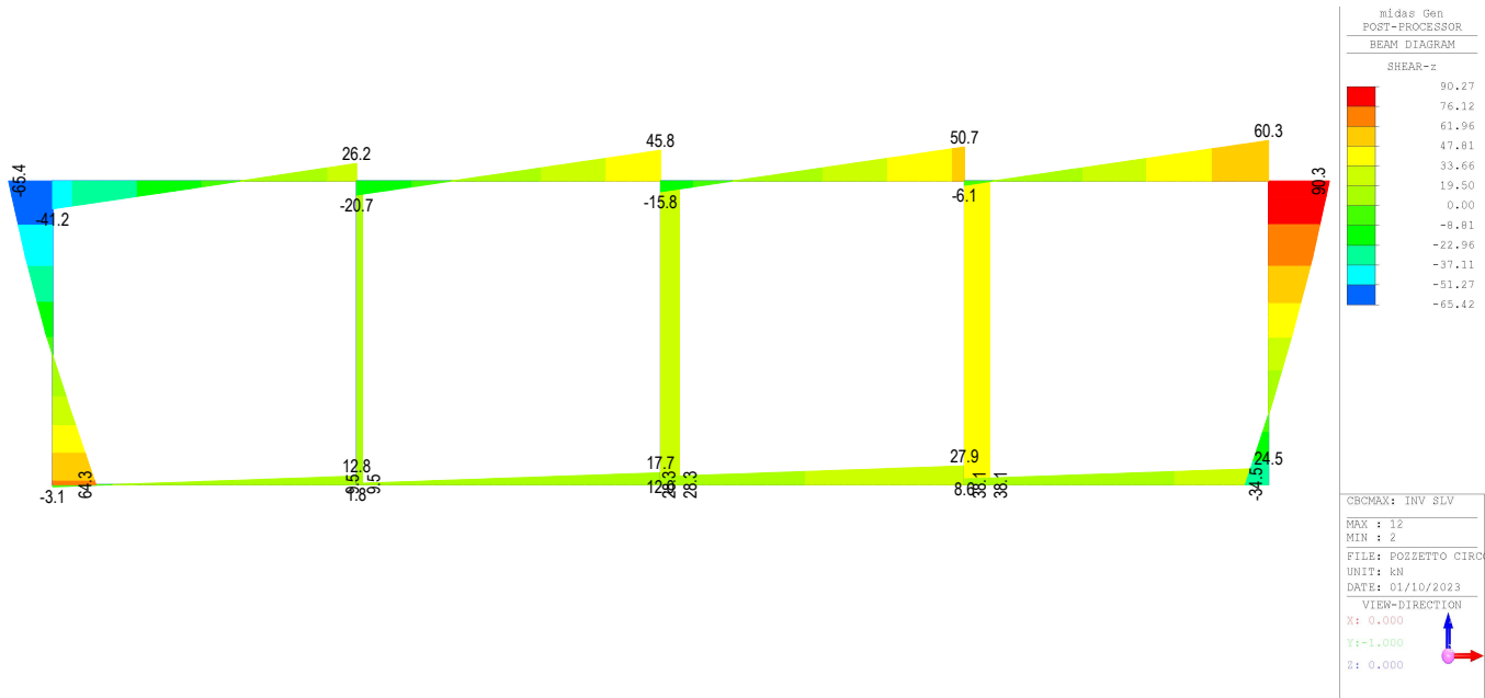
Fig. 11 – Inviluppo sforzi taglienti SLV
