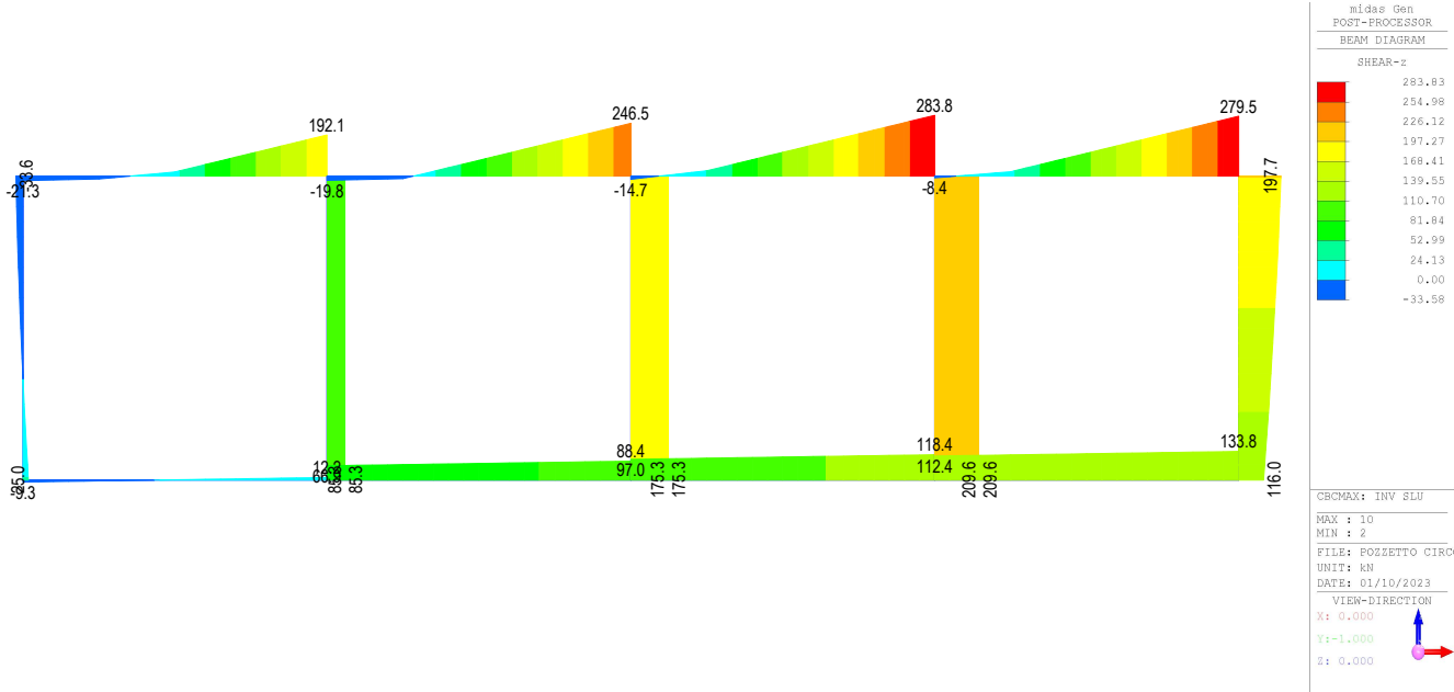
Fig. 8 – Involuppo sforzi taglienti SLU
