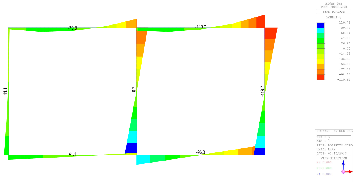
Fig. 13 – Involuppo momenti flettenti SLE rara
