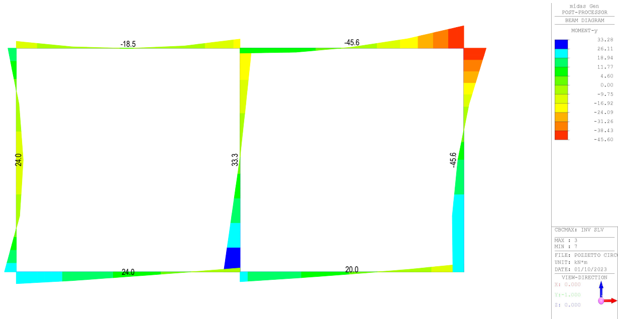
Fig. 10 – Involuppo momenti flettenti SLV
