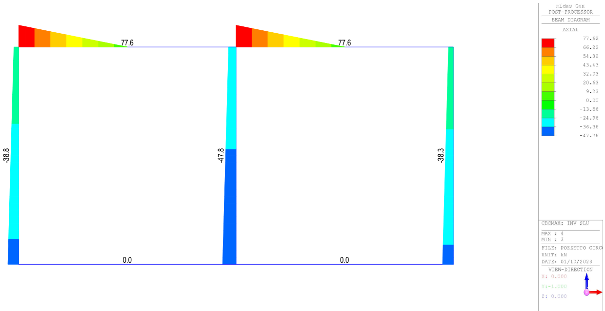
Fig. 9 – Involuppo azioni assiali SLU
