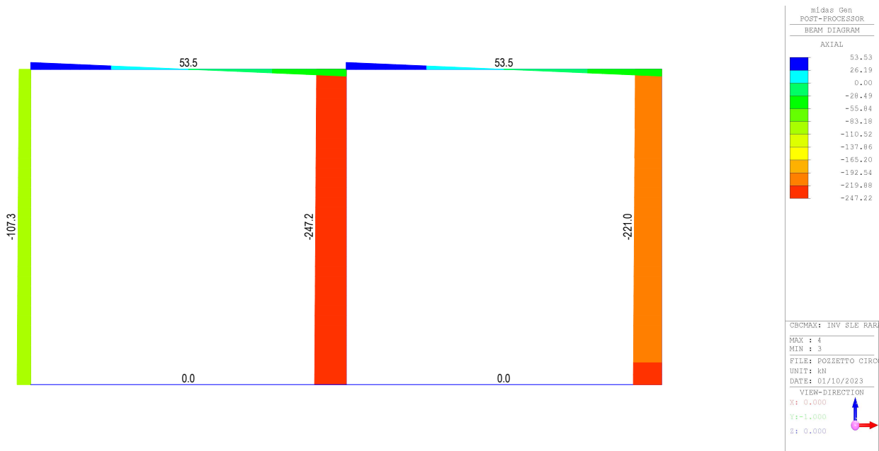
Fig. 14 – Involuppo azioni assiali SLE rara
