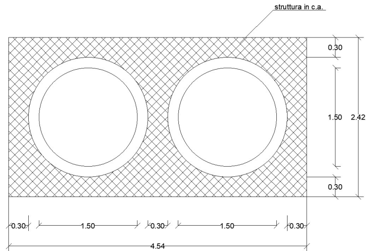
Figura 1: Sezione trasversale dell'opera
