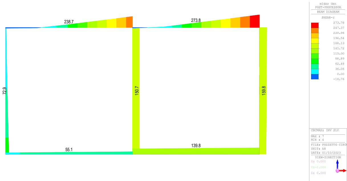
Fig. 8 – Involuppo sforzi taglianti SLU
