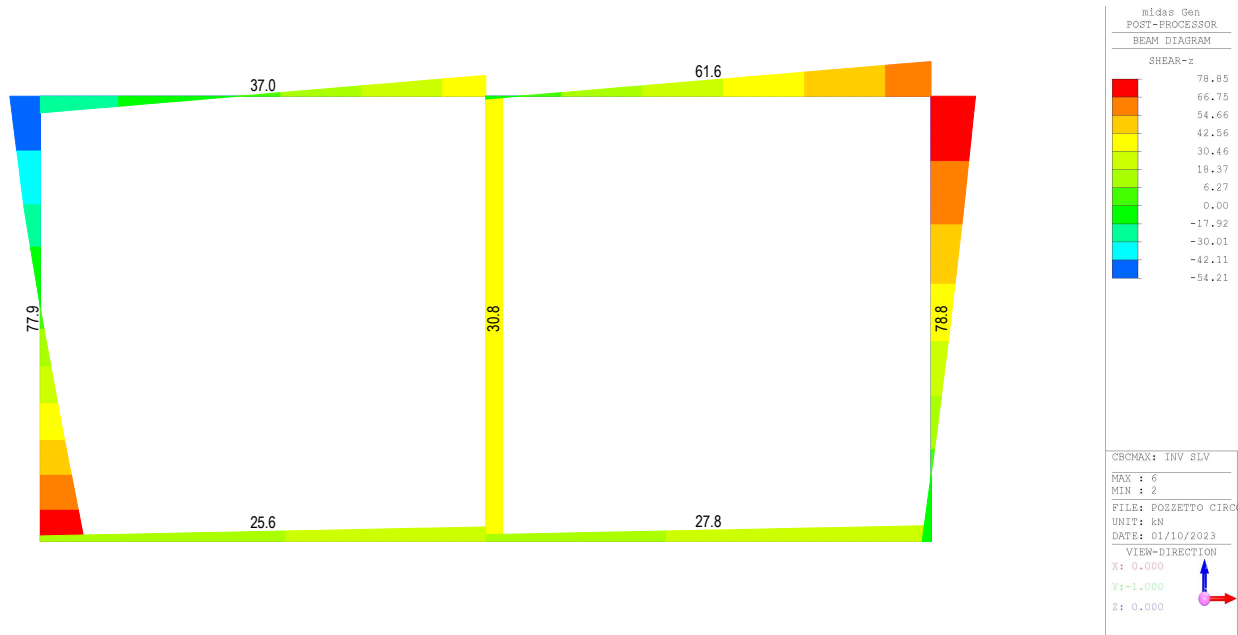
Fig. 11 – Inviluppo sforzi taglianti SLV
