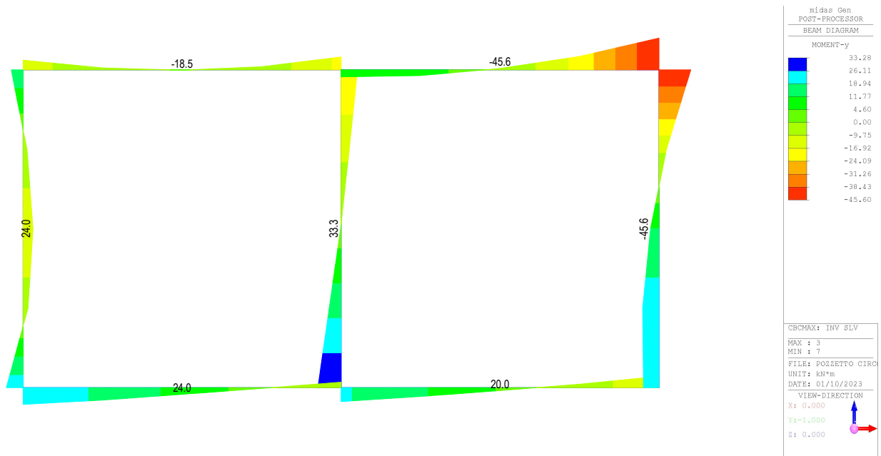
Fig. 10 – Involuppo momenti flettenti SLV
