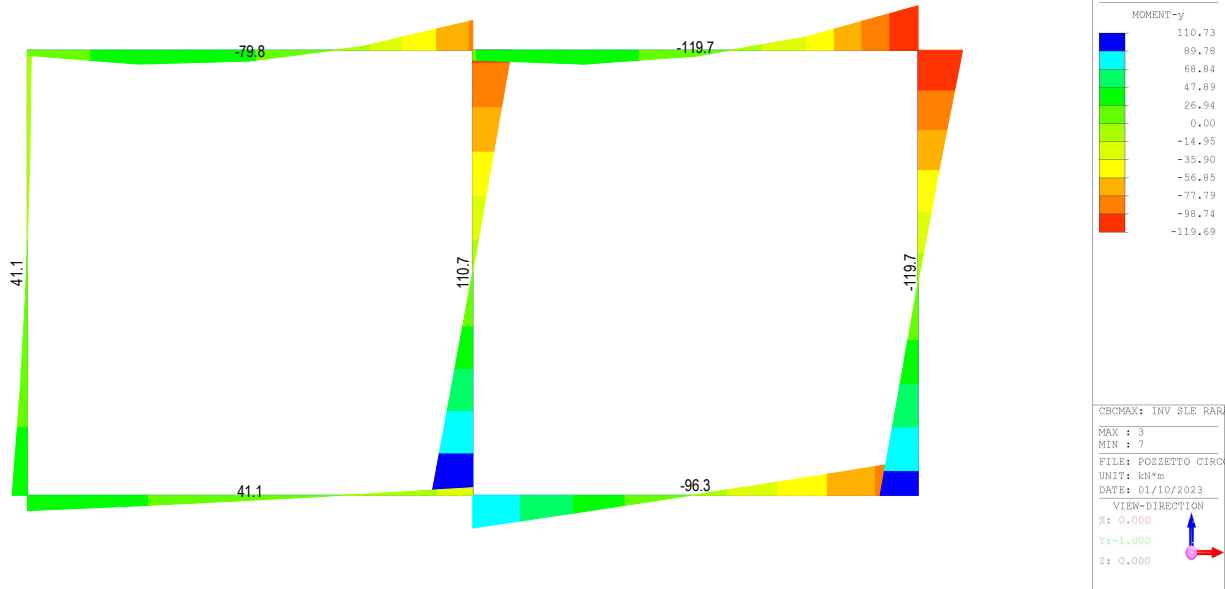
Fig. 13 – Involuppo momenti flettenti SLE rara
