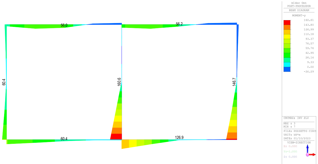
Fig. 7 – Involuppo momenti flettenti SLU
