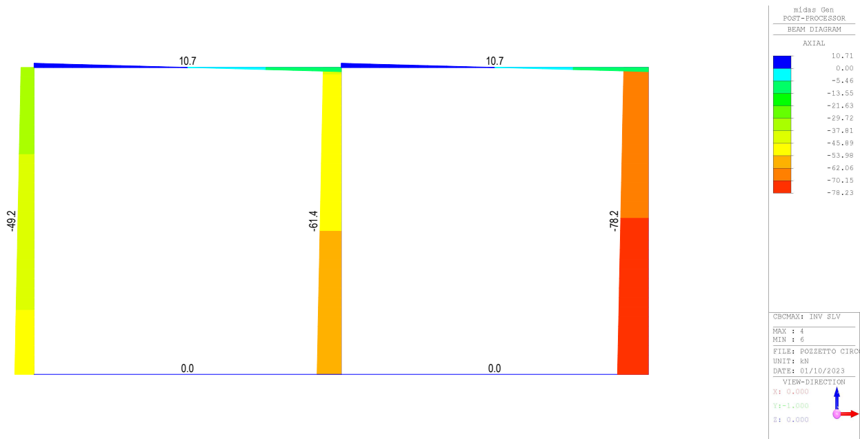
Fig. 12 – Inviluppo azioni assiali SLV
