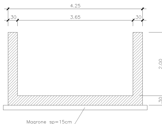
Figura 1: Sezione trasversale
