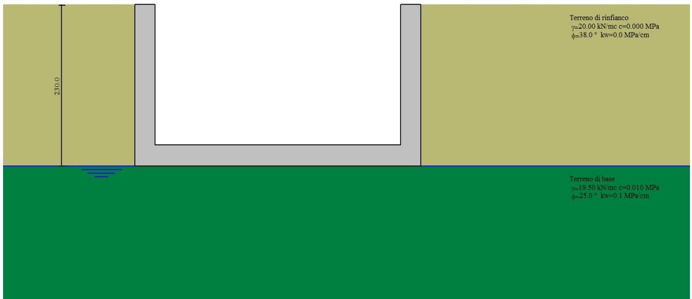
Figura 3: Modello Geometrico Geotecnico di Riferimento – 1/2
