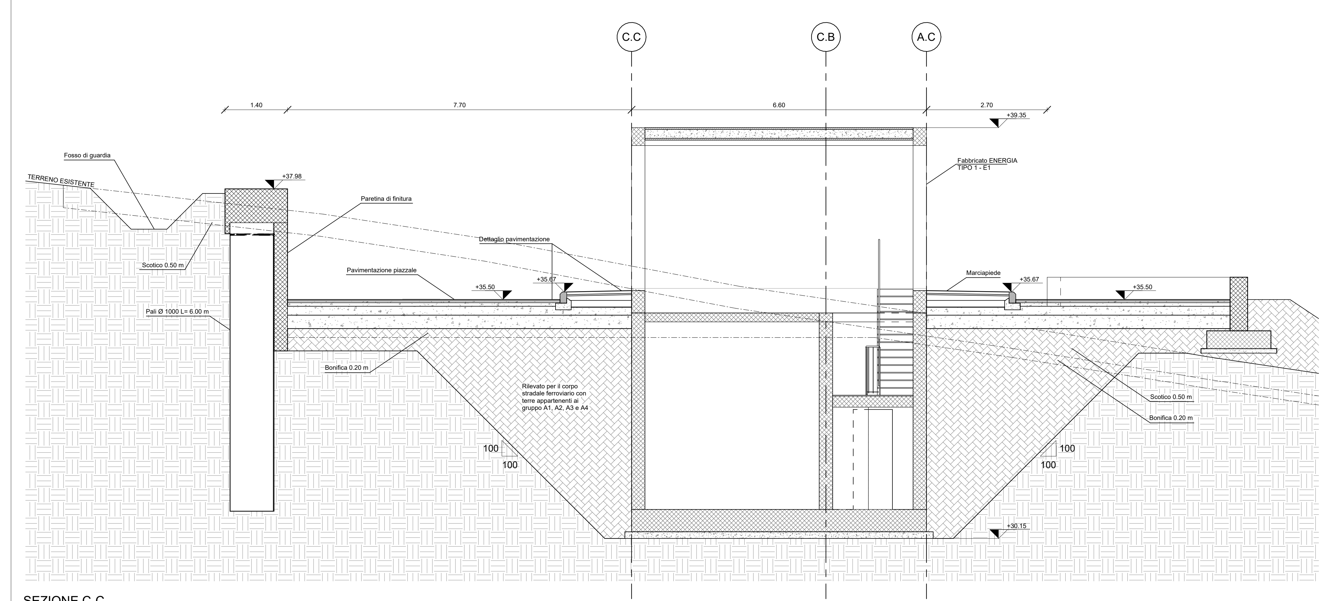
SEZIONE C-C 1 : 50
