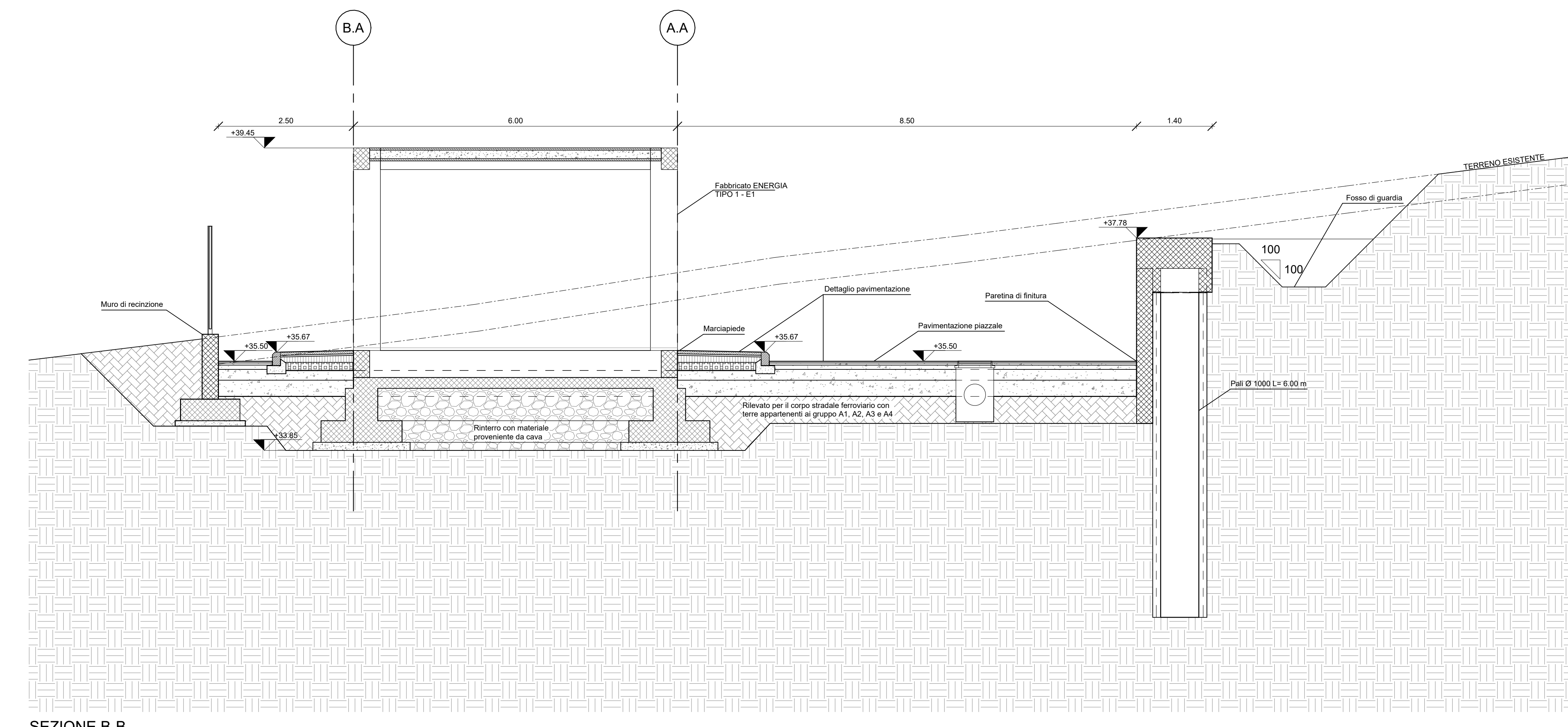
SEZIONE B-B 1 : 50
