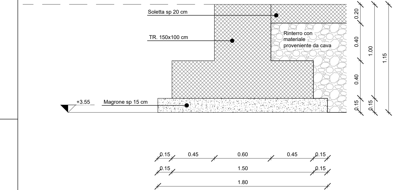
DETTAGLIO S1 - PARTICOLARE FONDAZIONE 1 : 20
