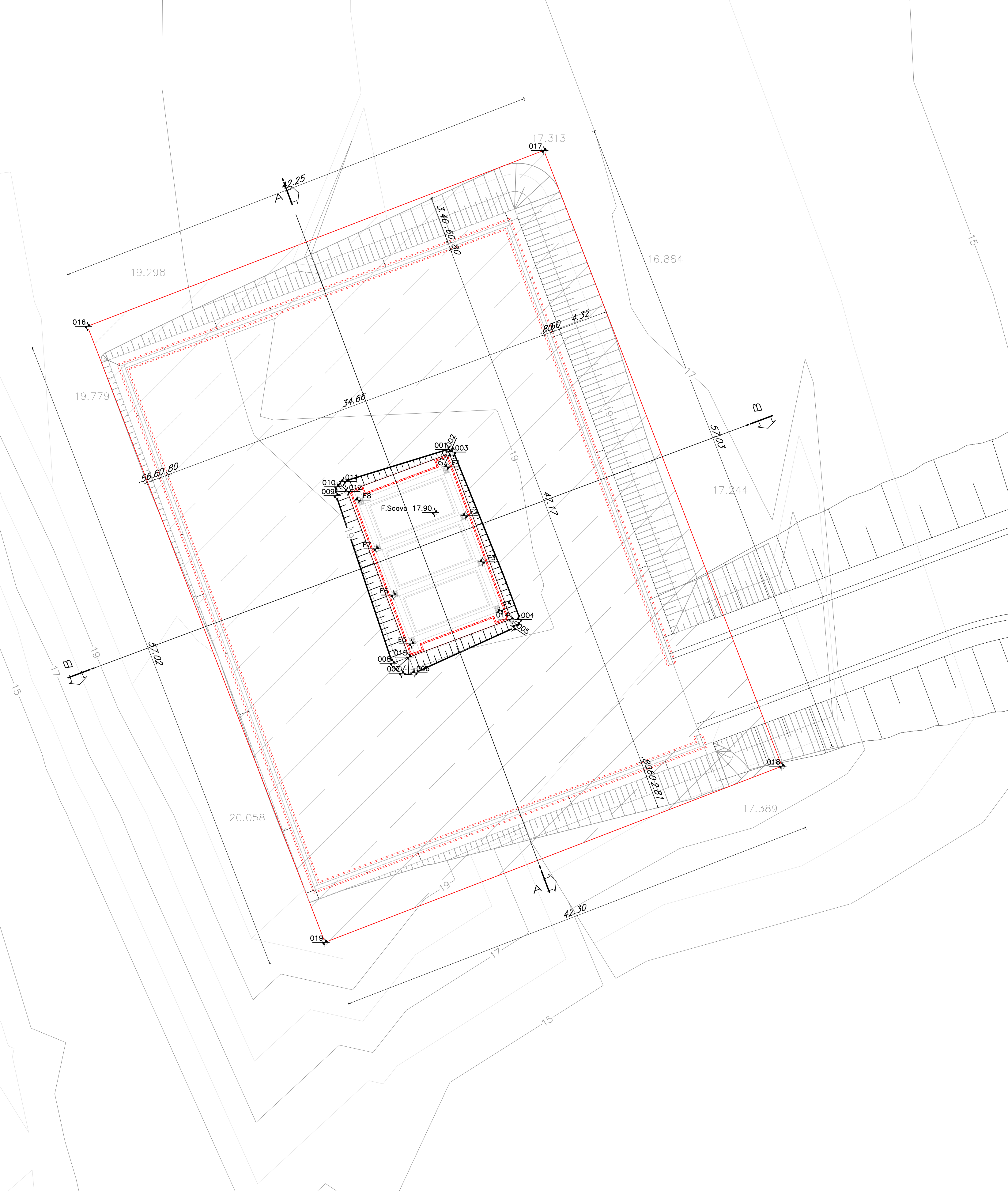
PIANTA SCAVI - SCALA 1:200
