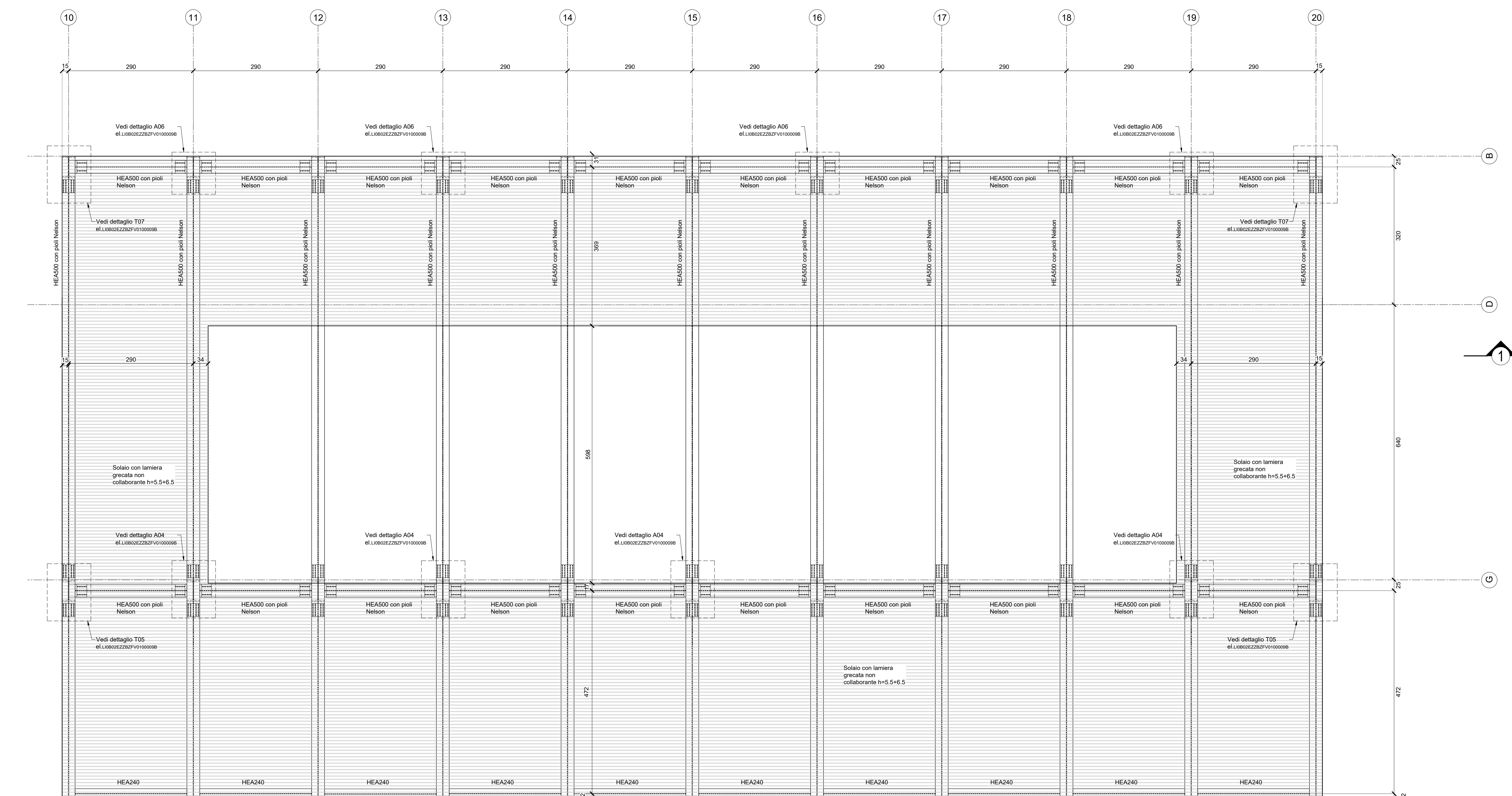
PIANTA "A-A" Scala 1:50
