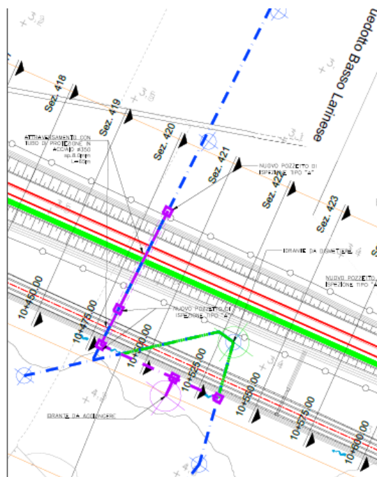
Figura 5-4 Stralcio risoluzione interferenze INT68 e INT69
