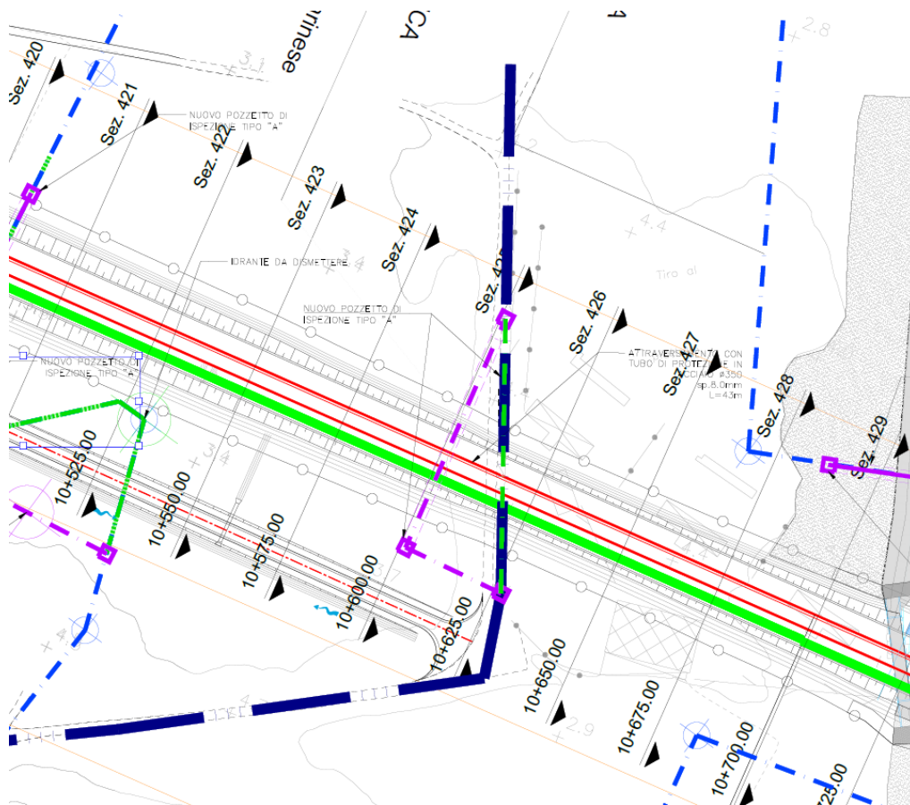
Figura 5-5 Stralcio risoluzione interferenze INT68, INT69 e INT106
