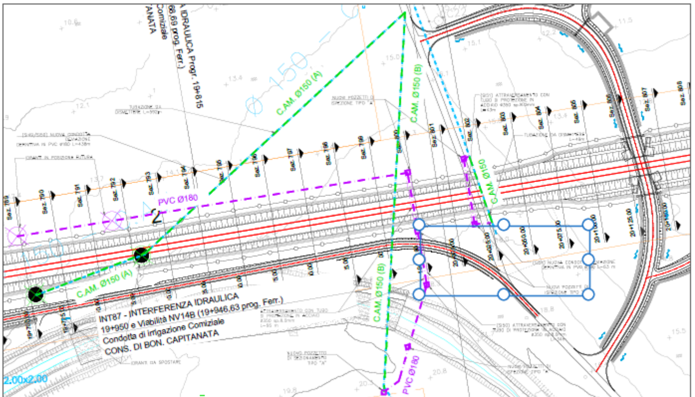
Figura 5-1. Stralcio risoluzione interferenze INT86, INT87 e INT88
