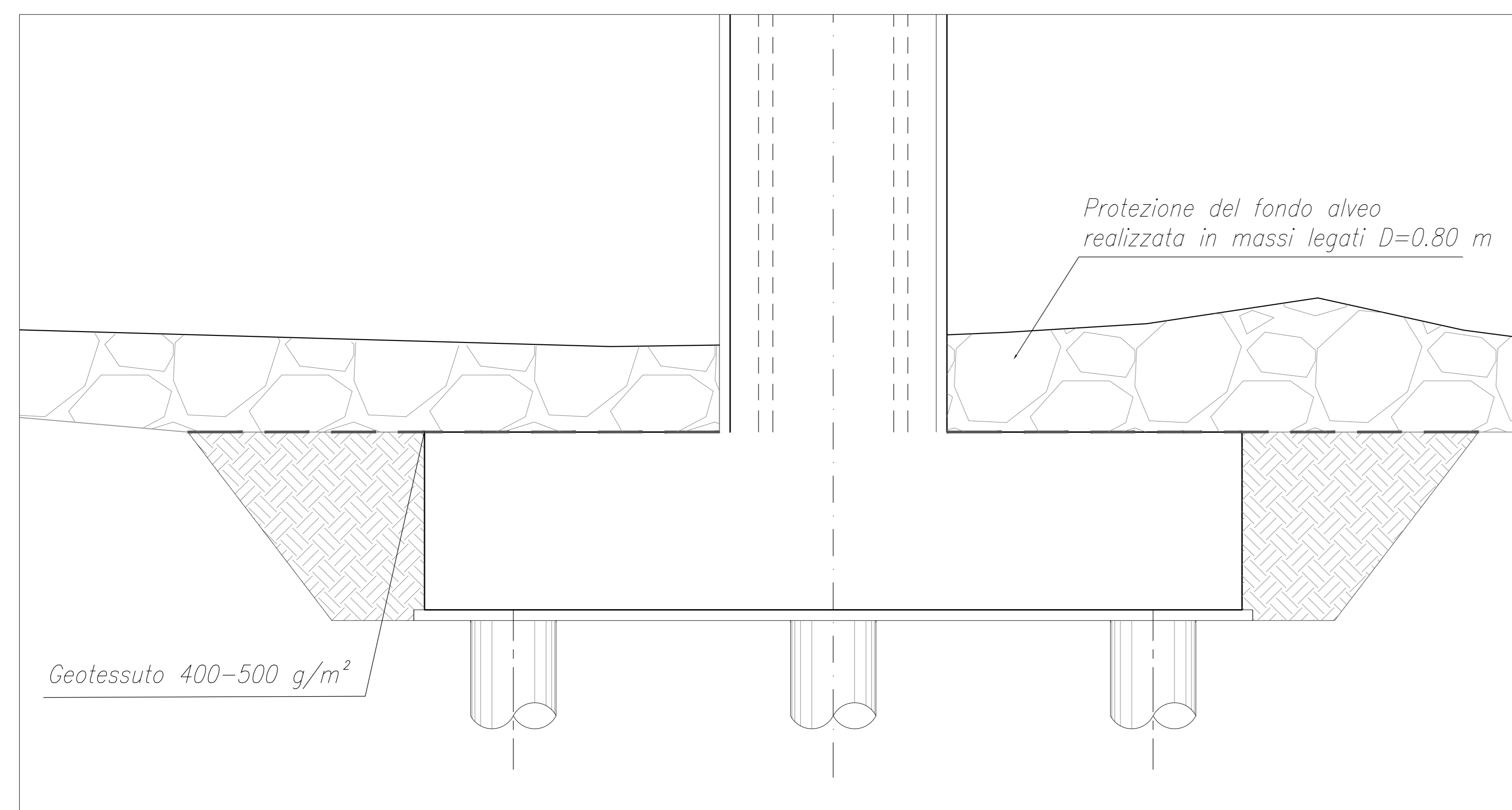
POSA DEI MASSI IN PROSSIMITA' DELLE PILE Scala: 1:50
