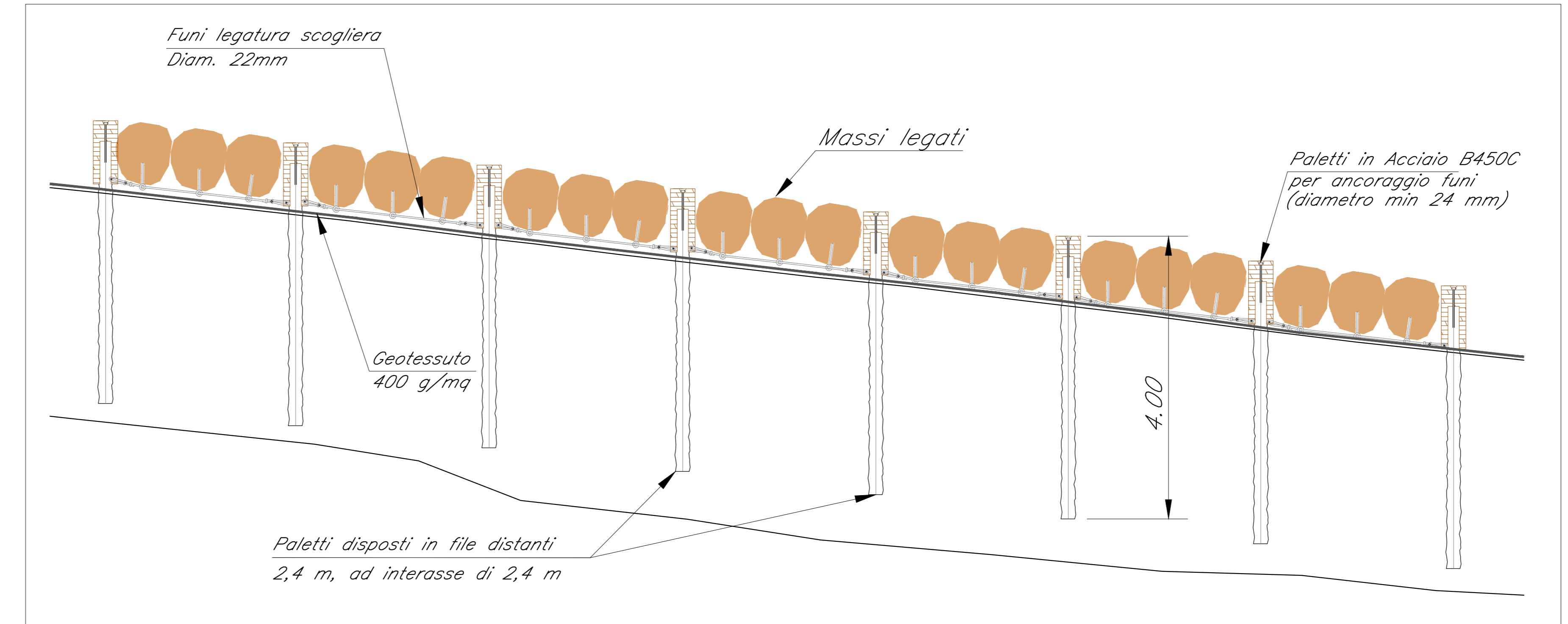
PARTICOLARE FISSAGGIO DEI MASSI Scala: 1:50
