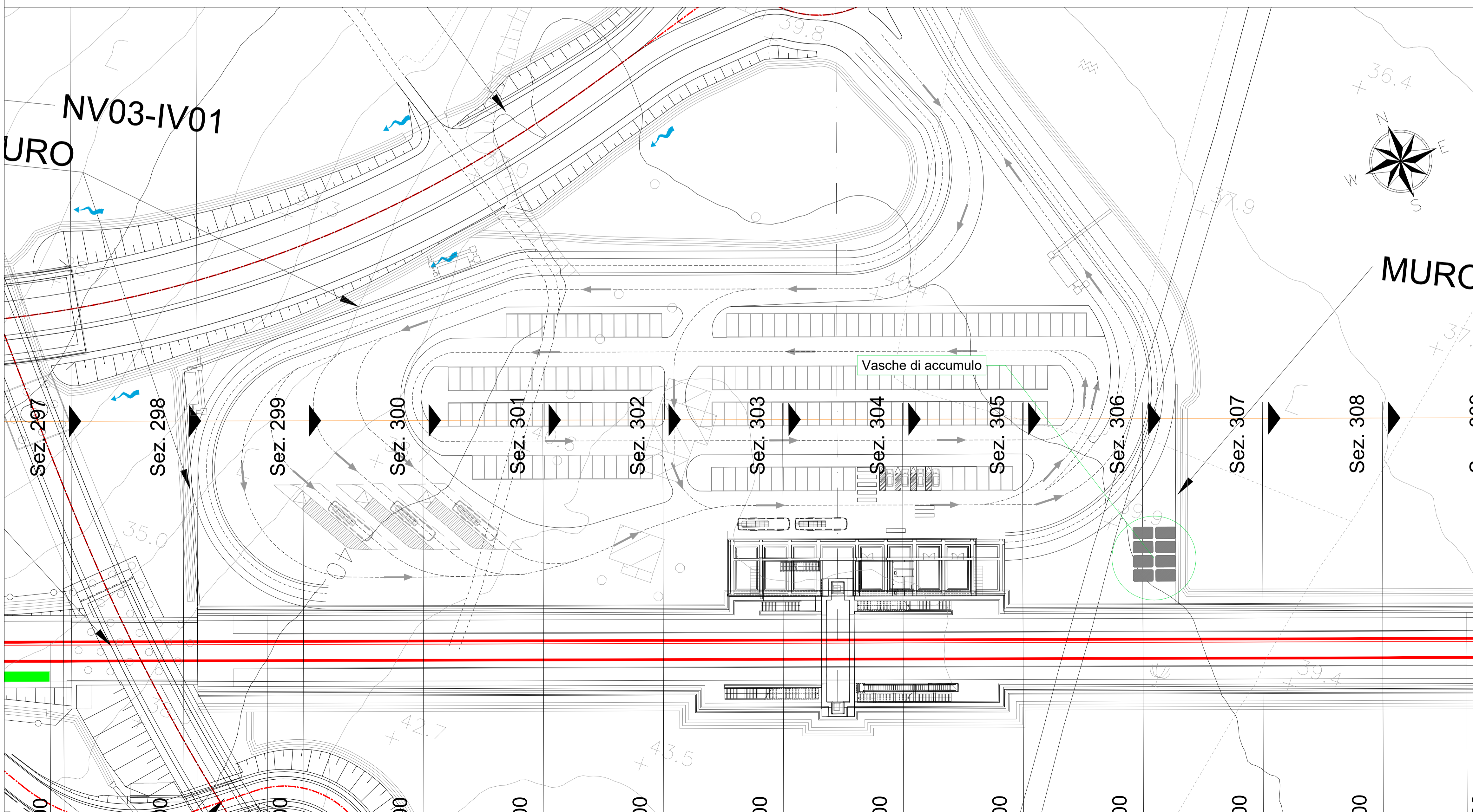
INQUADRAMENTO – SCALA 1:500
