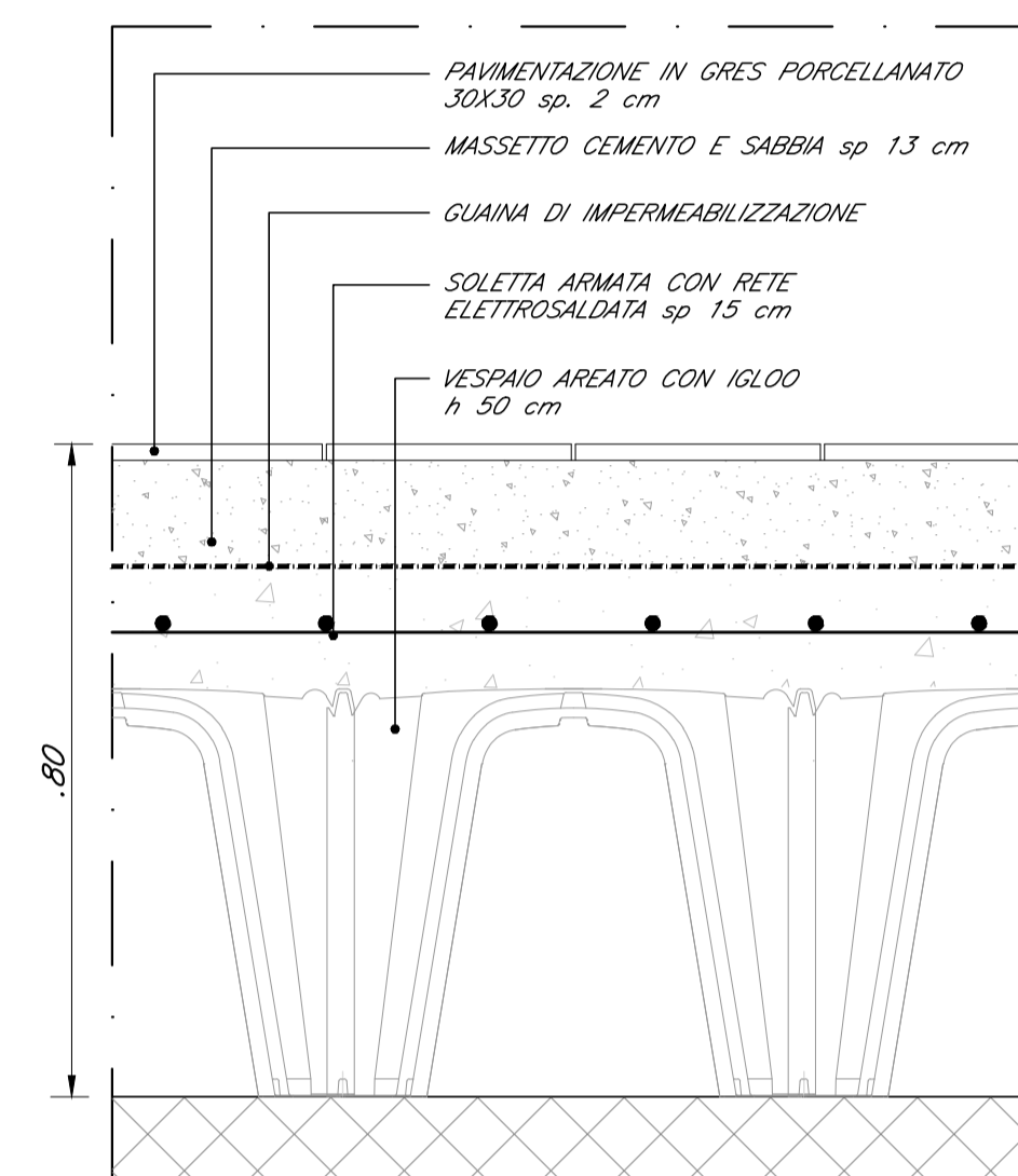
DETTAGLIO 27 PAVIMENTAZIONE BANCHINA IN GRES PORCELLANATO SCALA 1:10
