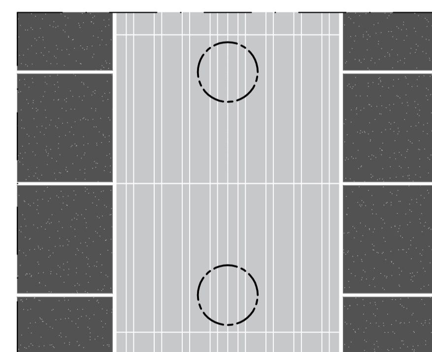
DETTAGLIO 23 B8 PAVIMENTO IN GRES FINE PORCELLANATO SISTEMA LVE SCALA 1:10
