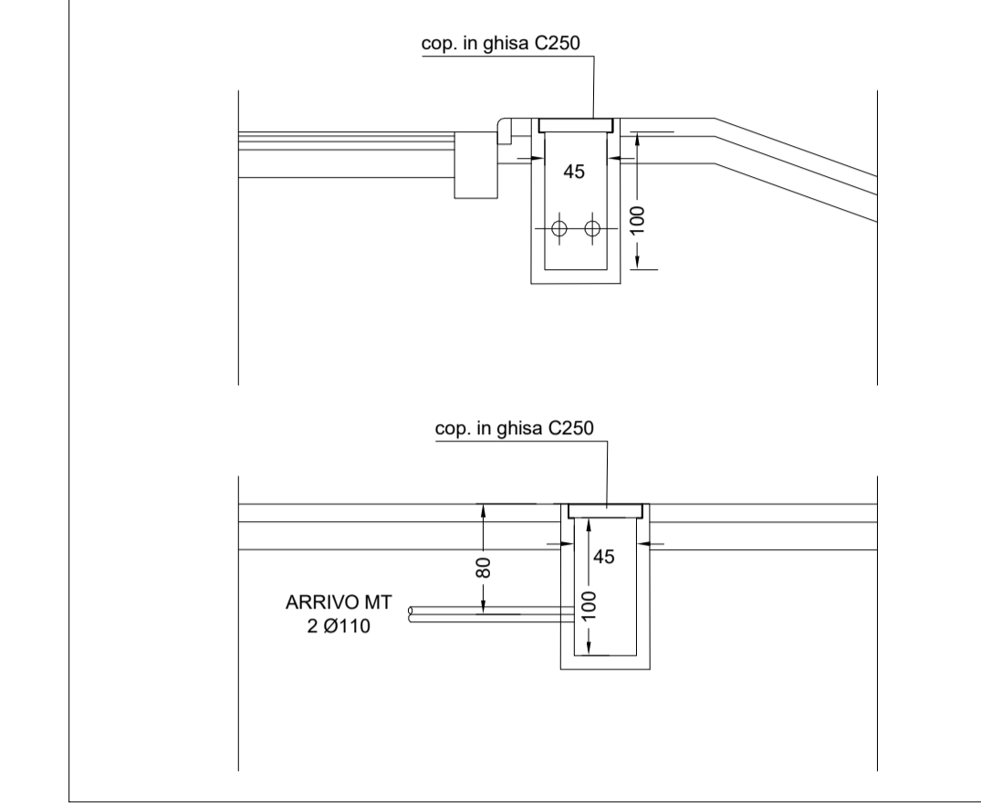
DETTAGLI DI COLLEGAMENTO TUBAZIONI INTERRATE
