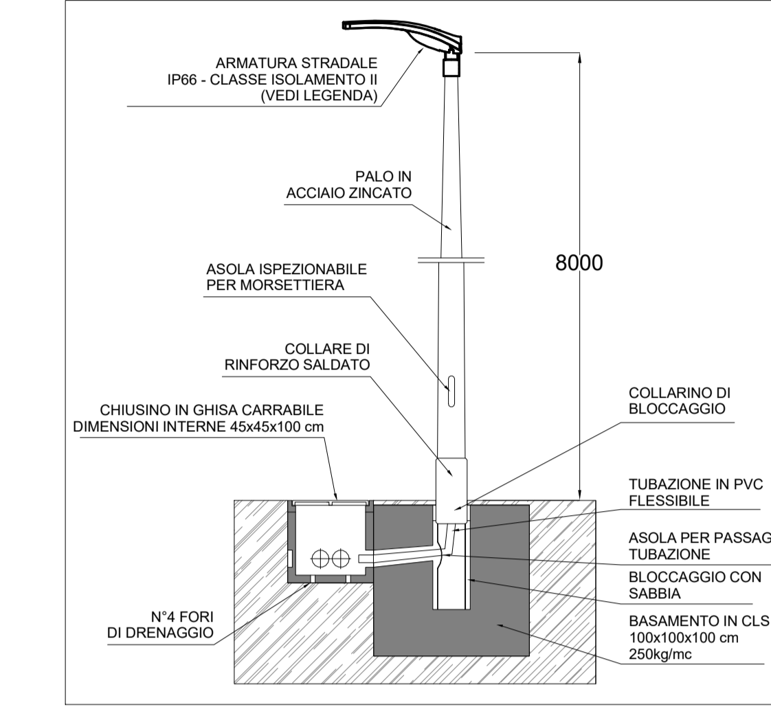
DETTAGLIO INSTALLAZIONE PROIETTORE SU PALO
