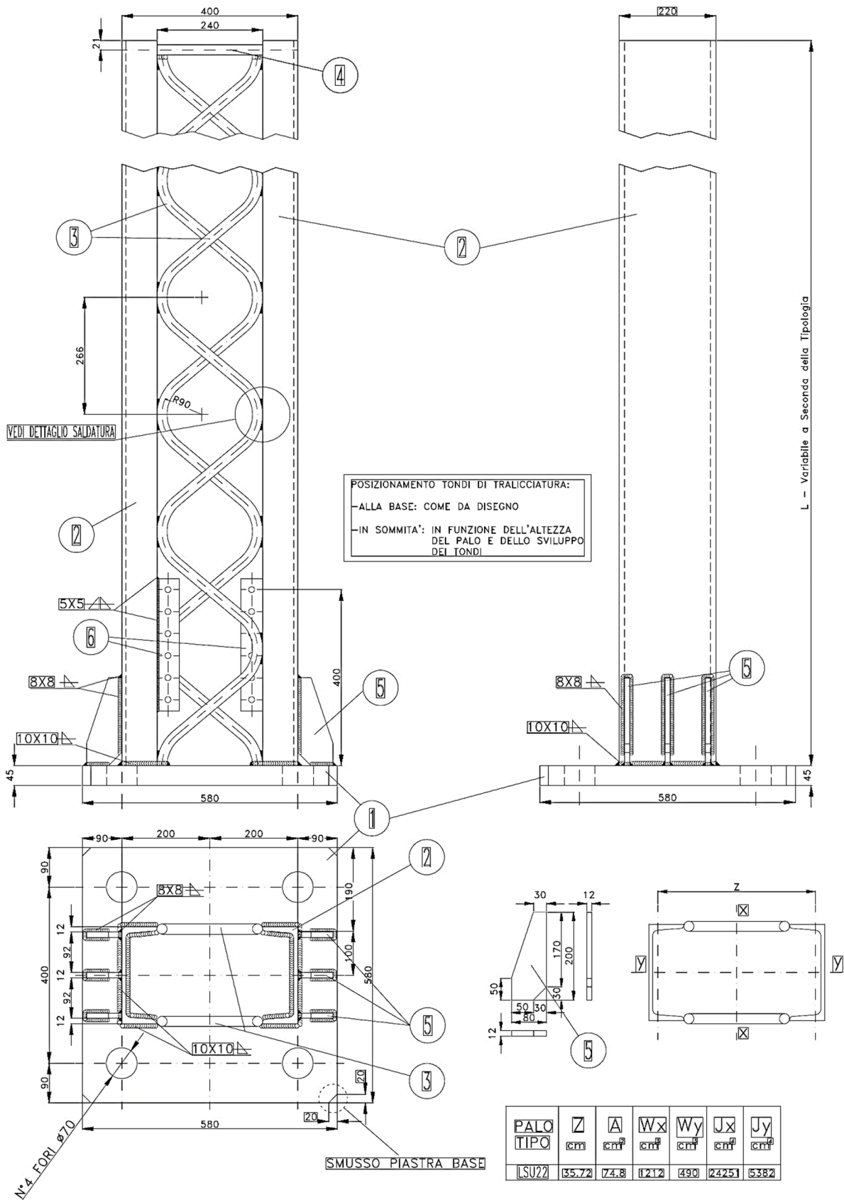
Particolari palo tipo LSU
