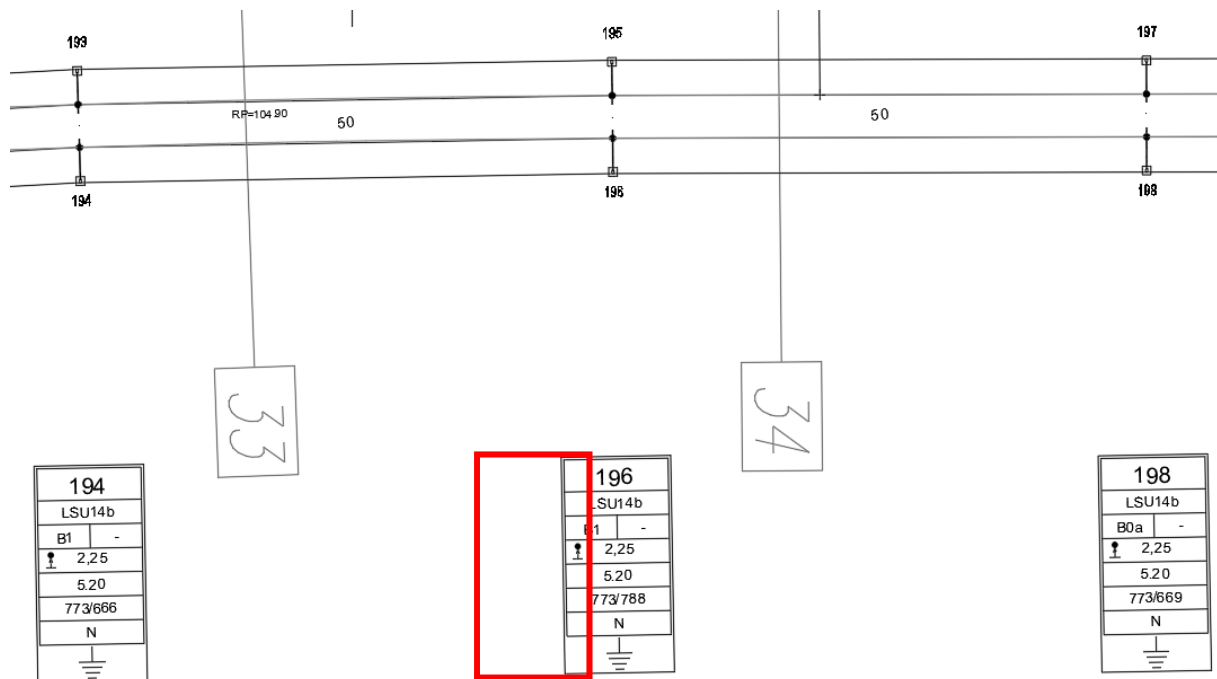
Figura 1 - Rappresentazione del palo in questione
