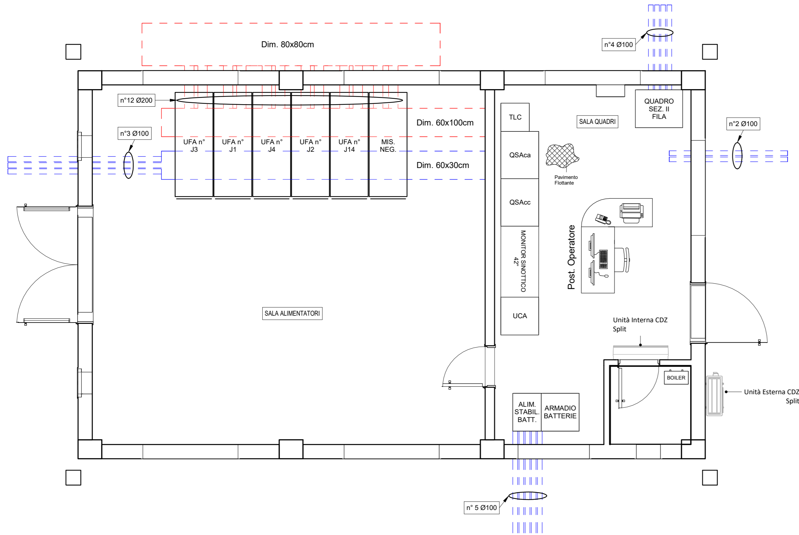
Pianta Fabbricato di cabina TE- Canalizzazioni e pozzetti
