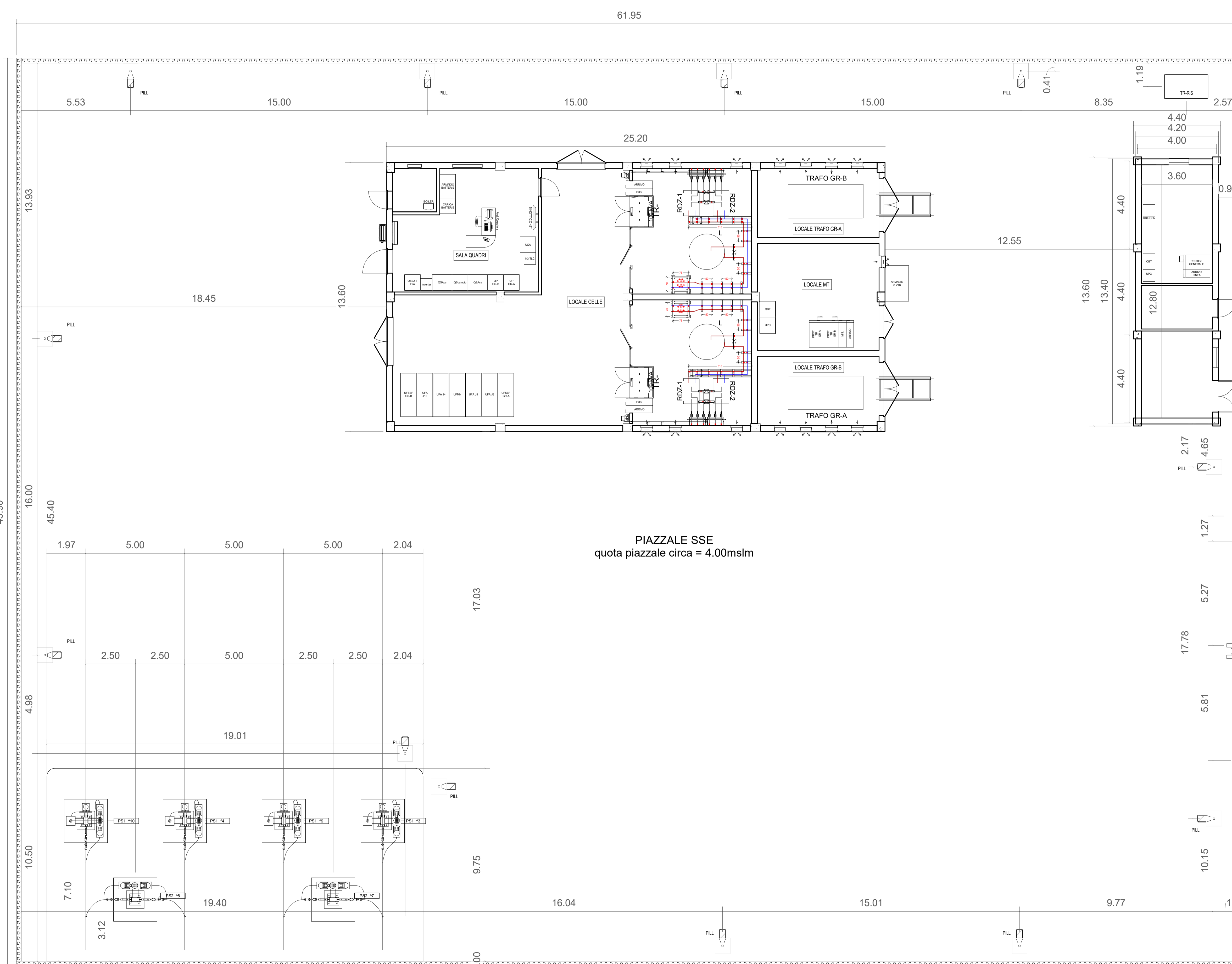
PLANIMETRIA PIAZZALE SSE - Apparecchiature 1 : 100
