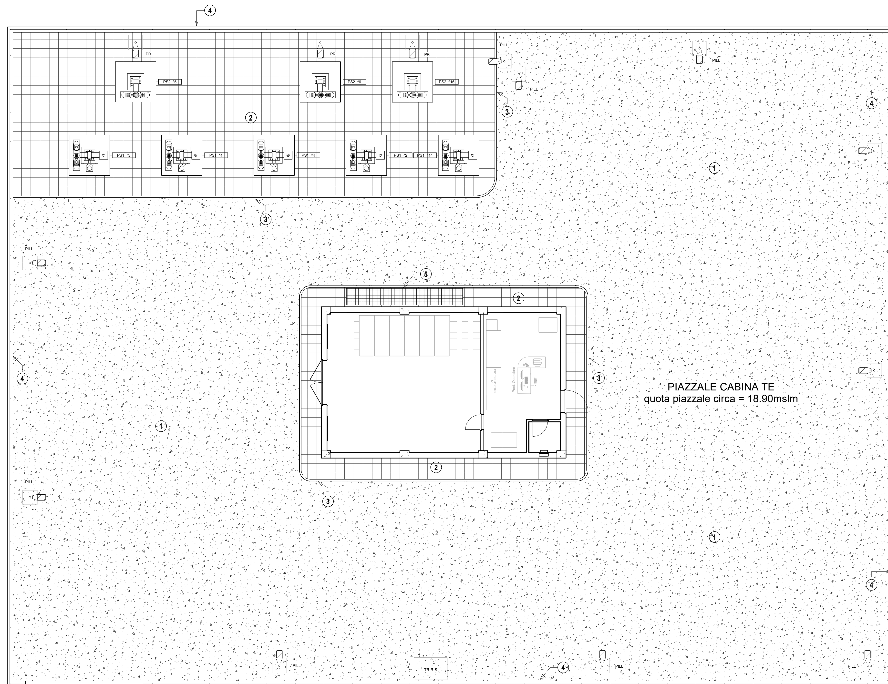
Planimetria Piazzale - Planimetria Sistemazione area e viabilità 1 : 100
